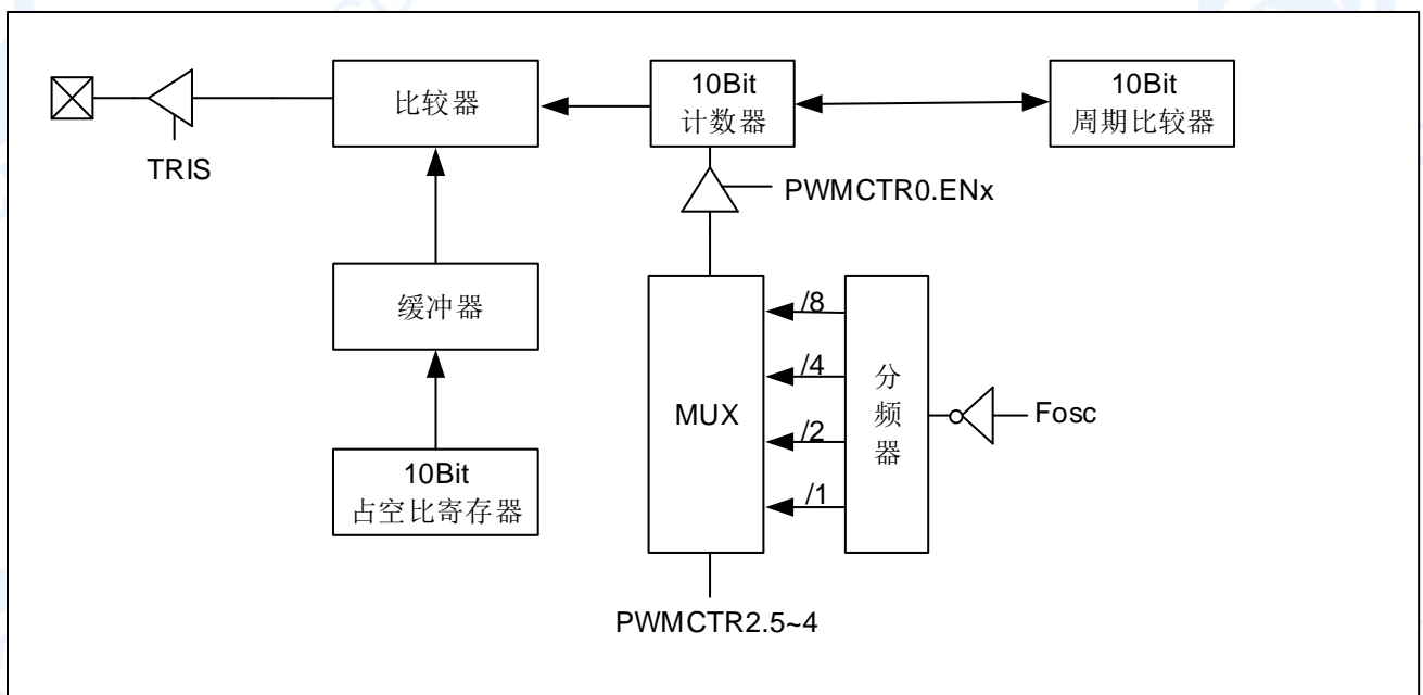
图 9-1: 普通 PWM 框图
