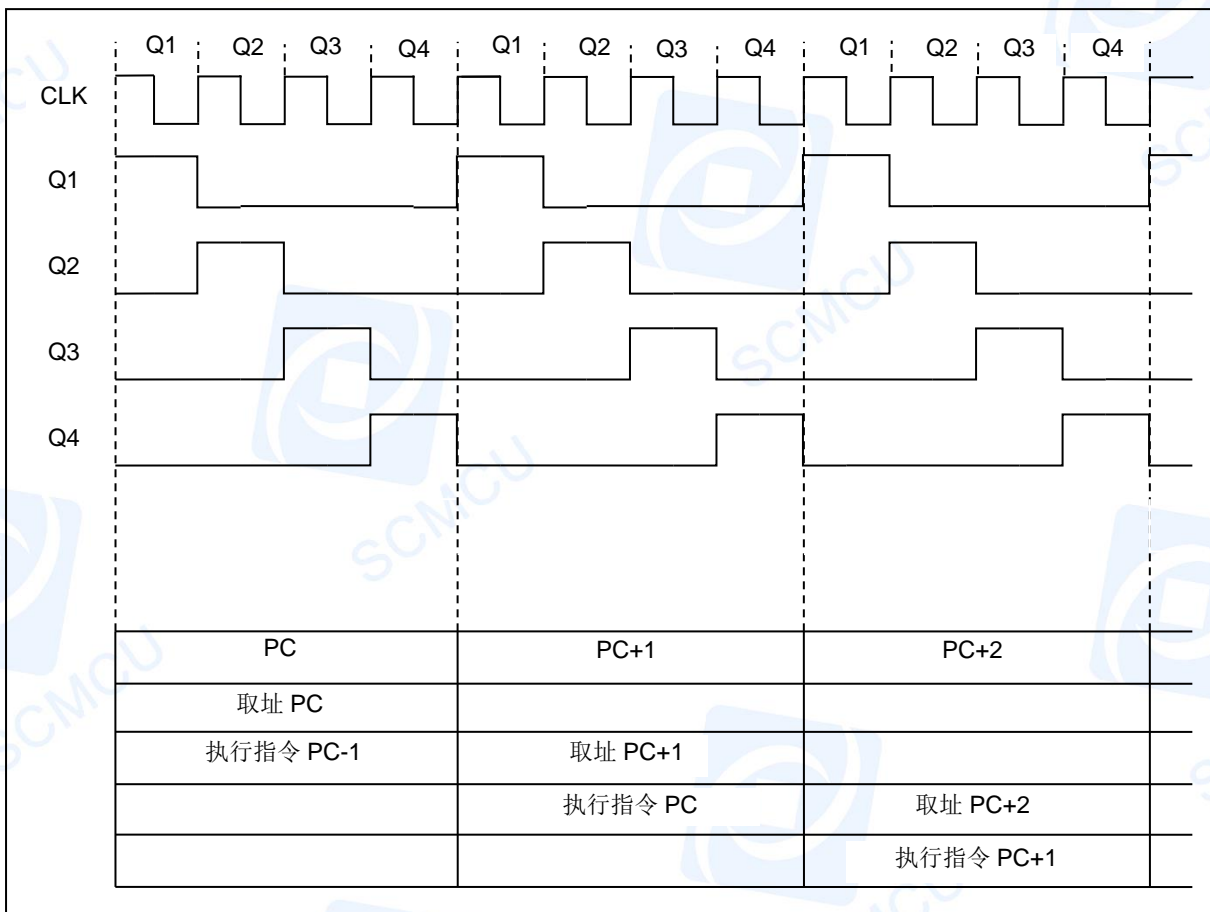
图 3-1: 时钟与指令周期时序图
