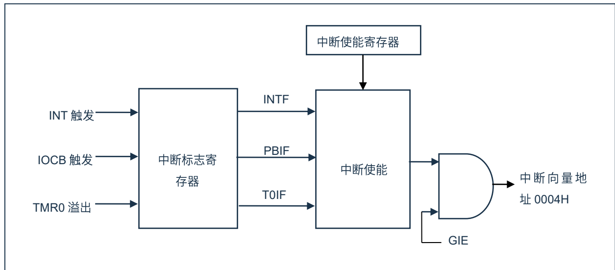
图7-1：中断系统
