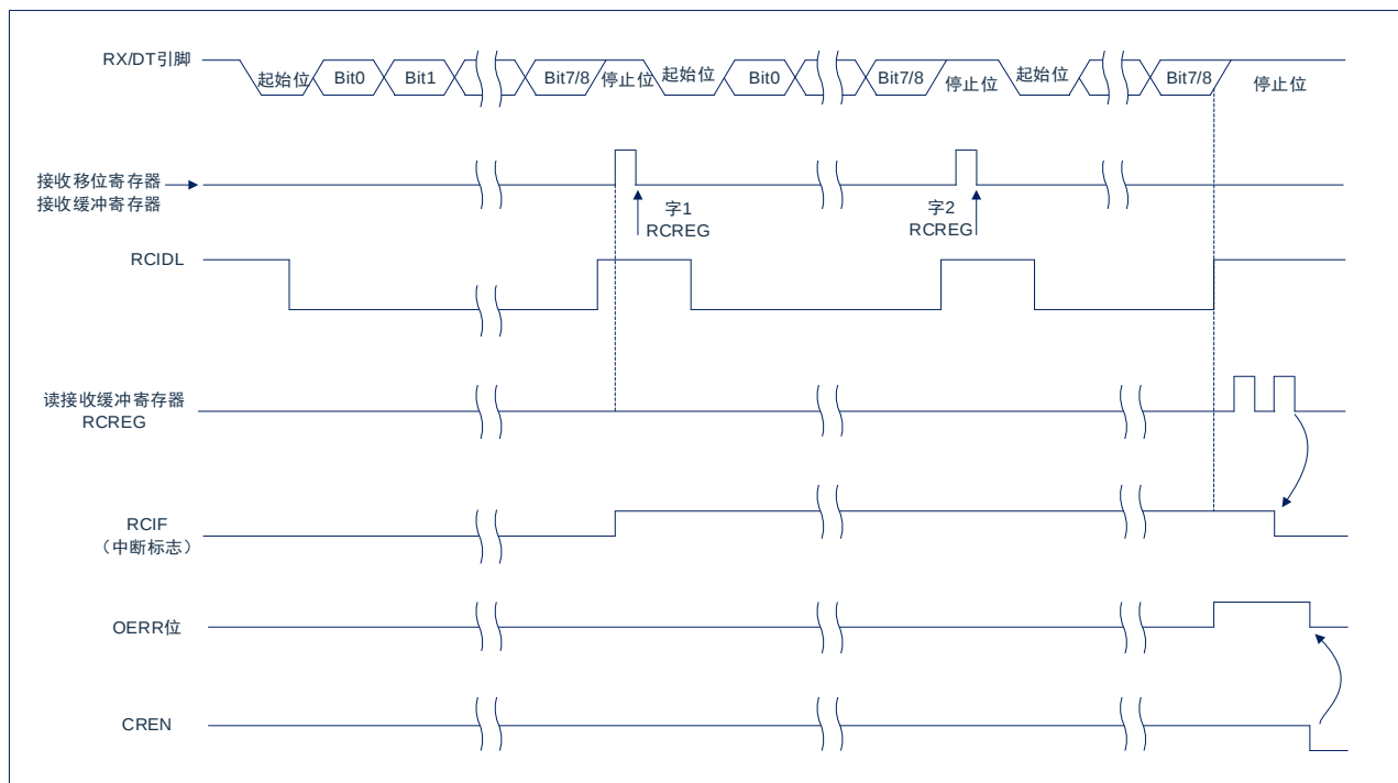
图 18-5: 异步接收
