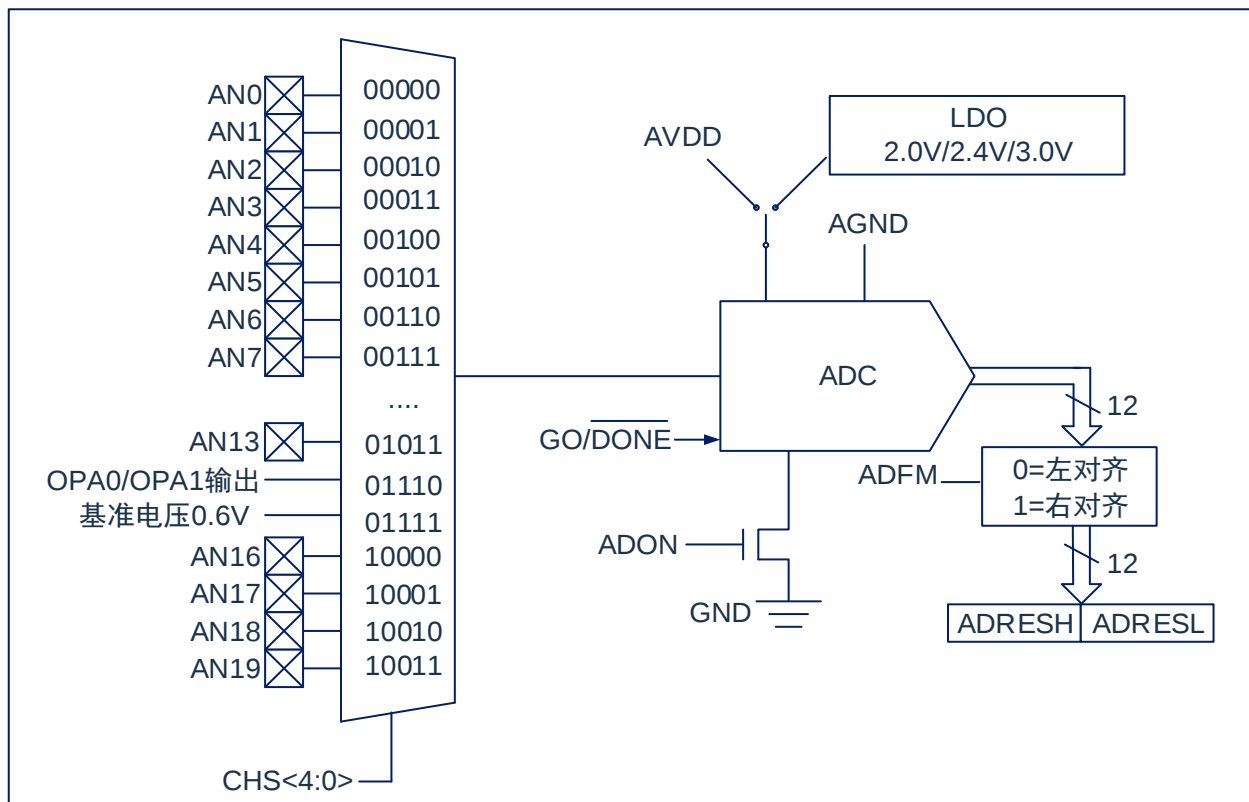
图 11-1: ADC 框图
