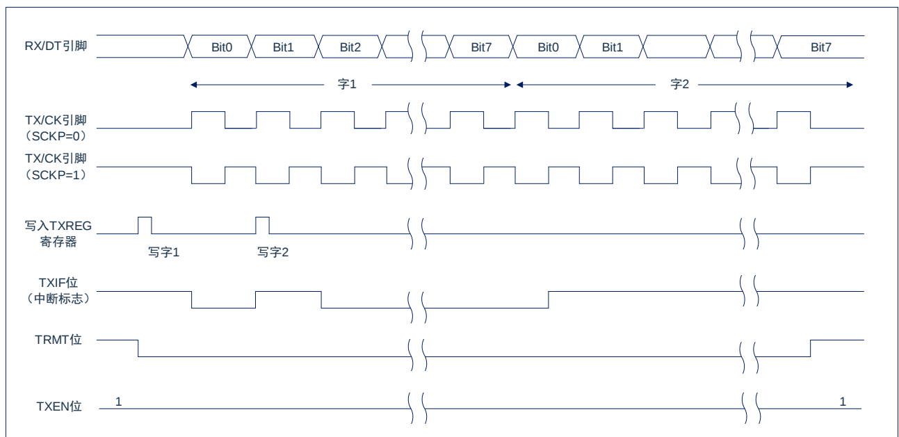
图 18-6：同步发送
