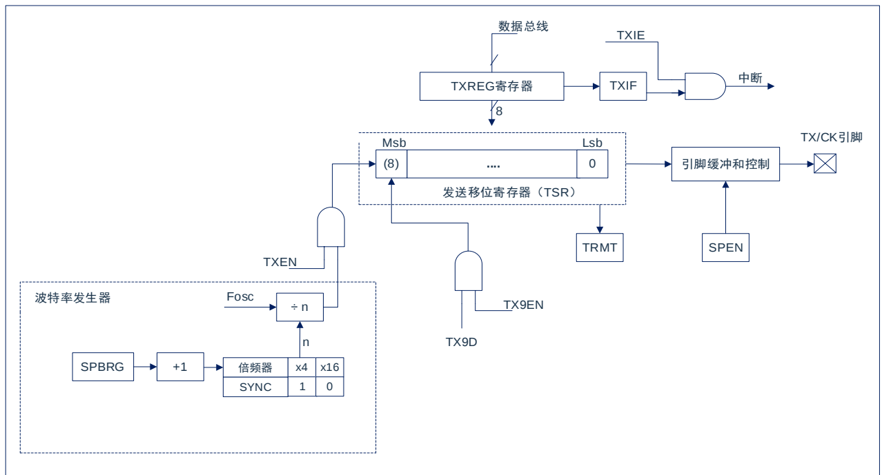
图18-1: USART发送框图
