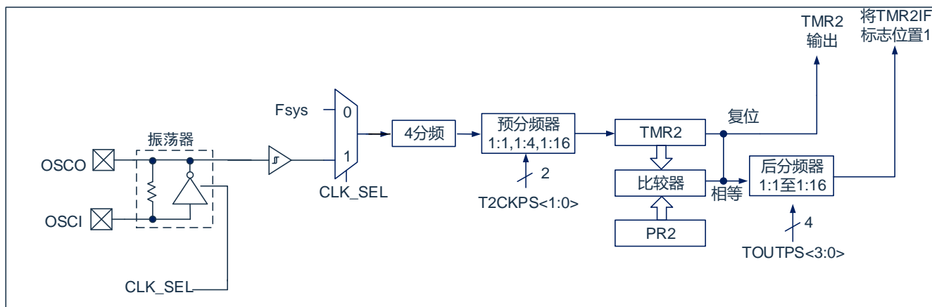
图 9-1: TIMER2 框图
