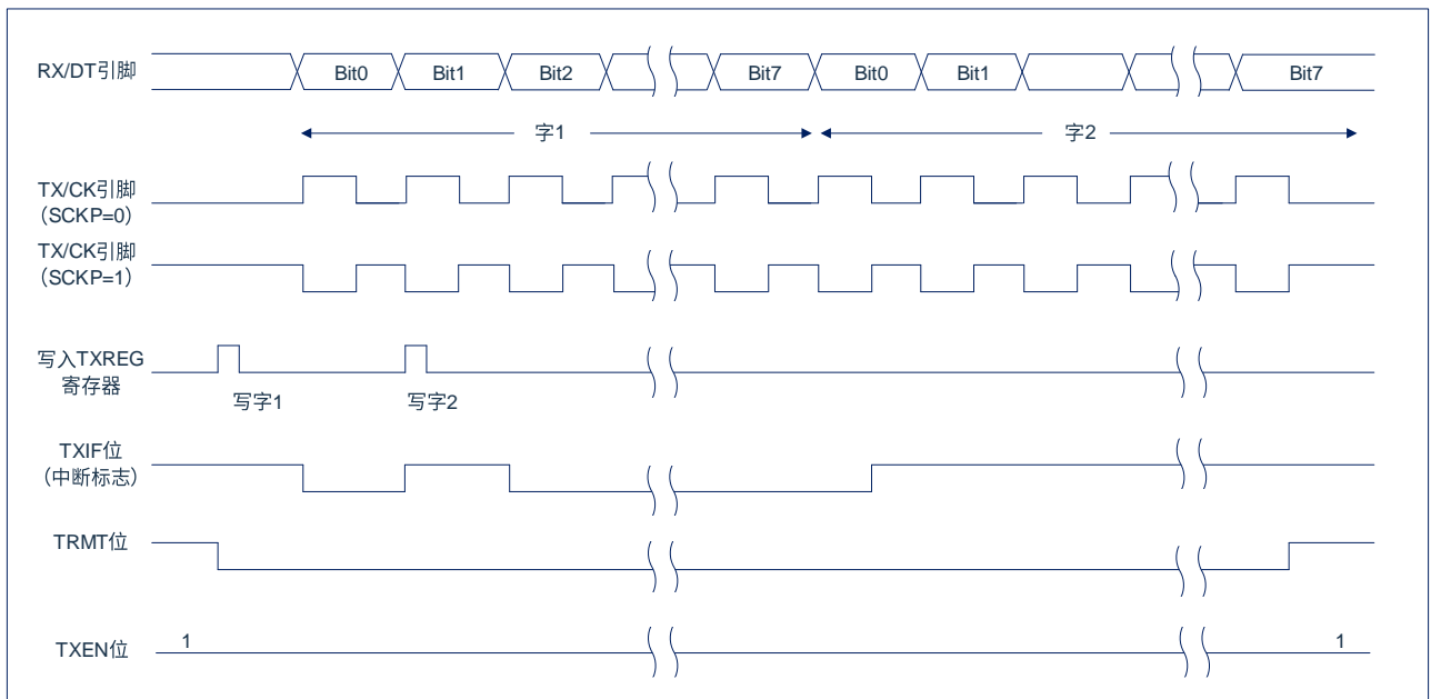
图 16-6: 同步发送
