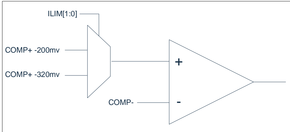
图 14-1: COMP 框图
