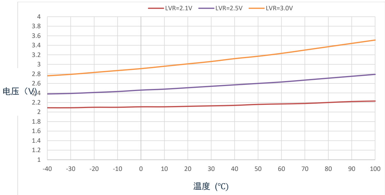
LVR 温度特性曲线
