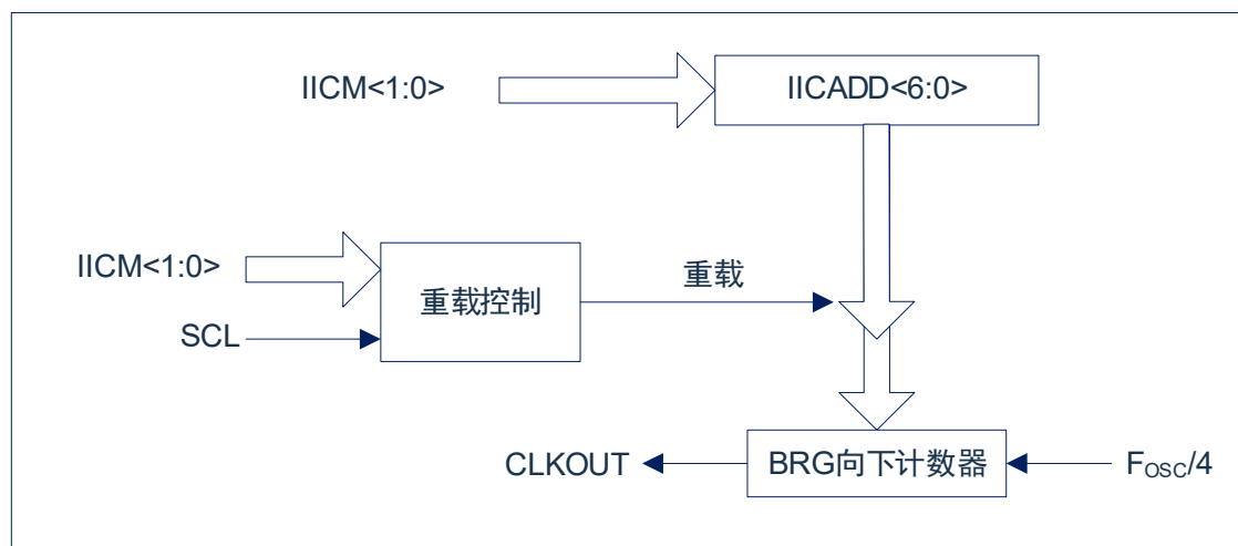
图18-3：波特率发生器框图
