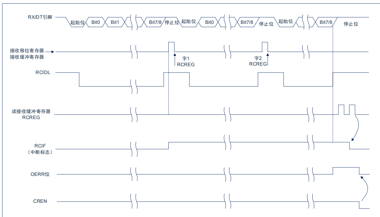
图 16-5: 异步接收
