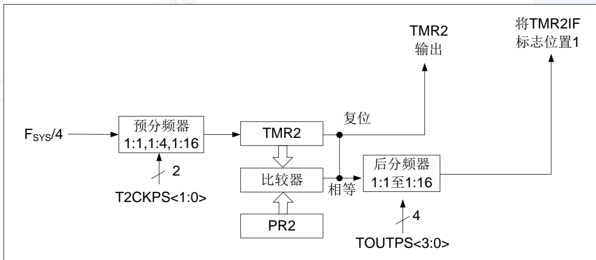
图 9-1: TIMER2 框图
