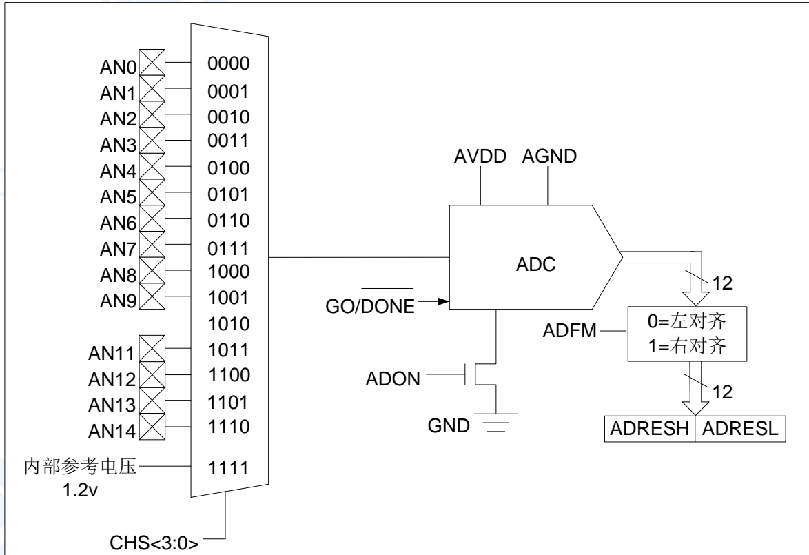
图 10-1: ADC 框图
