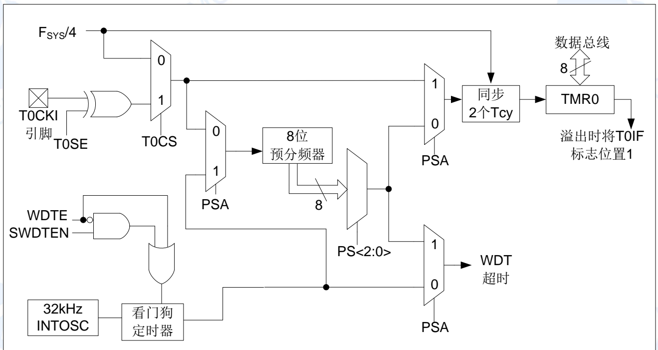
图 8-1: TIMER0/WDT 结构图
