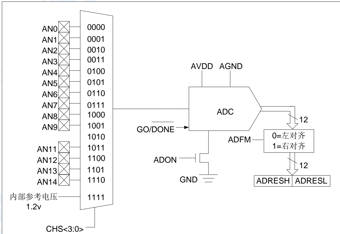
图 10-1: ADC 框图
