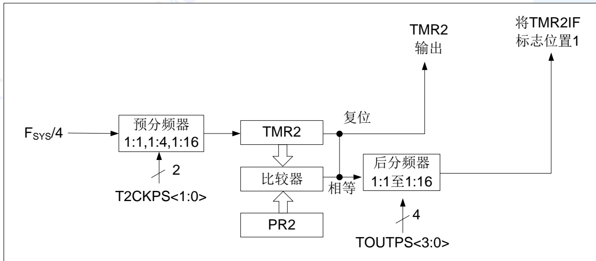
图 9-1: TIMER2 框图
