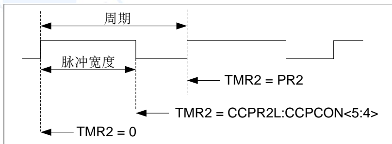
图10-3: PWM2输出
