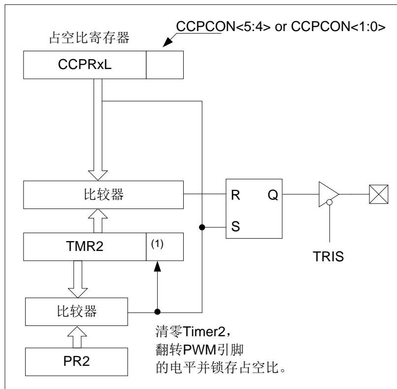
图 10-1: PWM 简化框图
