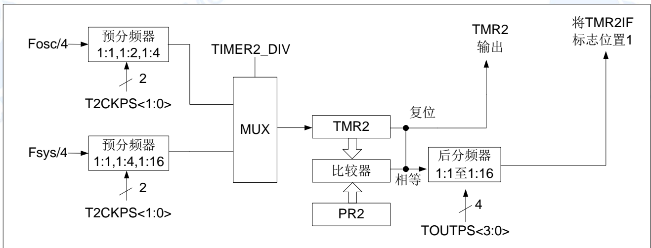
图 9-1: TIMER2 框图
