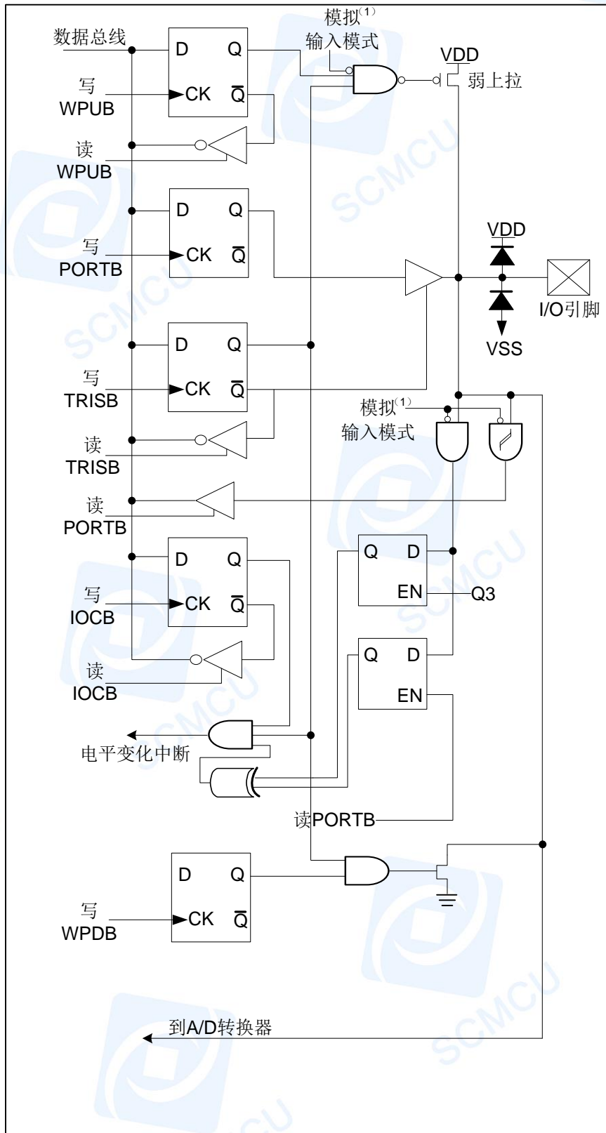
图 6-2: I/O 口结构图
