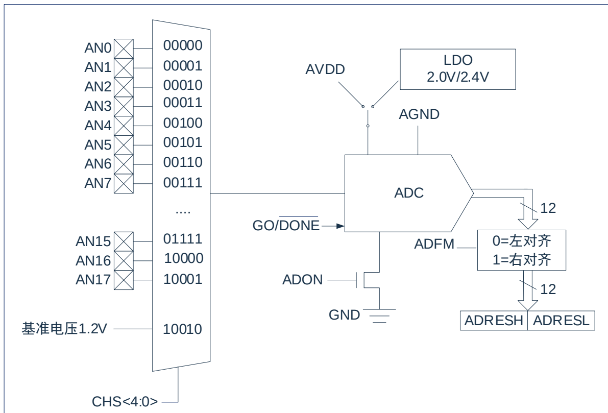
图 11-1：ADC 框图
