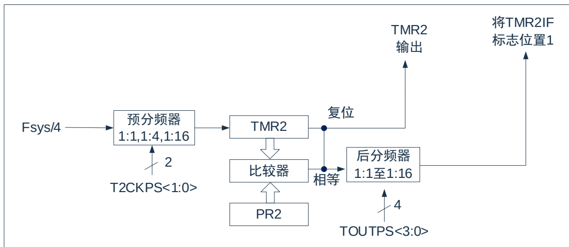
图 10-1: TIMER2 框图
