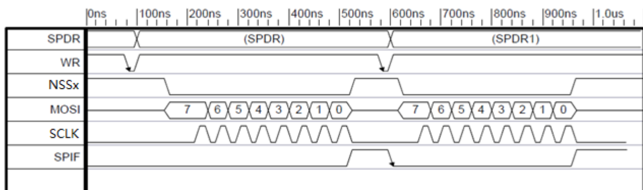
图 17-3: 自动从机选择线使用
