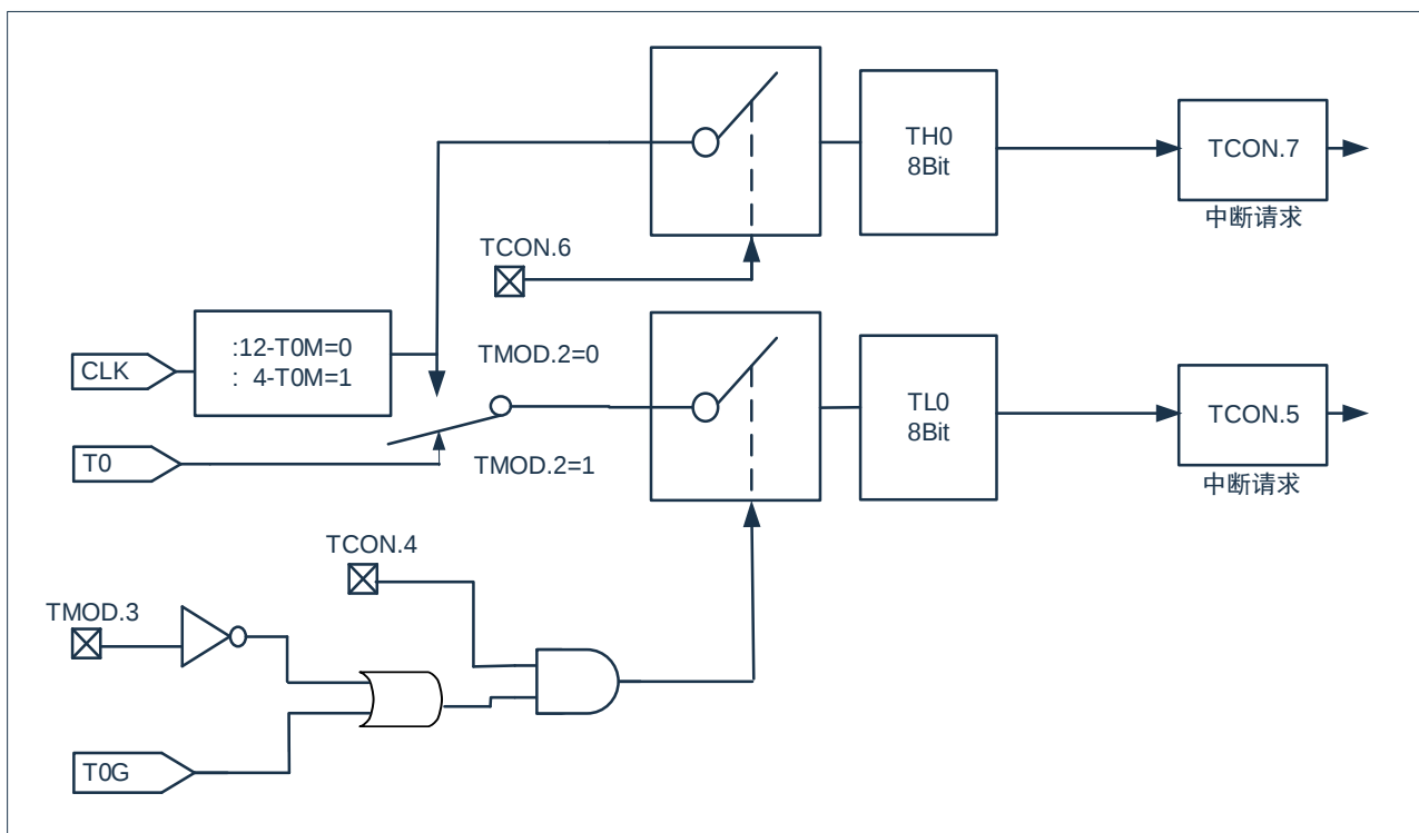
图 8-4: Timer0, 模式 3: 两个 8-位定时/计数器
