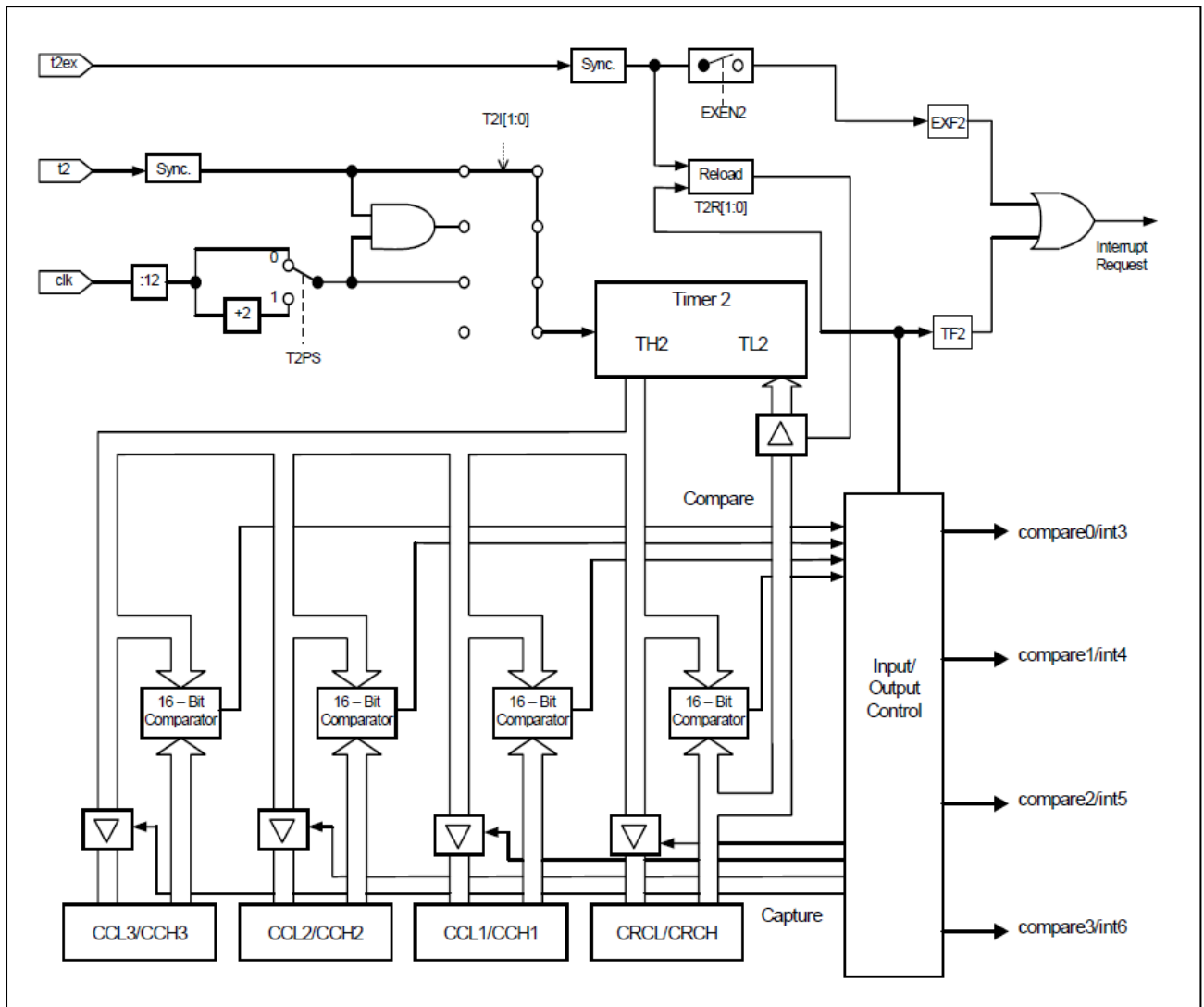
图 9-1: 比较/捕获模块
