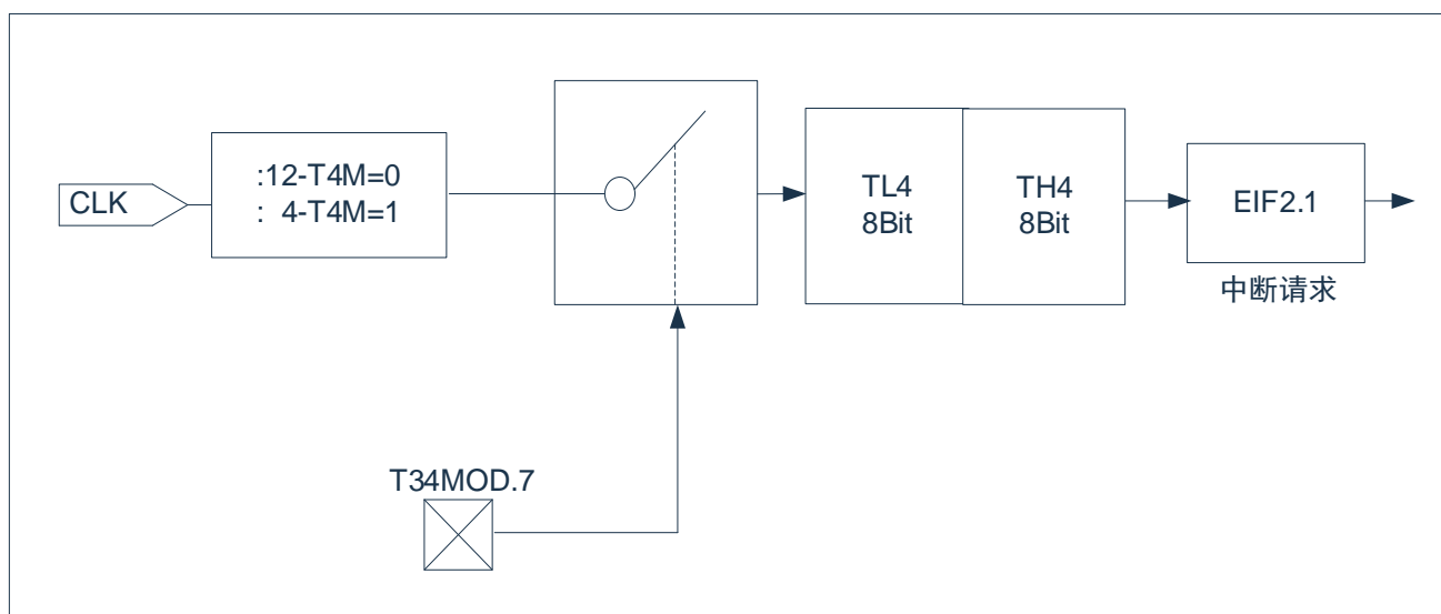
图 10-6: Timer4, 模式 1: 16-位定时/计数器
