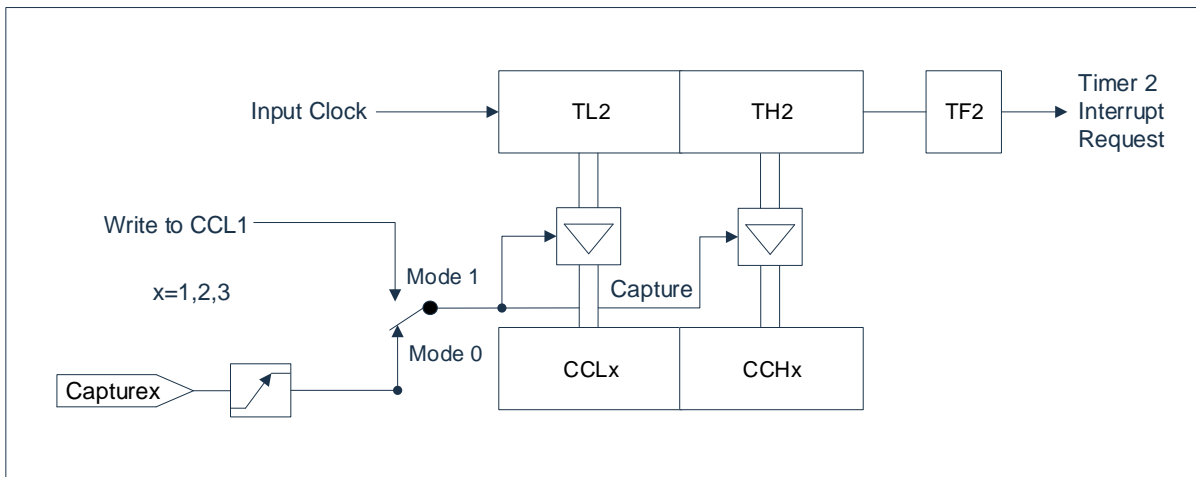
图 9-7: Timer2 捕获模式对应 CCLx 与 CCHx 寄存器
