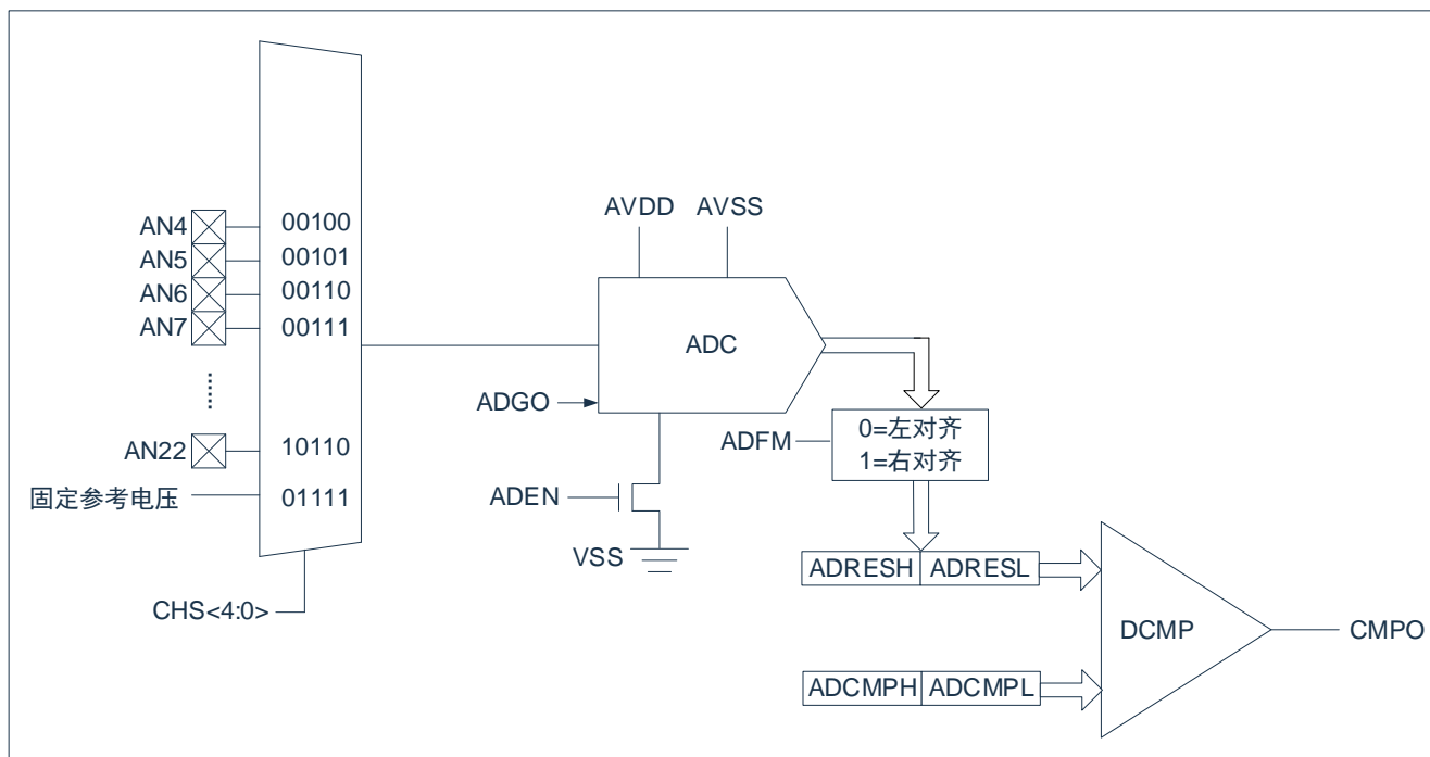
图 12-1: ADC 框图
