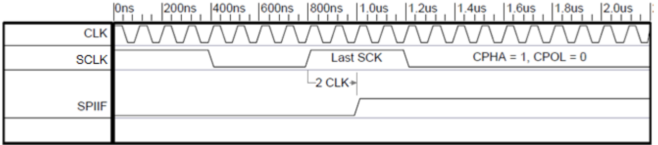
图 17-12: 中断产生
