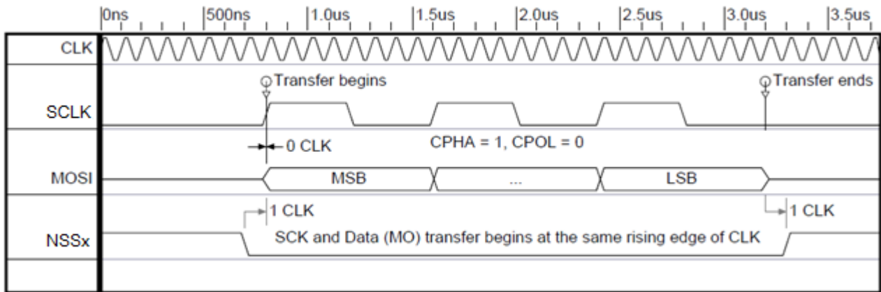
图 17-10: 主模式时序图
