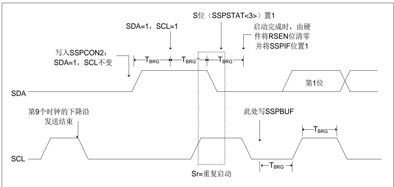
图 11-13: 重复启动条件时序波形
