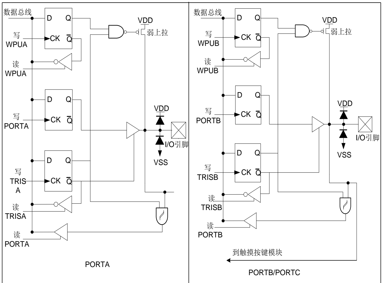
图 6-1: I/O 结构图
