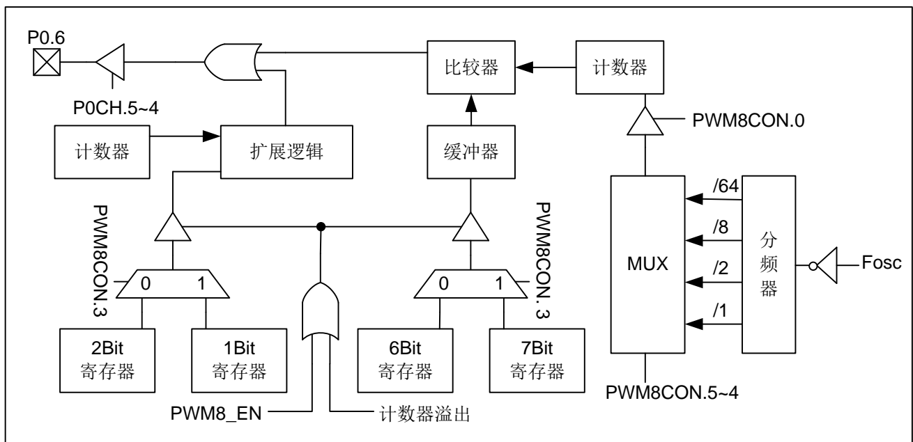
图 16-1：8 位 PWM 框图
