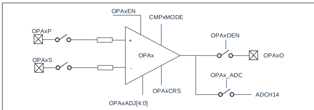
图 13-1: OP Ax 框图
