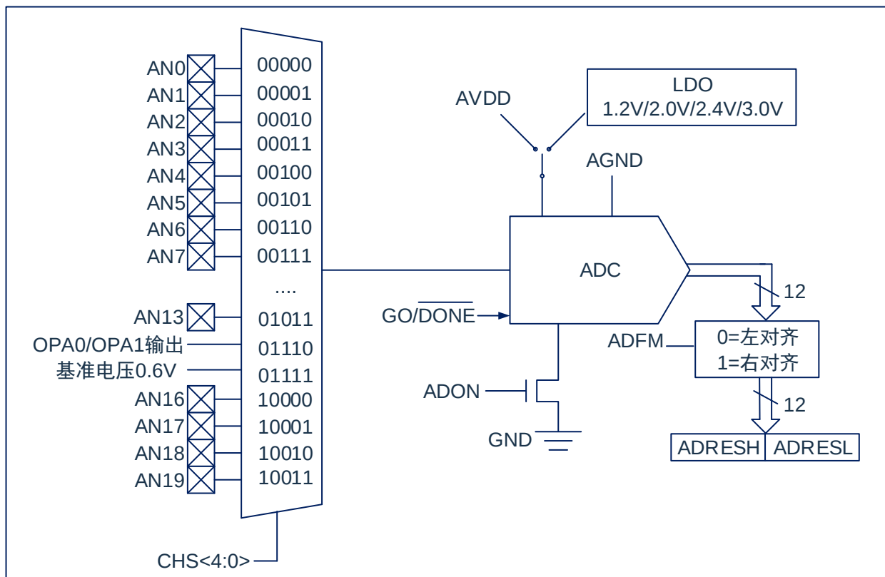
图 10-1: ADC 框图
