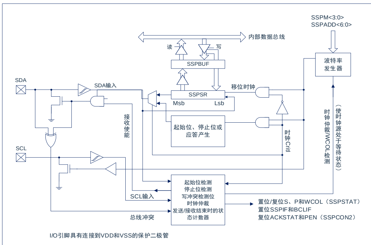
图15-6: MSSP框图 (I 2 C™主控模式)
