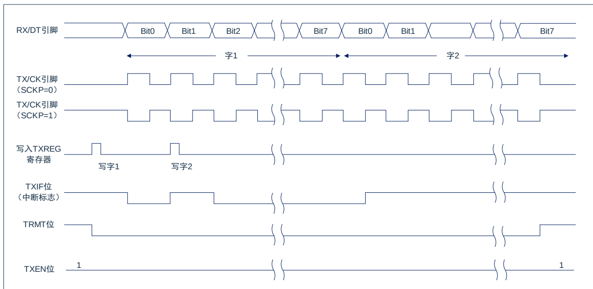
图 14-6：同步发送
