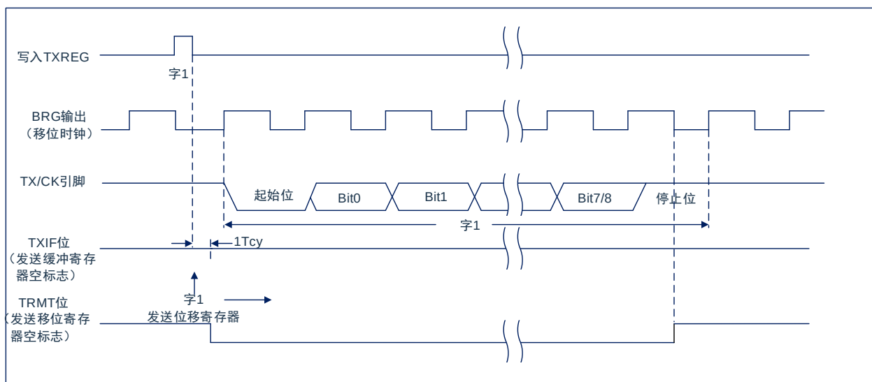
图 14-3：异步发送
