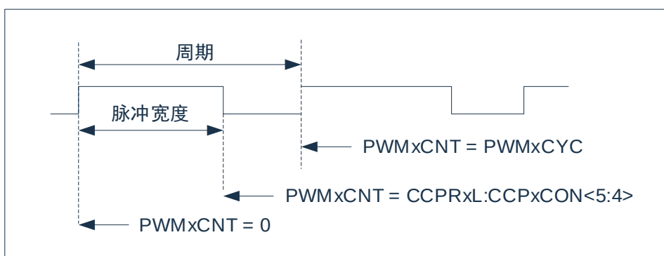
图13-4: CCPPWM输出
