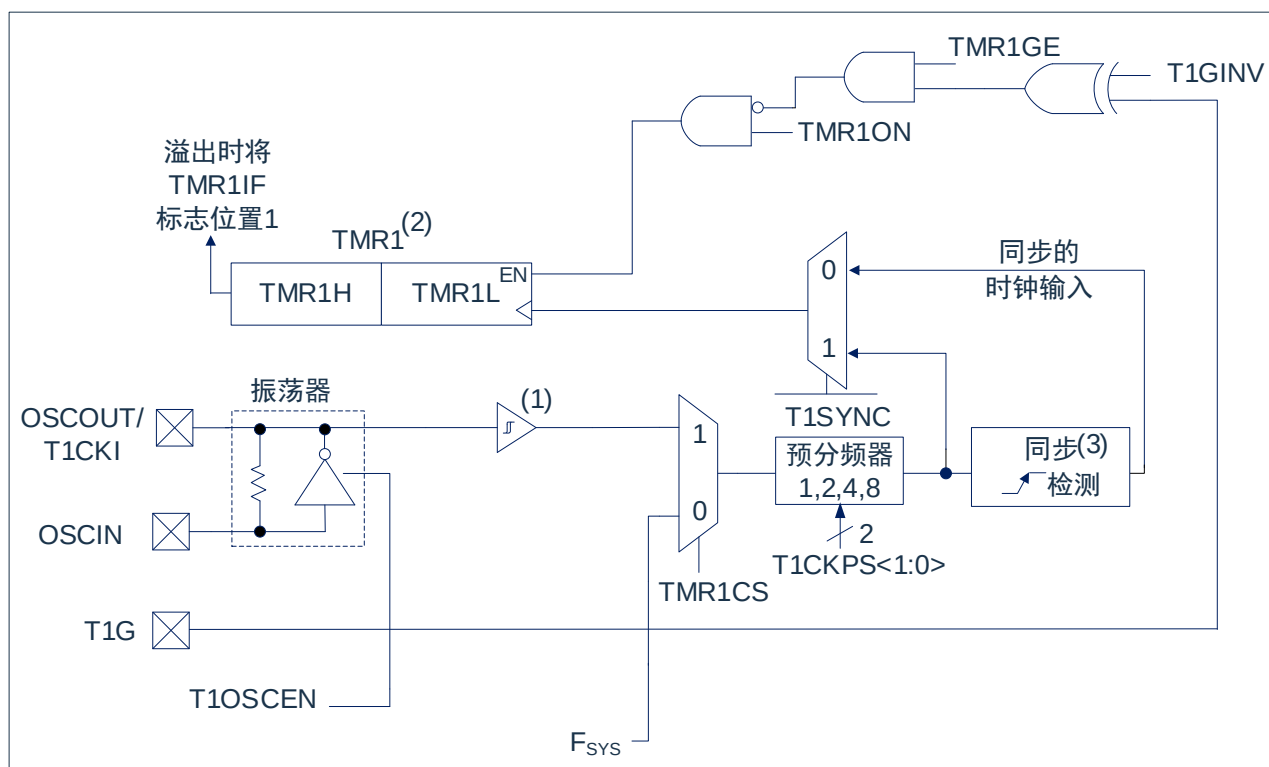
图9-1: TIMER1结构图
