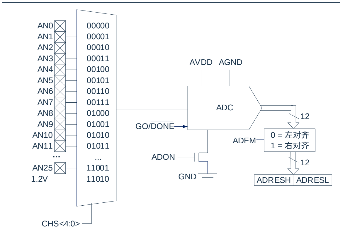
图 11-1: ADC 框图
