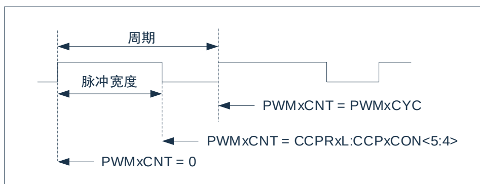
图13-4: CCPPWM输出
