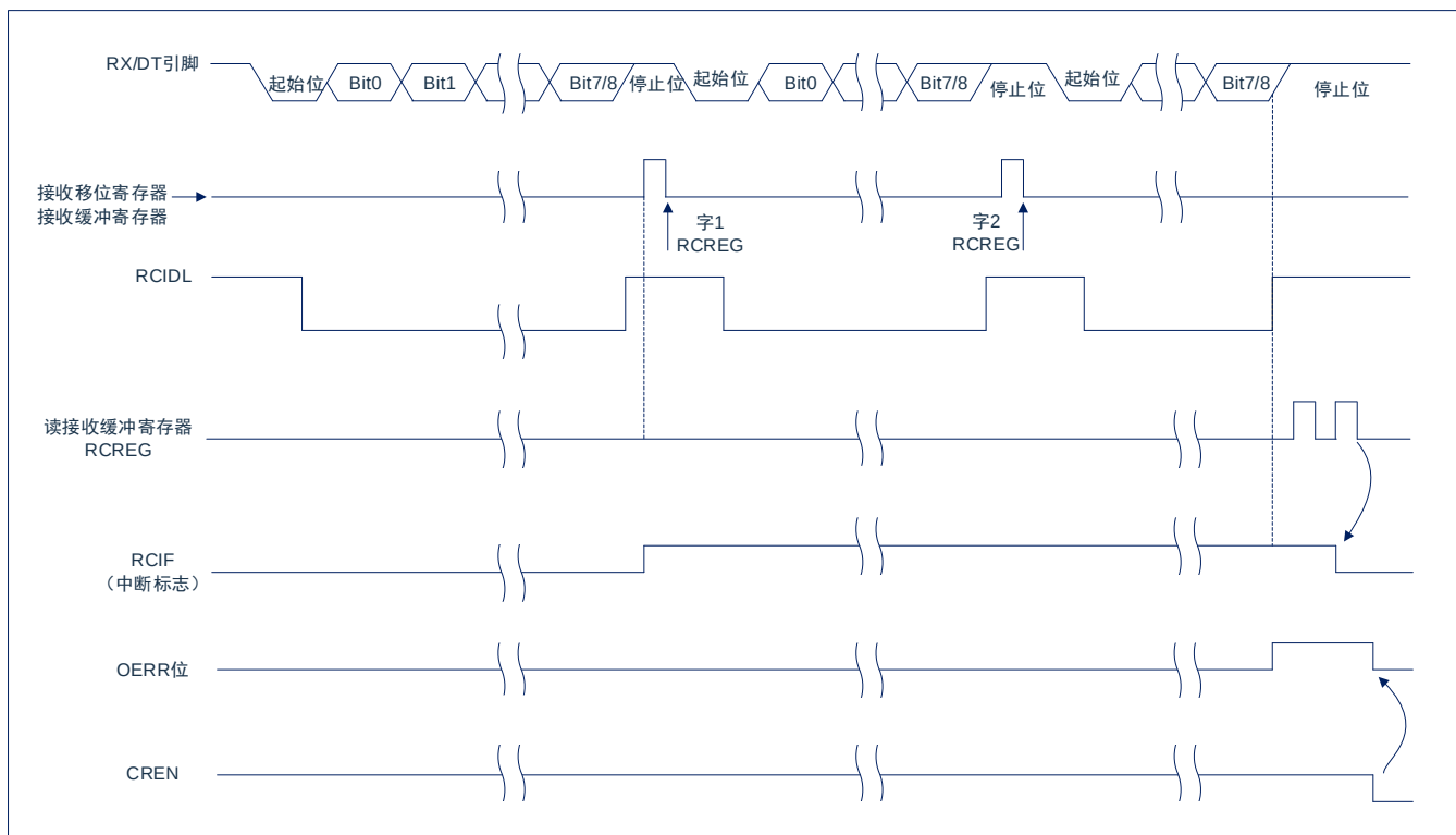
图 14-5: 异步接收
