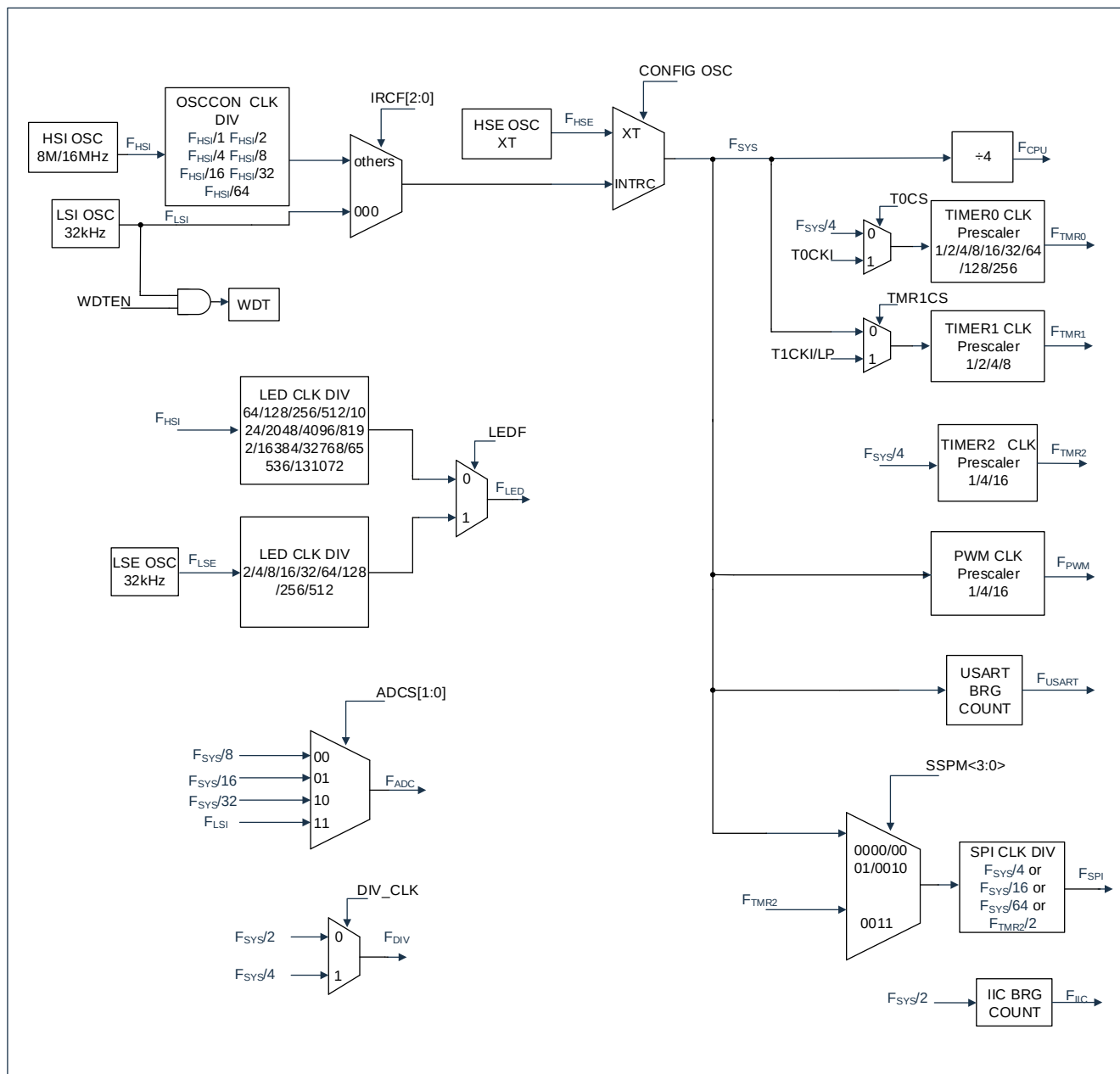
图 3-2: 时钟框图
