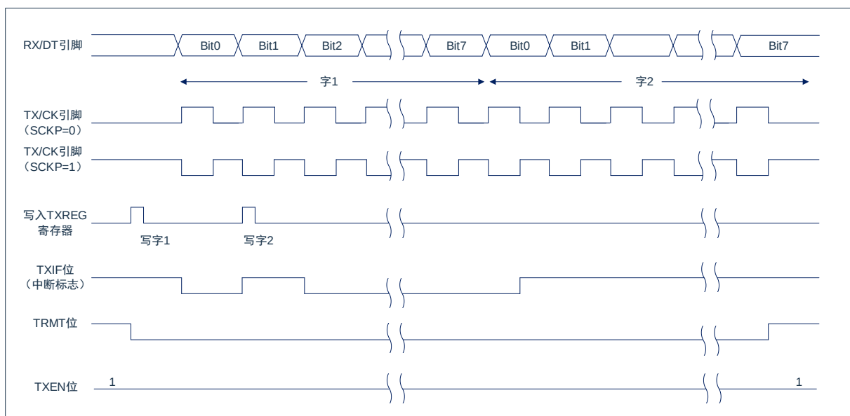
图 14-6：同步发送
