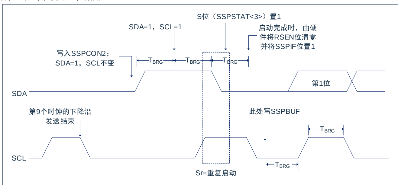
图15-13：重复启动条件时序波形
