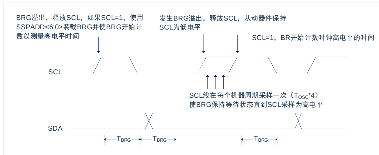
图 15-16：主控发送模式下的时钟仲裁时序
