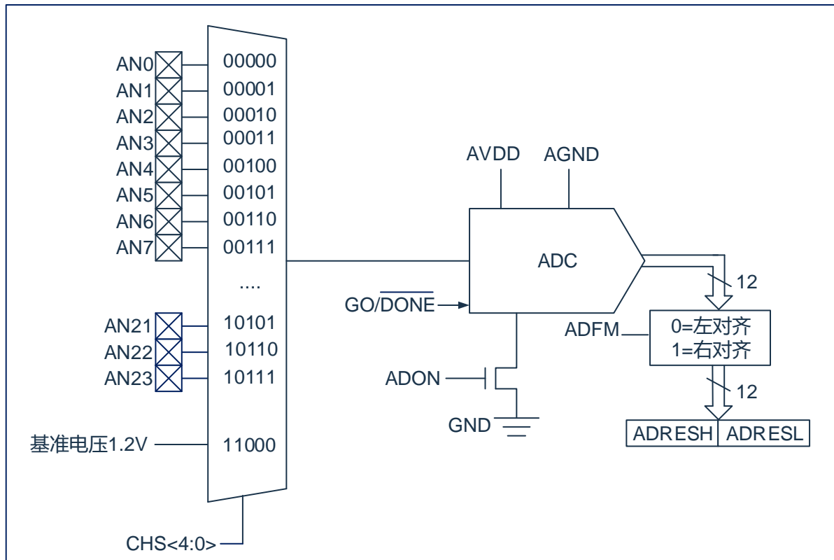
图 11-1: ADC 框图
