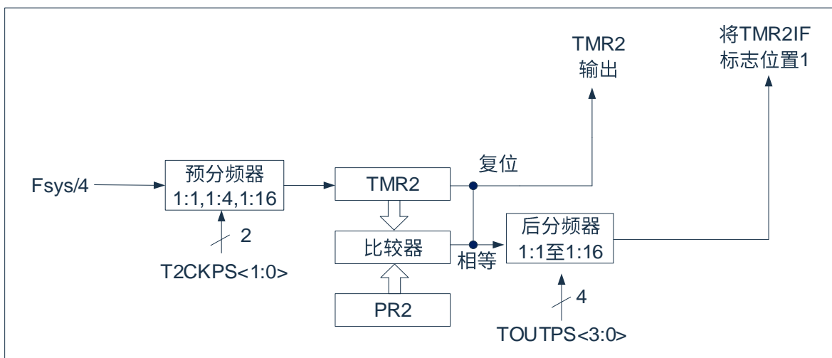
图 9-1: TIMER2 框图
