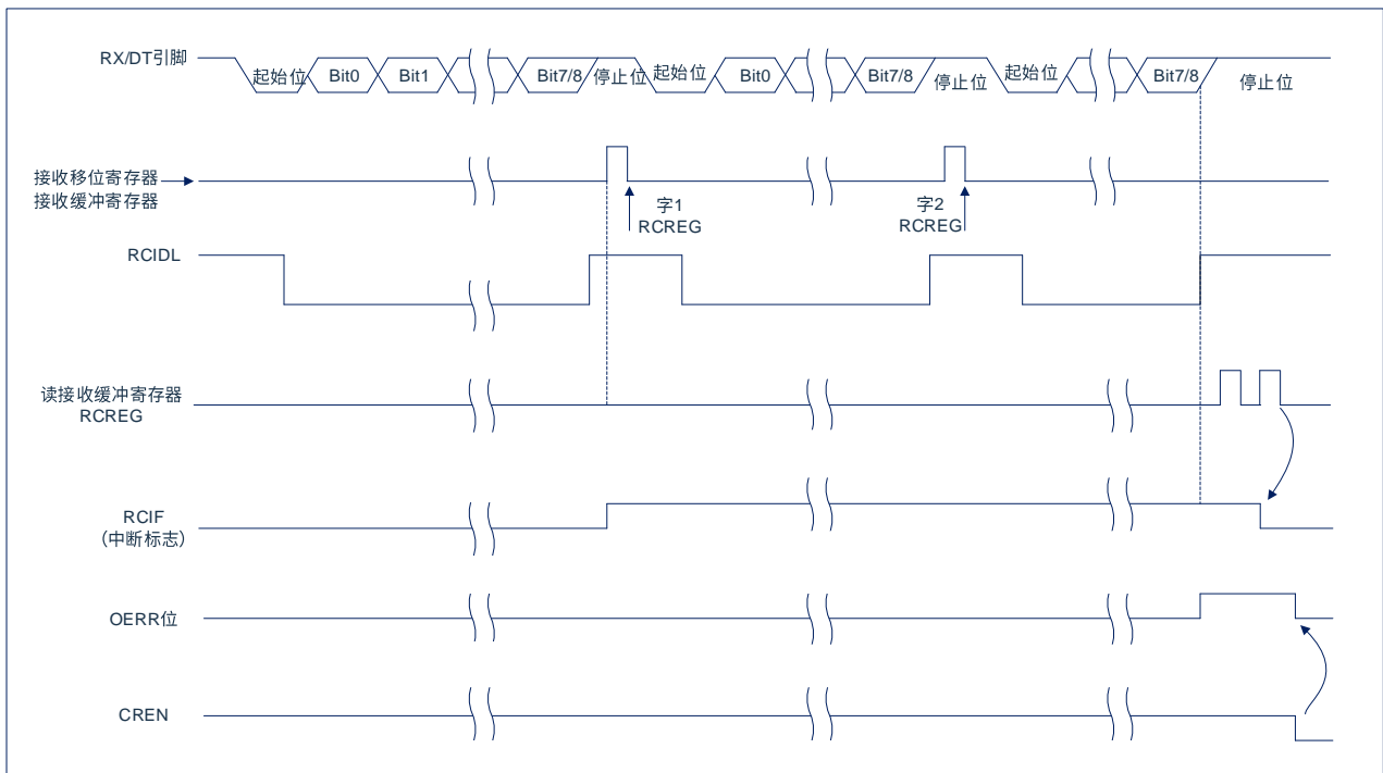
图 14-5: 异步接收
