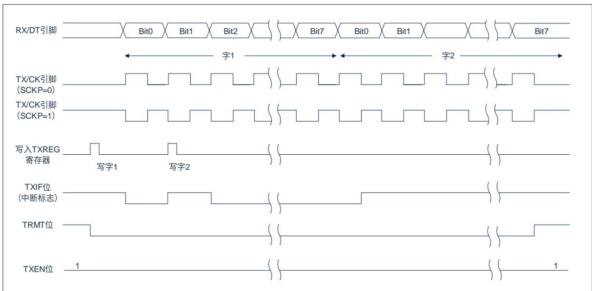
图 14-6: 同步发送
