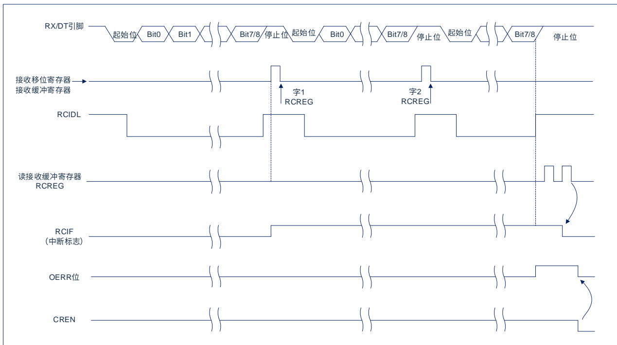
图 14-5: 异步接收
