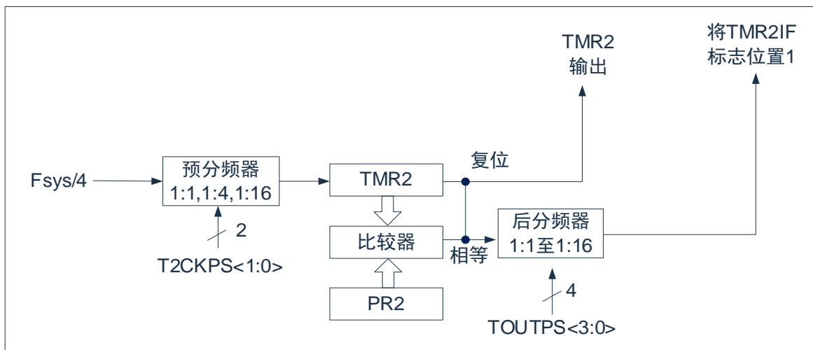
图 9-1: TIMER2 框图
