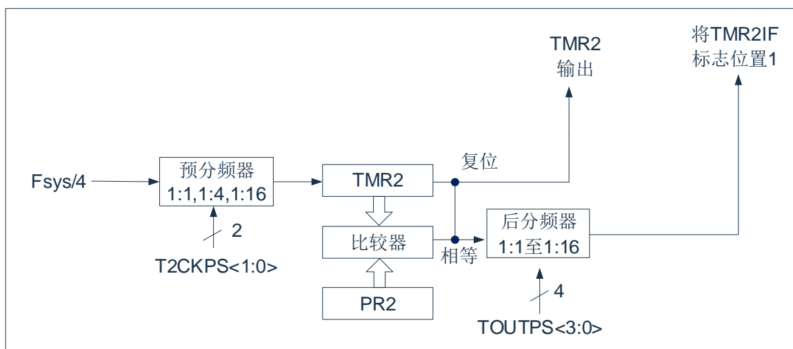
图 10-1 : TIMER2 框图
