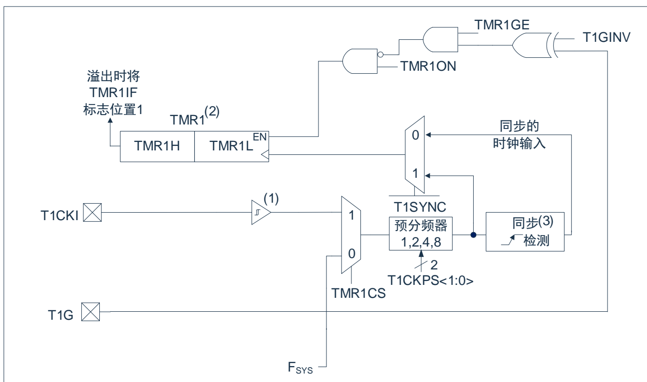
图9-1：TIMER1结构图
