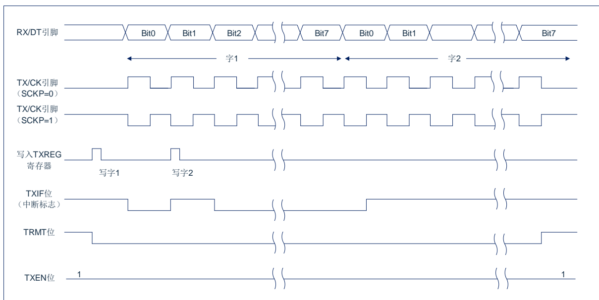
图 14-6：同步发送
