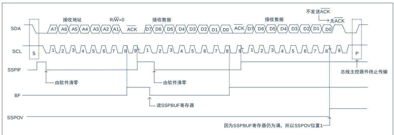
图 15-17: I²C™ 从动模式接收时序（7 位地址）
