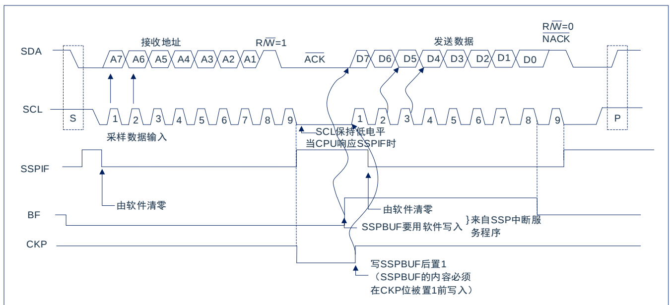
图 15-18: I²C™ 从动模式发送时序（7 位地址）
