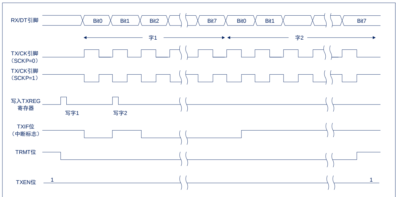
图 15-6：同步发送
