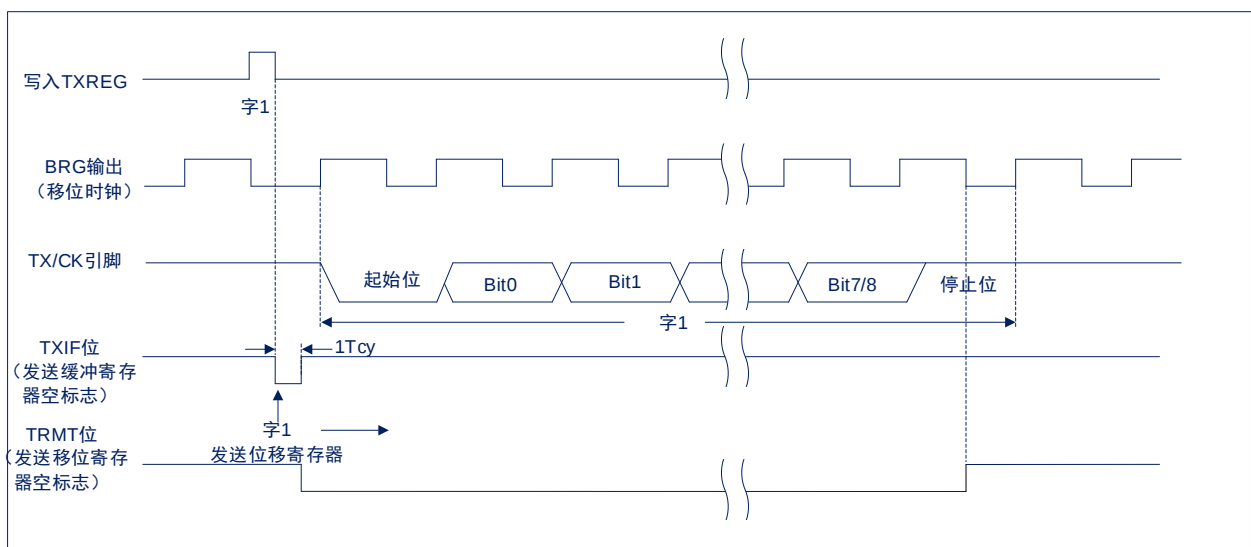
图 15-3: 异步发送
