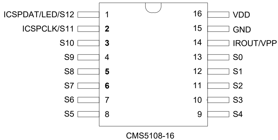
CMS5108-16 引脚说明:
