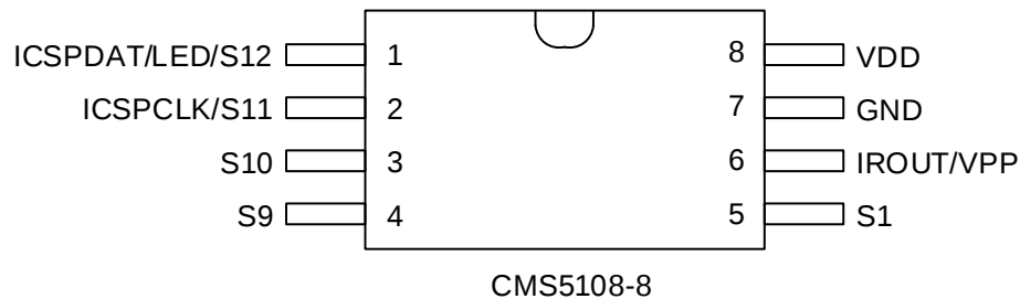
CMS5108-8 引脚说明:
