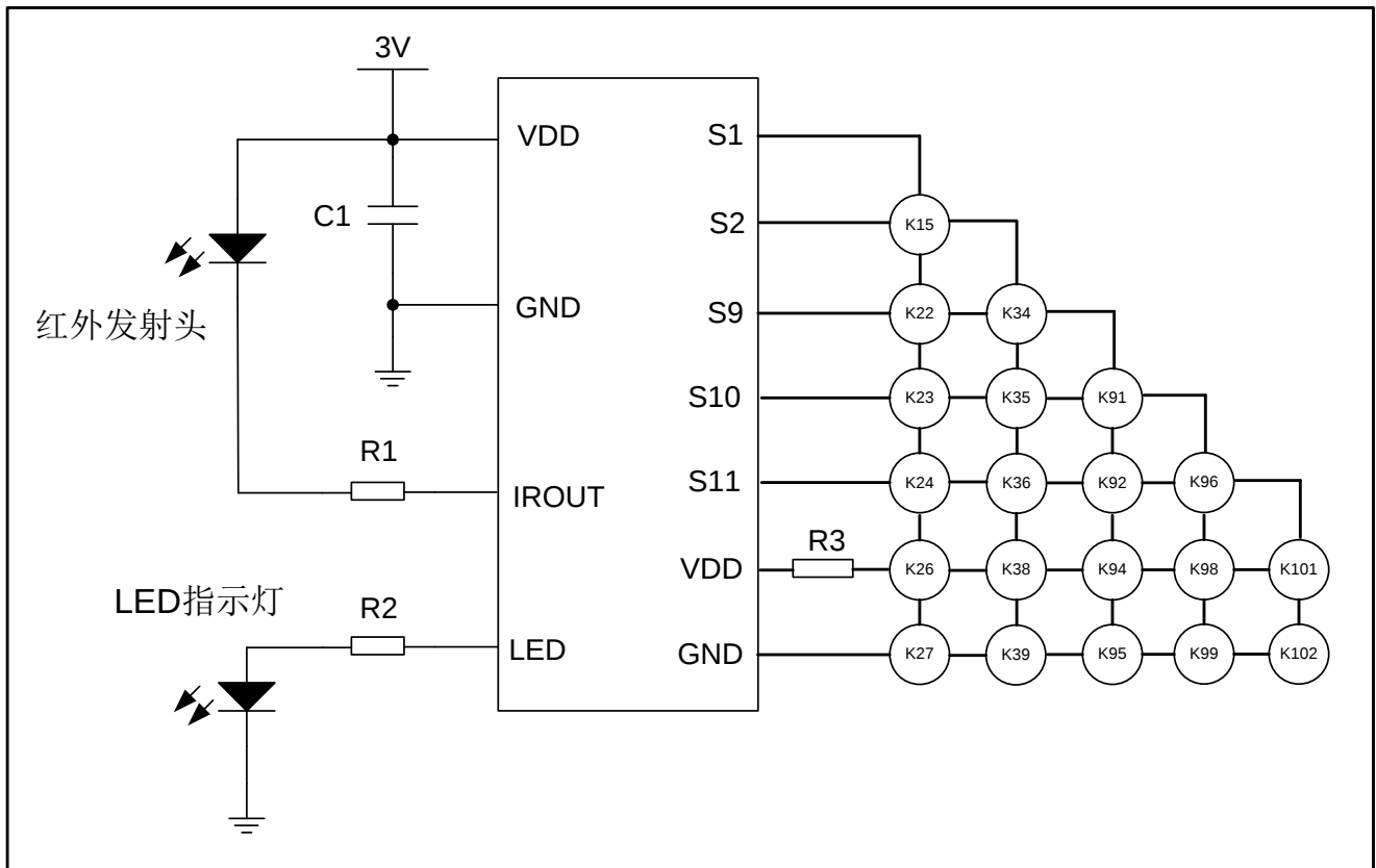
图 2-4：9PIN 带 LED 输出电路图
