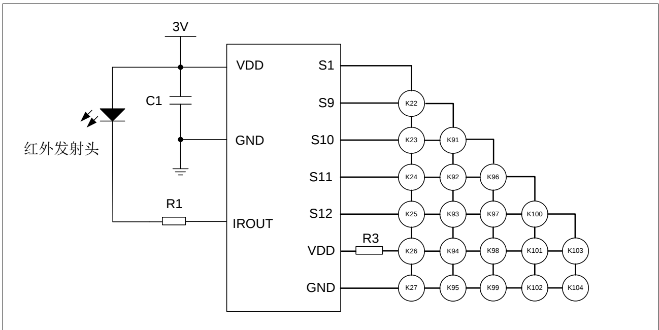
图 2-1: 8PIN 不带 LED 输出电路图
