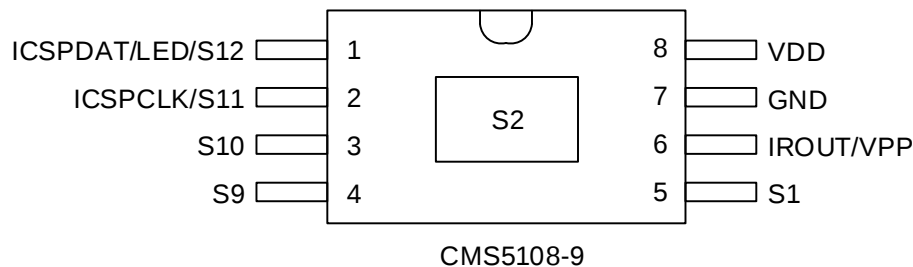
CMS5108-9 引脚说明:
