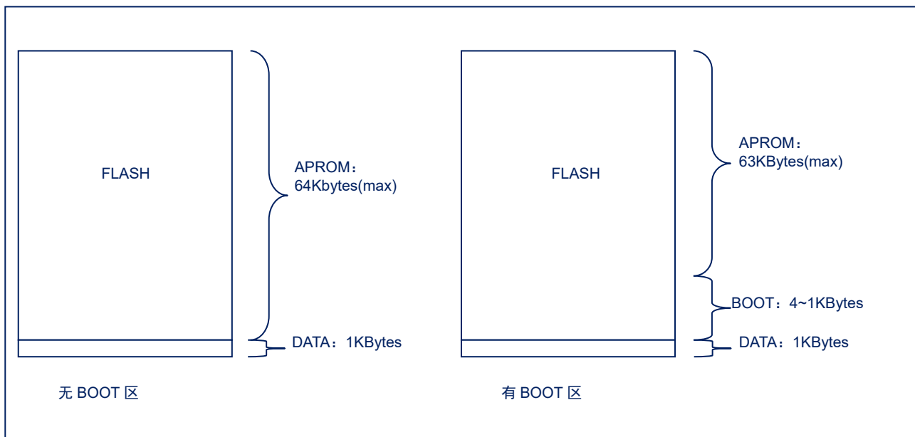
图 25-1: 存储器结构图
