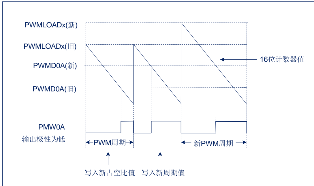
图 15-1: PWM 时序图
