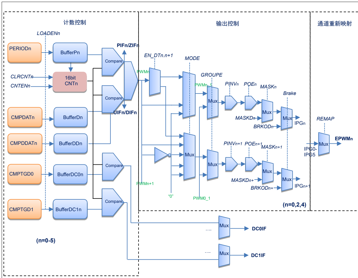
图 16-1: IPG n 的信号为 EPWM n 重映射前的信号。
