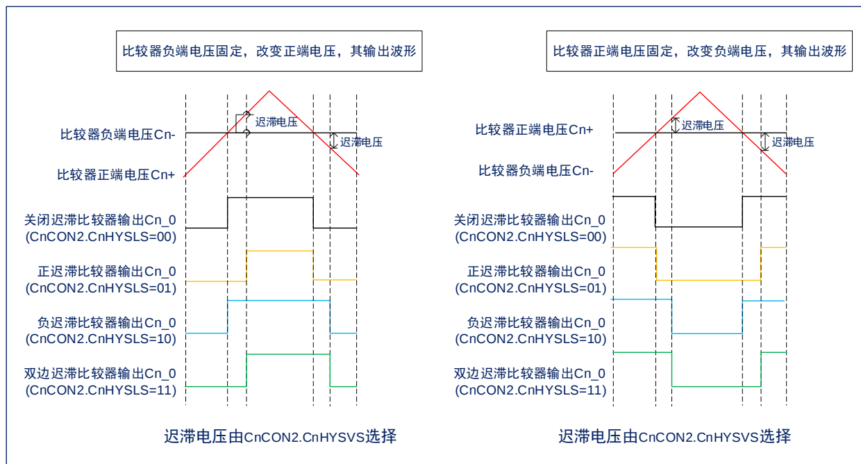
图 23-2：比较器迟滞功能结构框图
