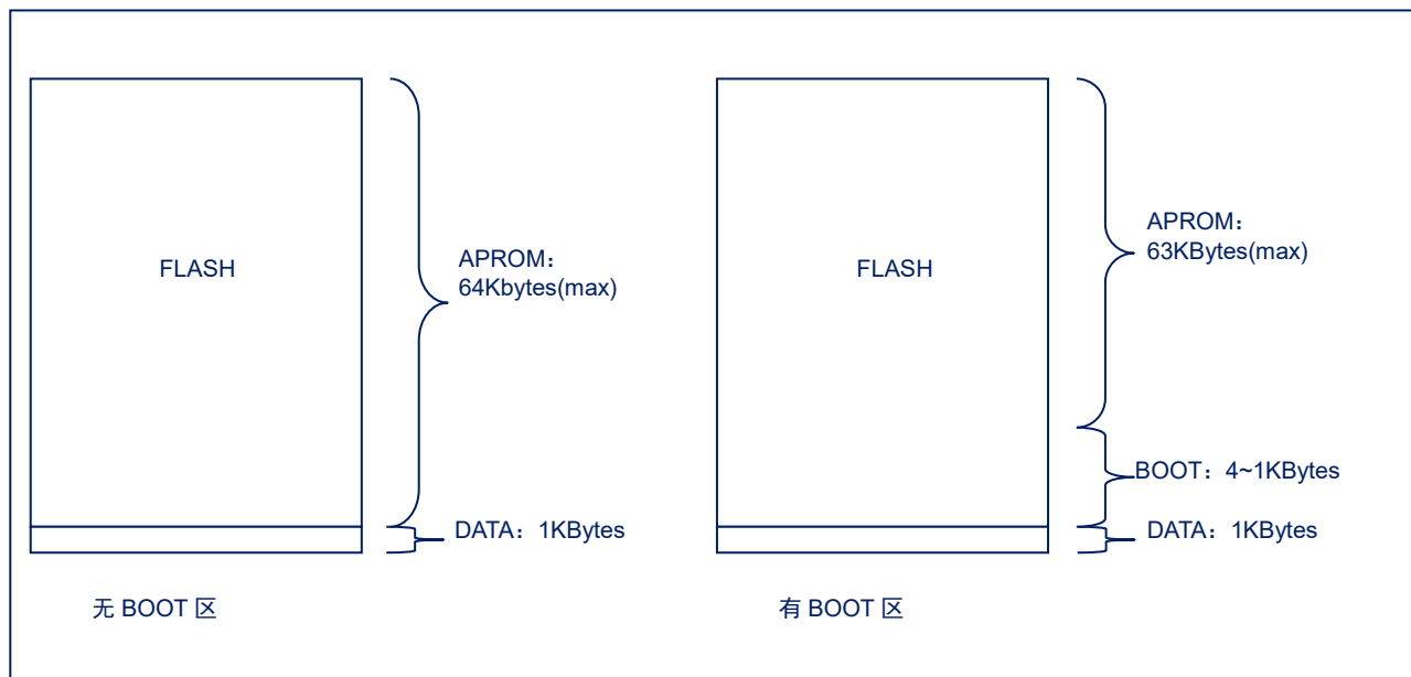
图 25-1：存储结构图
