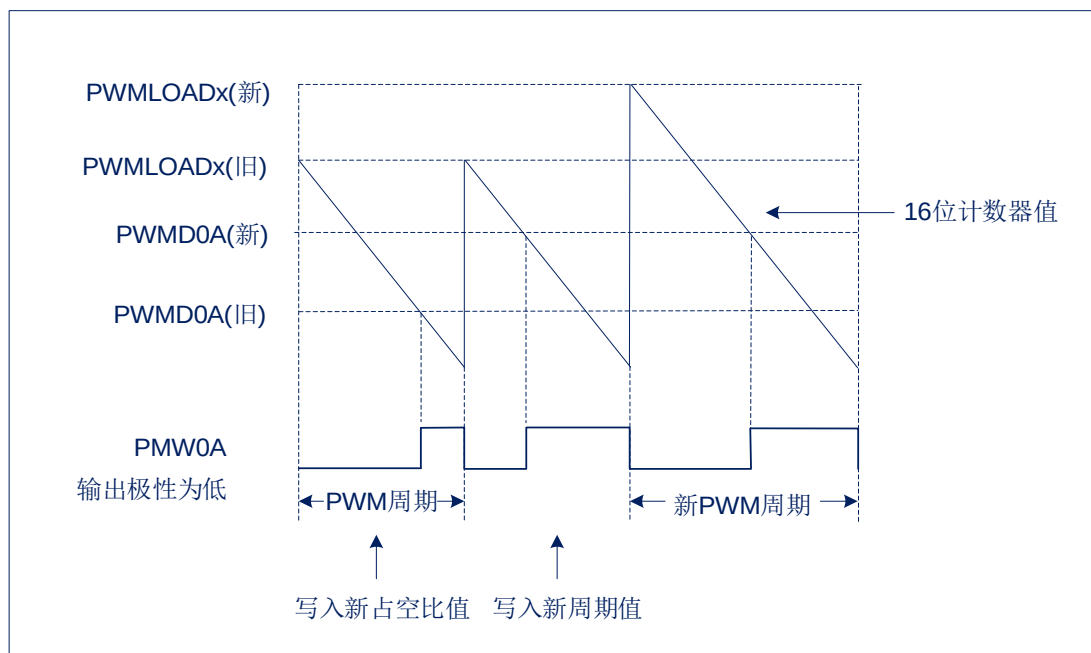
图 15-1: PWM 时序图
