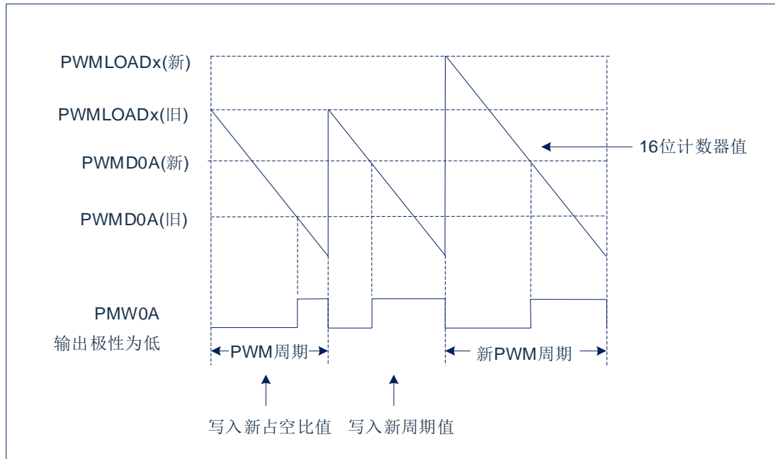
图 15-1: PWM 时序图
