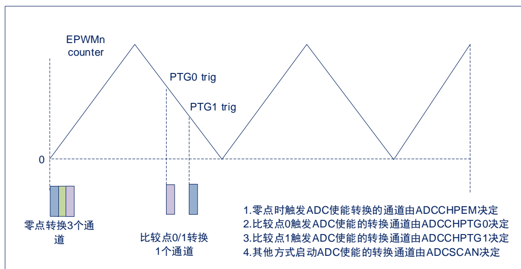
图 21-2: EPWM 触发启动 ADC 设置
