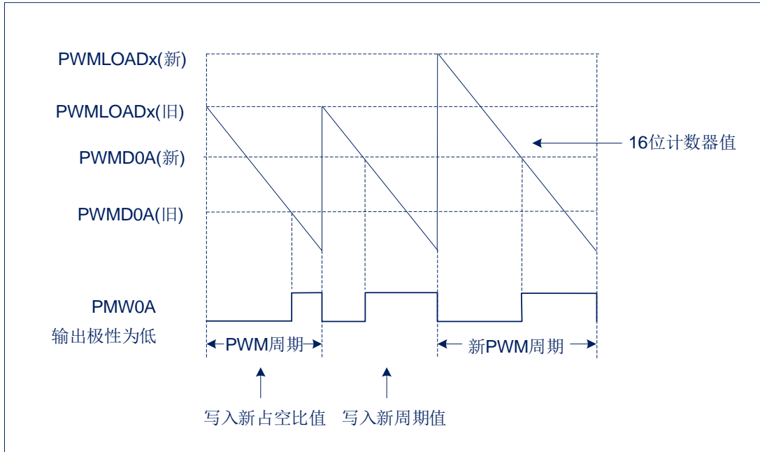
图 15-1: PWM 时序图
