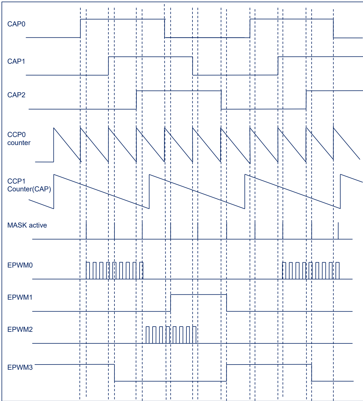
图 16-11: HALL 检测时序示例 (不代表实际运行波形)
