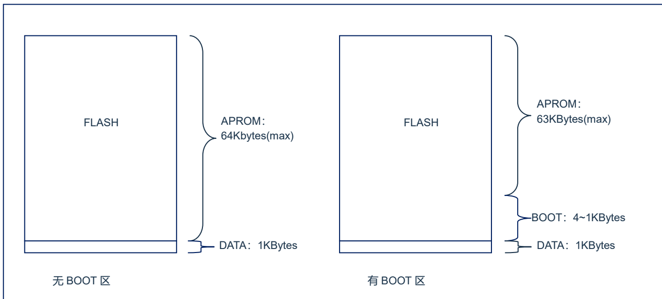
图 25-1: 存储器结构图
