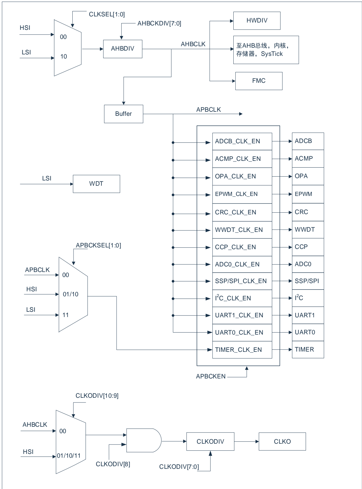
图 3-2: 时钟控制框图
