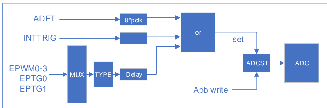
图 21-1: ADC 硬件触发启动
