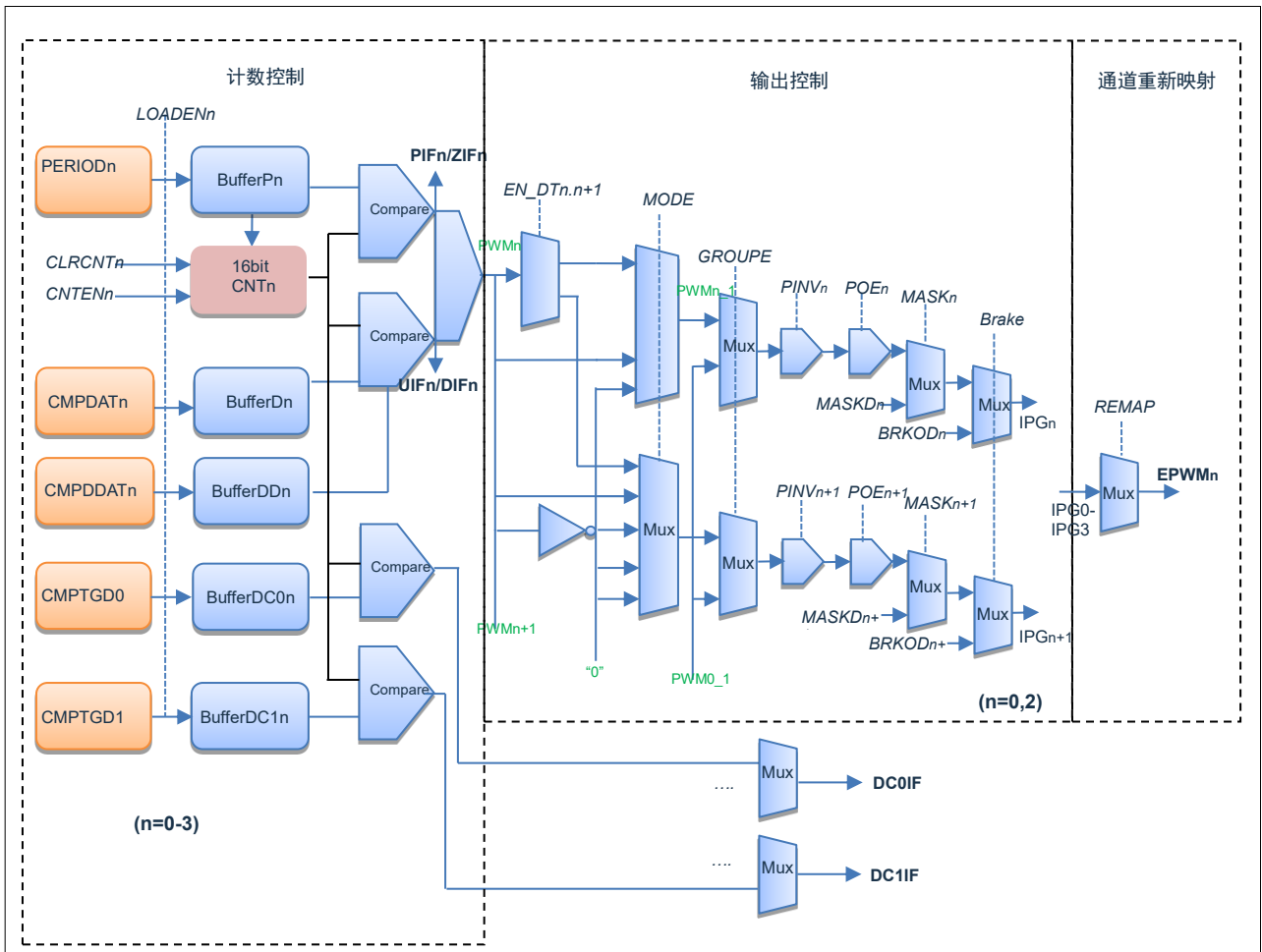
图 16-1: IPG n 的信号为 EPWM n 重映射前的信号。
