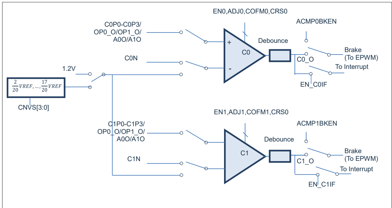
图 0-1：比较器结构图
