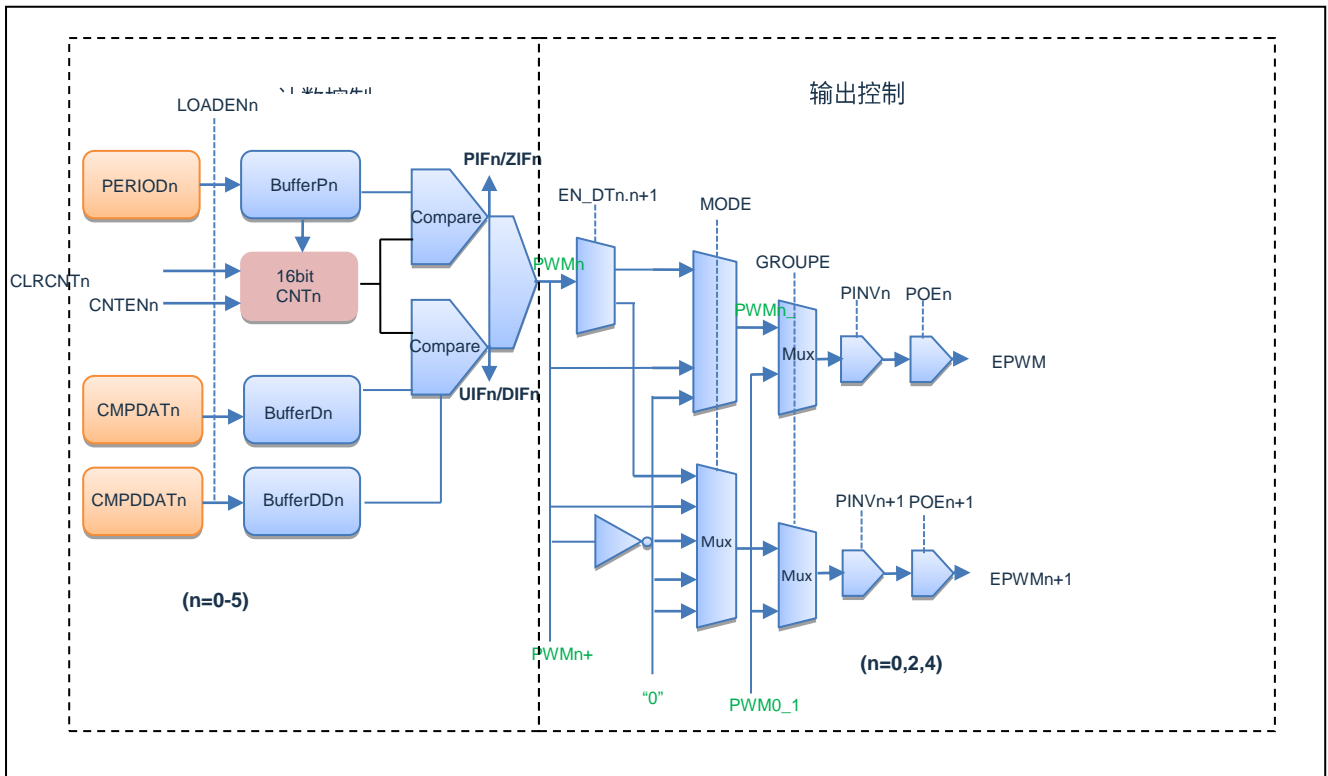
图 3-3: EPWM 结构图
