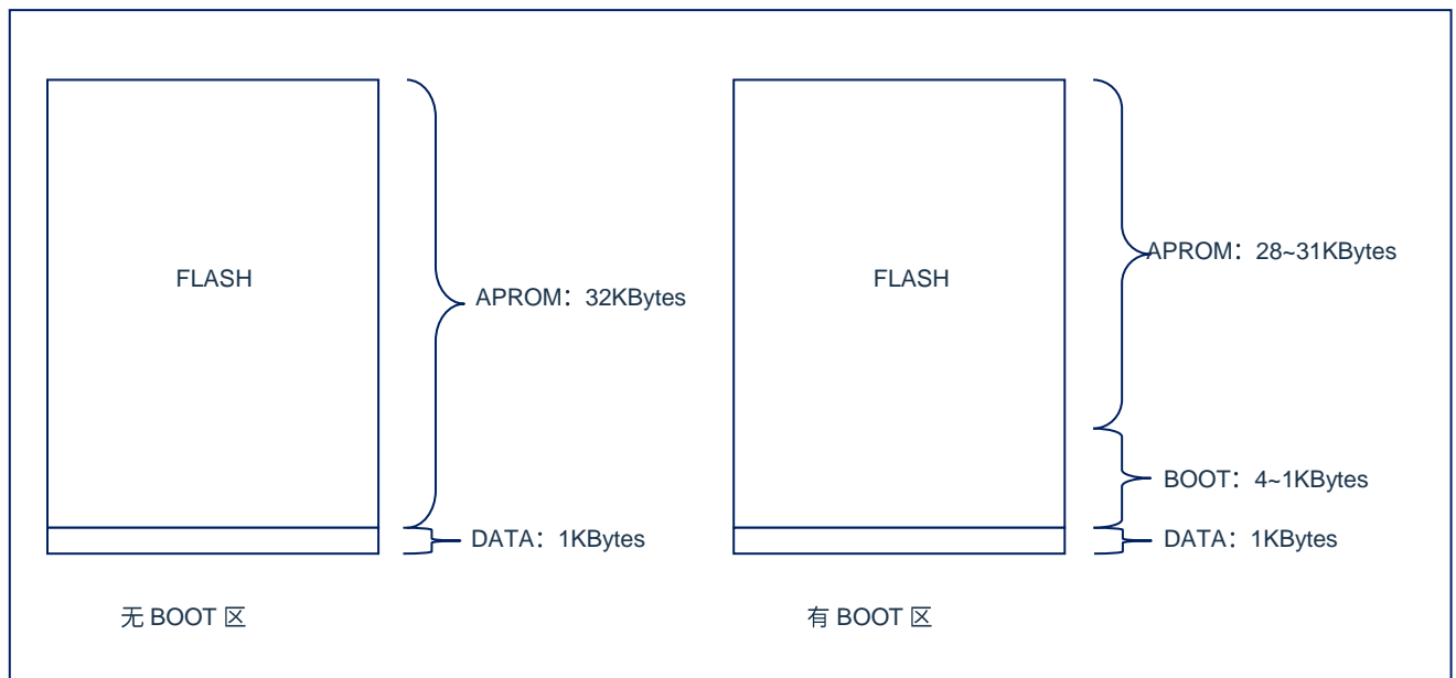
图 3-14: 存储器结构图
