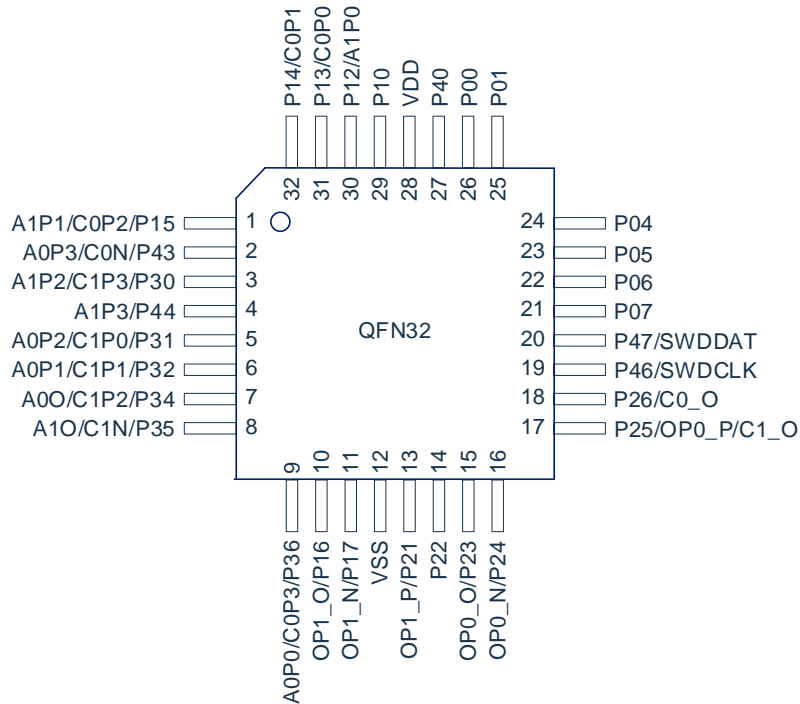
CMS32F033QN32
