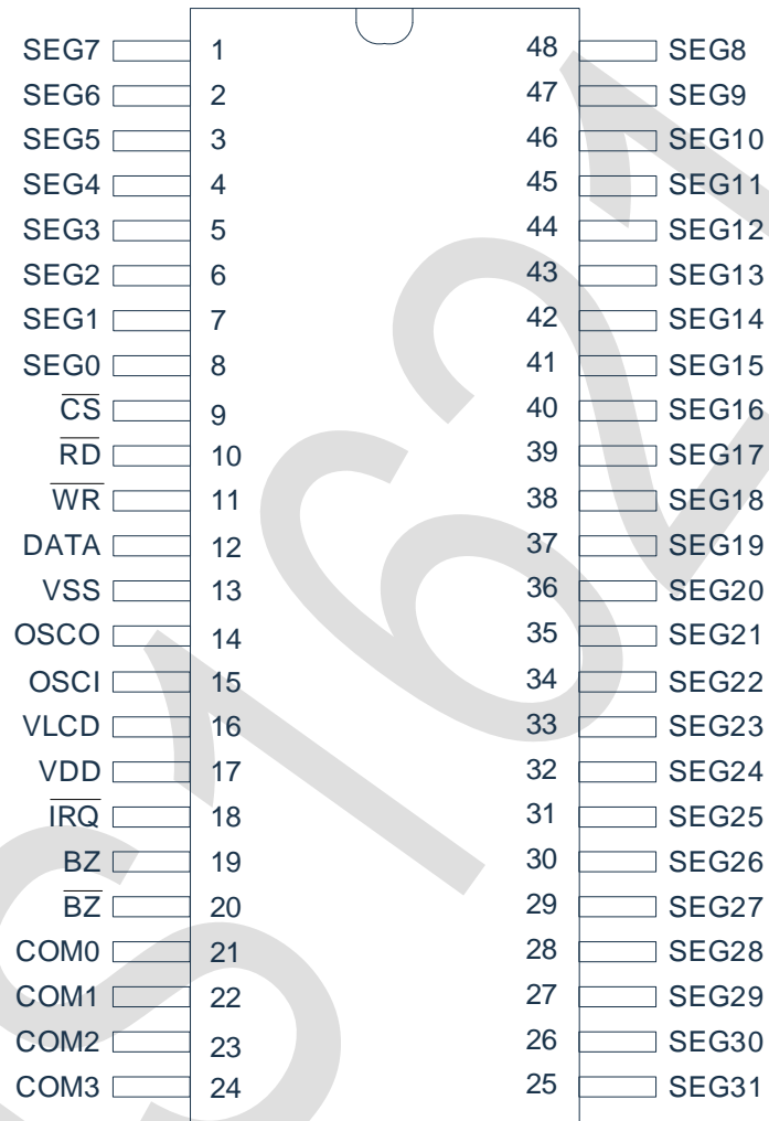
CMS1621_SSOP48
