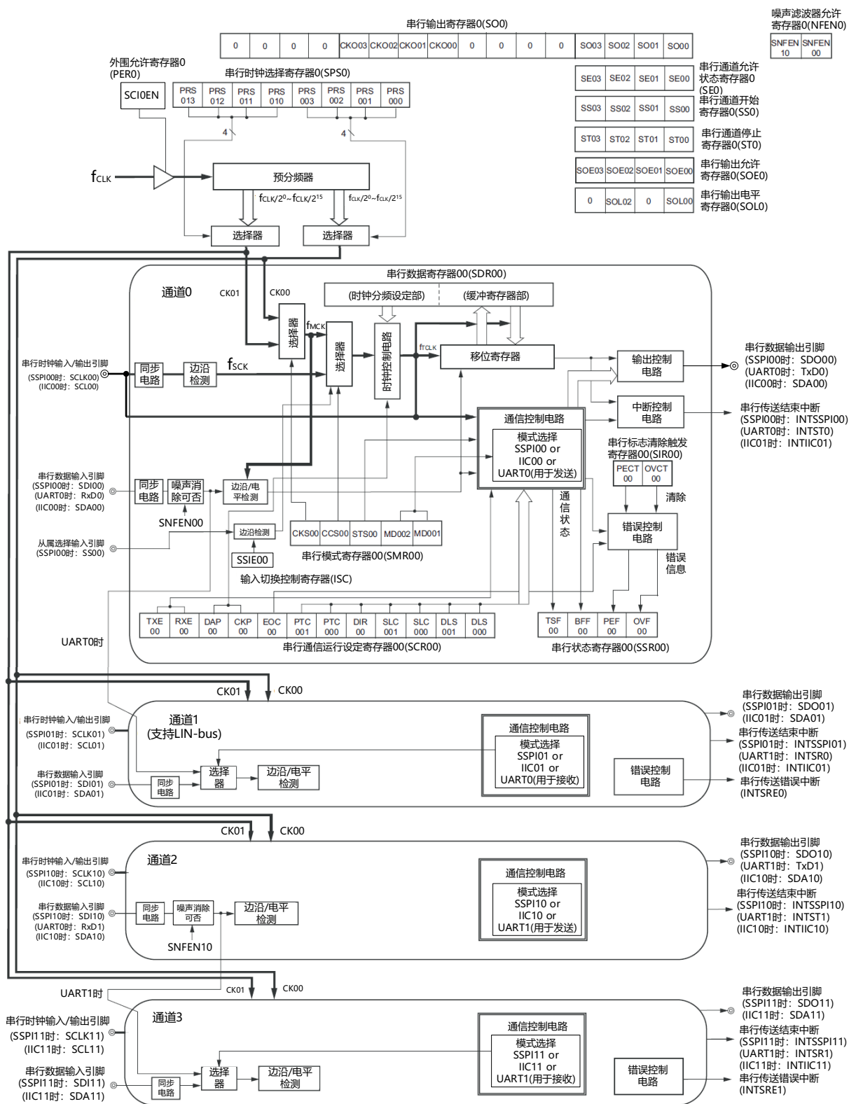
图14-1 通用串行通信单元0的框图
