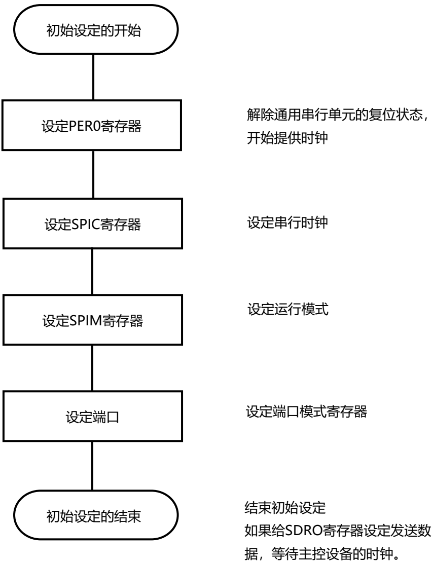
图15-13 从属发送/接收的初始设置步骤
