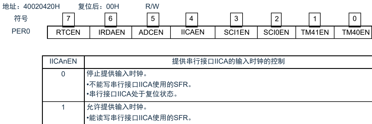
图16-5 外围允许寄存器0 (PER0) 的格式
