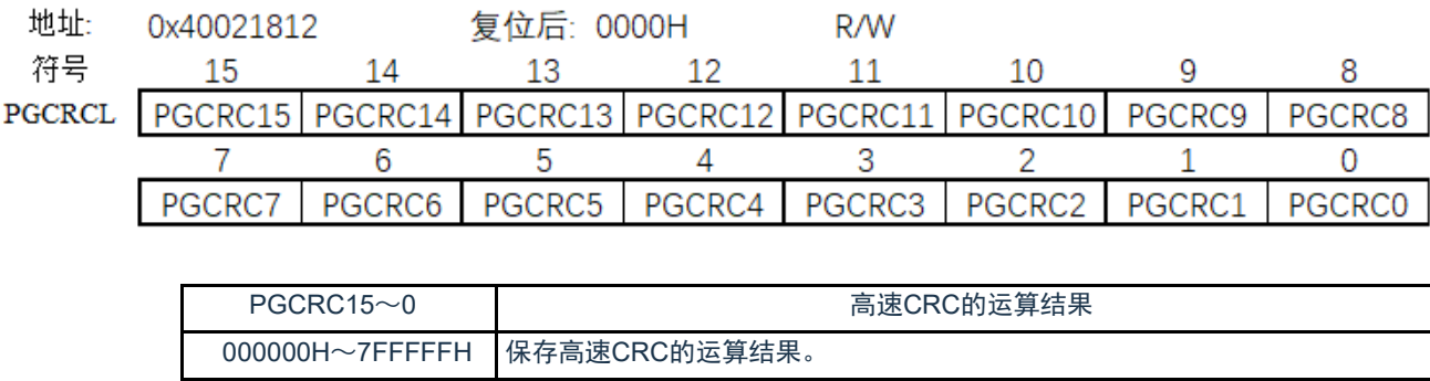
图26-2 闪存CRC运算结果寄存器（PGCRCL）的格式
