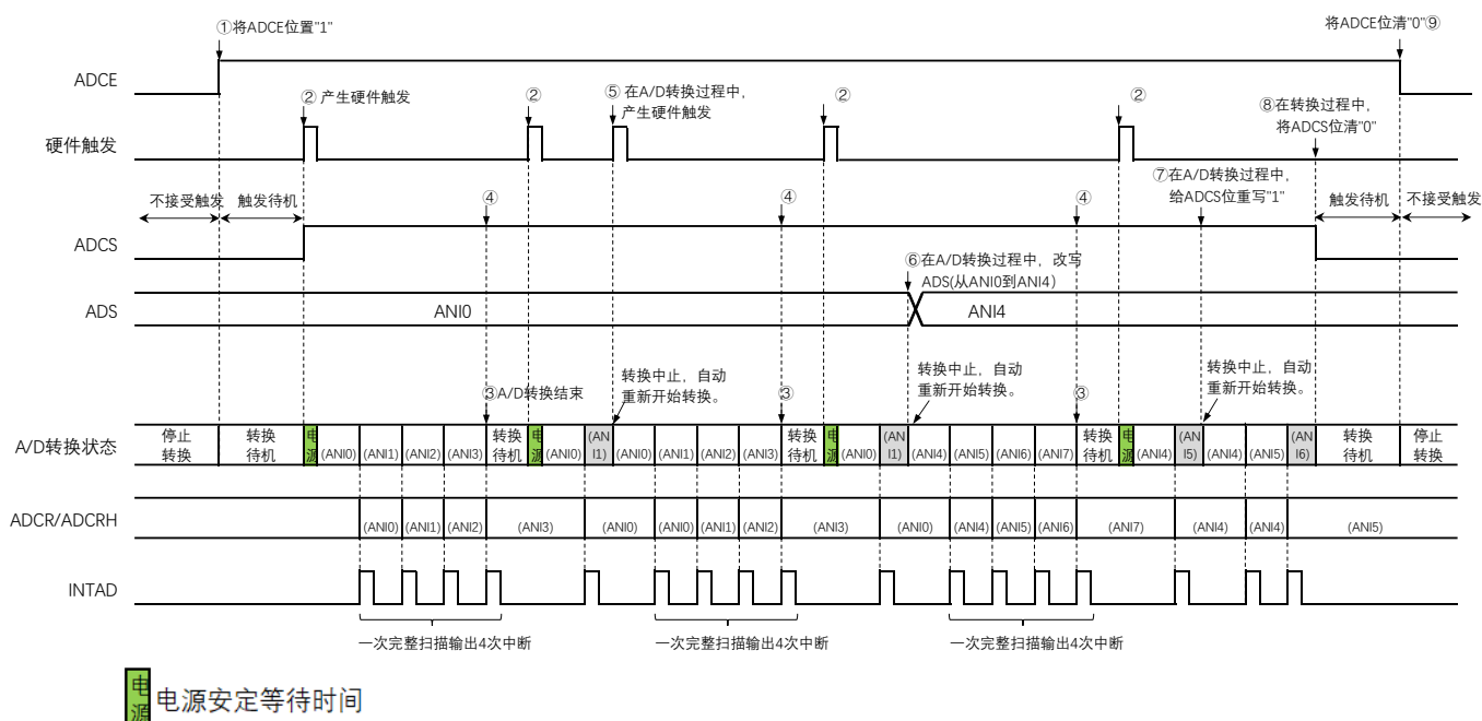
图 11-31 硬件触发等待模式（扫描模式、单次转换模式）的运行时序例子
