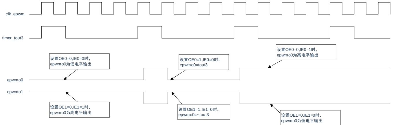
图6-8 输出时序图
