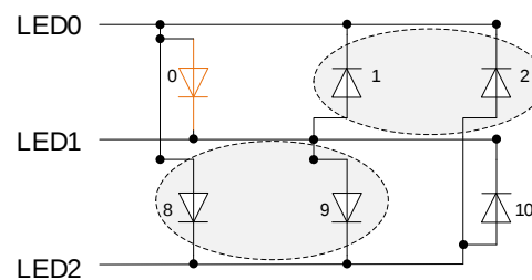
两灯示意图
