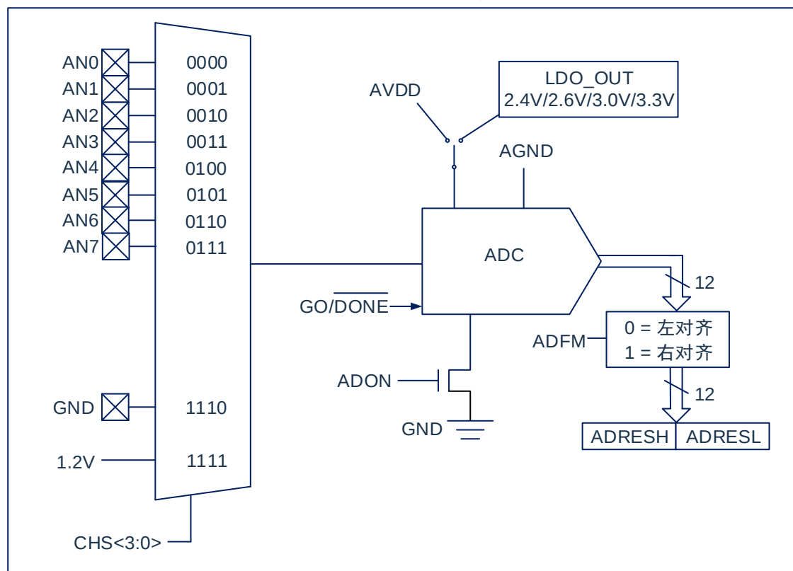
图 10-1: ADC 框图
