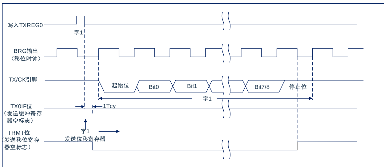
图 12-3: 异步发送
