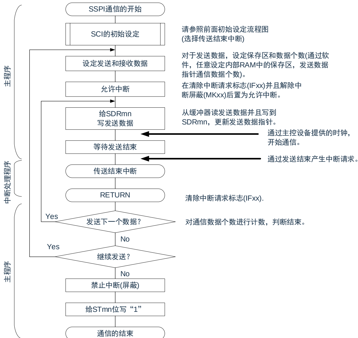
图 16-52: 从属发送（单次发送模式）的流程图
