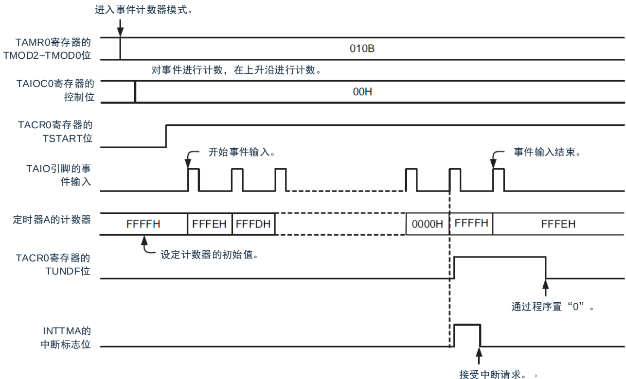
图 6-12：事件计数器模式的运行例子 1
