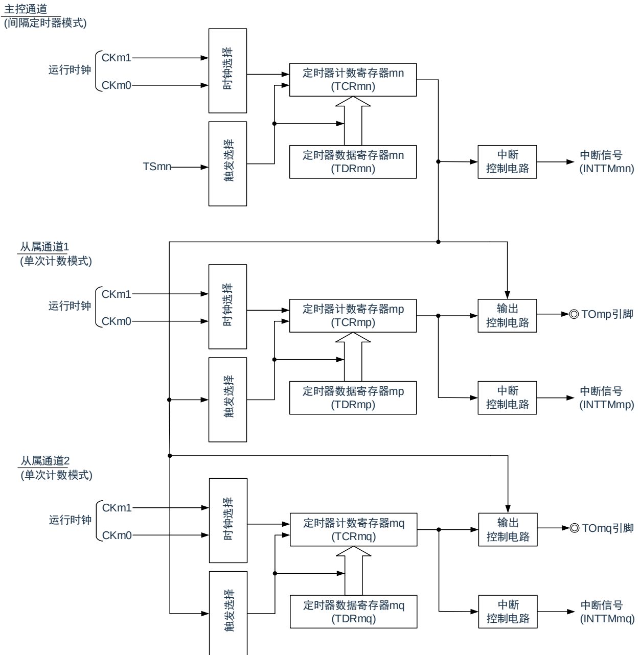
图 5-72：作为多重 PWM 输出功能运行的框图（输出 2 种 PWM 的情况）
