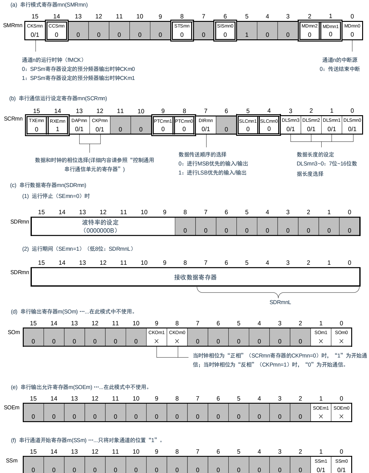
图 16-55: 3 线串行 I/O (SSPI00、SSPI01、SSPI10、SSPI11、SSPI20、SSPI21) 从属接收时的寄存器设定内容例子
