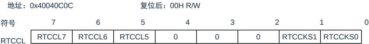
图 7-3：实时时钟选择寄存器（RTCCL）的格式
