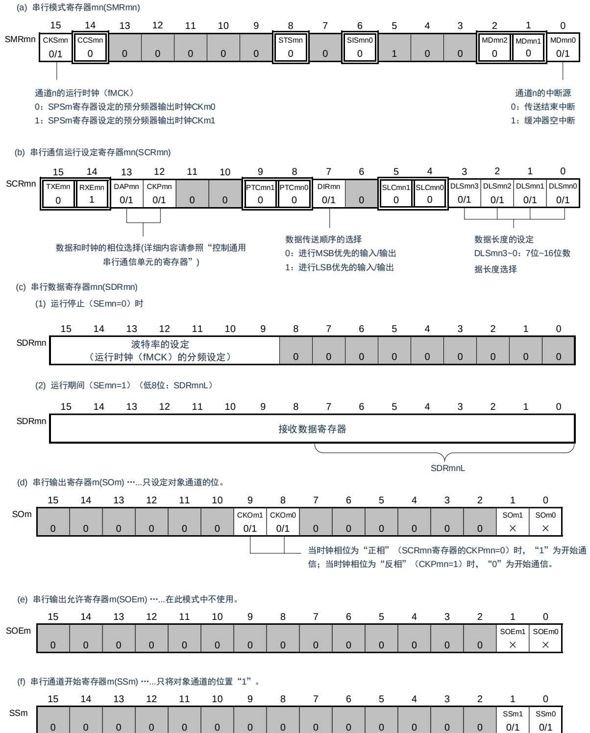
图 16-31：3 线串行 I/O（SSPI00、SSPI01、SSPI10、SSPI11、SSPI20、SSPI21） 主控接收时的寄存器设定内容例子
