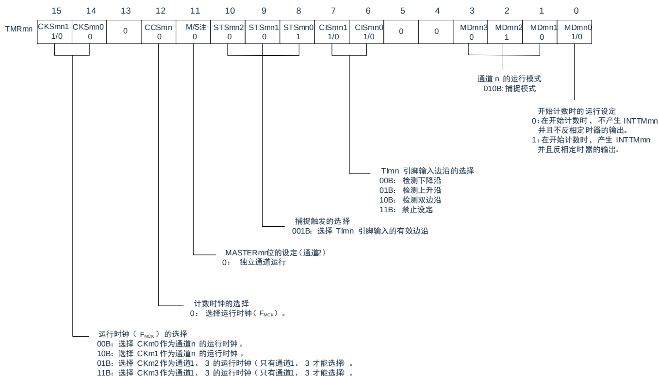
图 5-52：测量输入脉冲间隔时的寄存器设定内容例子
