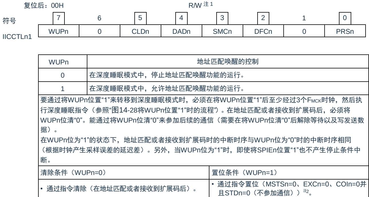
图 18-9：IICA 控制寄存器 n1（IICCTLn1）的格式(1/2)
