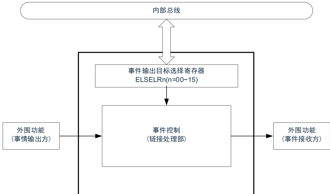
图 22-1：EVENTC 的框图
