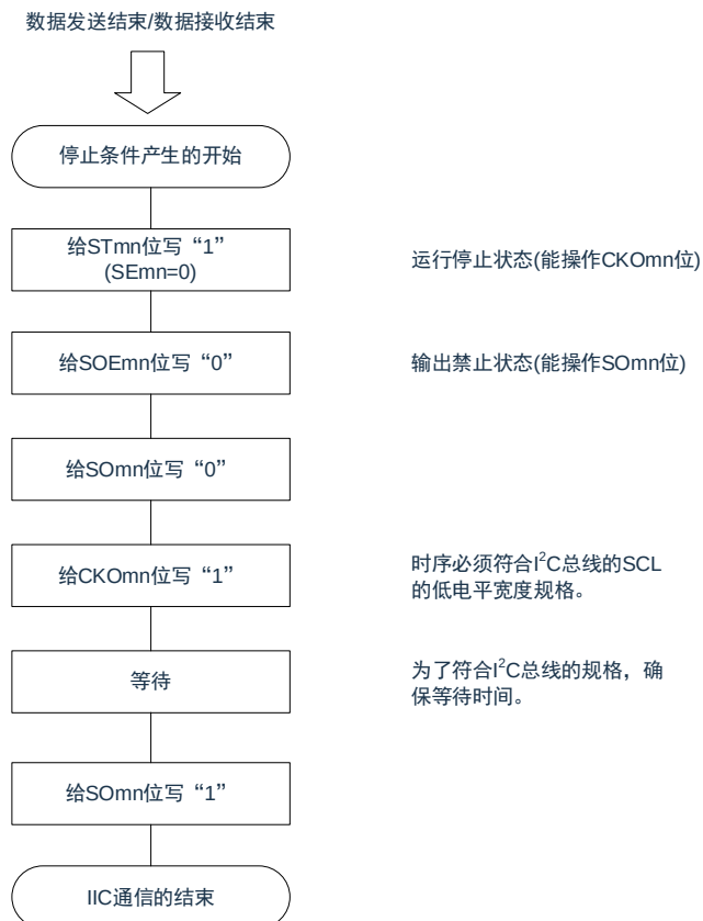
图 16-133：产生停止条件的流程图
