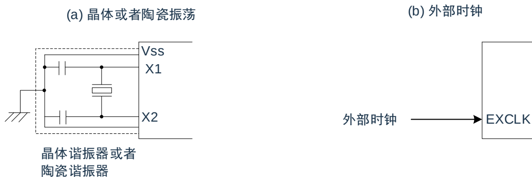
图 4-13：X1 振荡电路的外接电路例子
