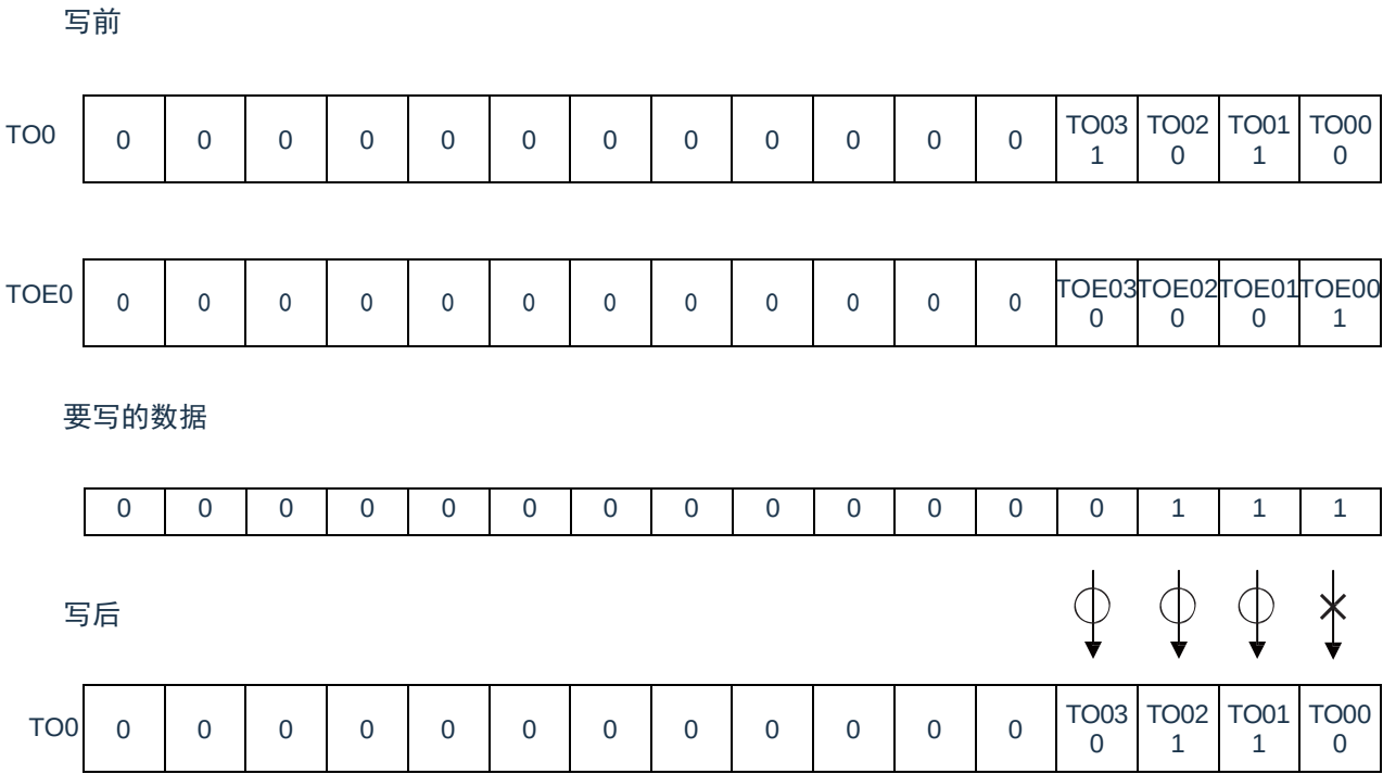
图 5-36: TO0n 位的一次性操作例子
