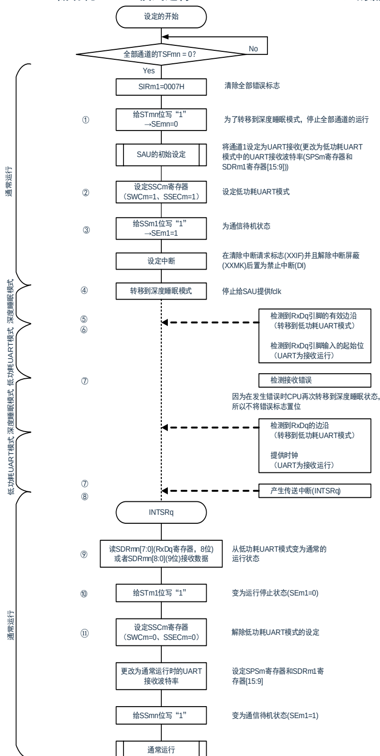
图 16-113: 低功耗 UART 模式运行 (EOCm1=1、SSECm=1) 的流程图
