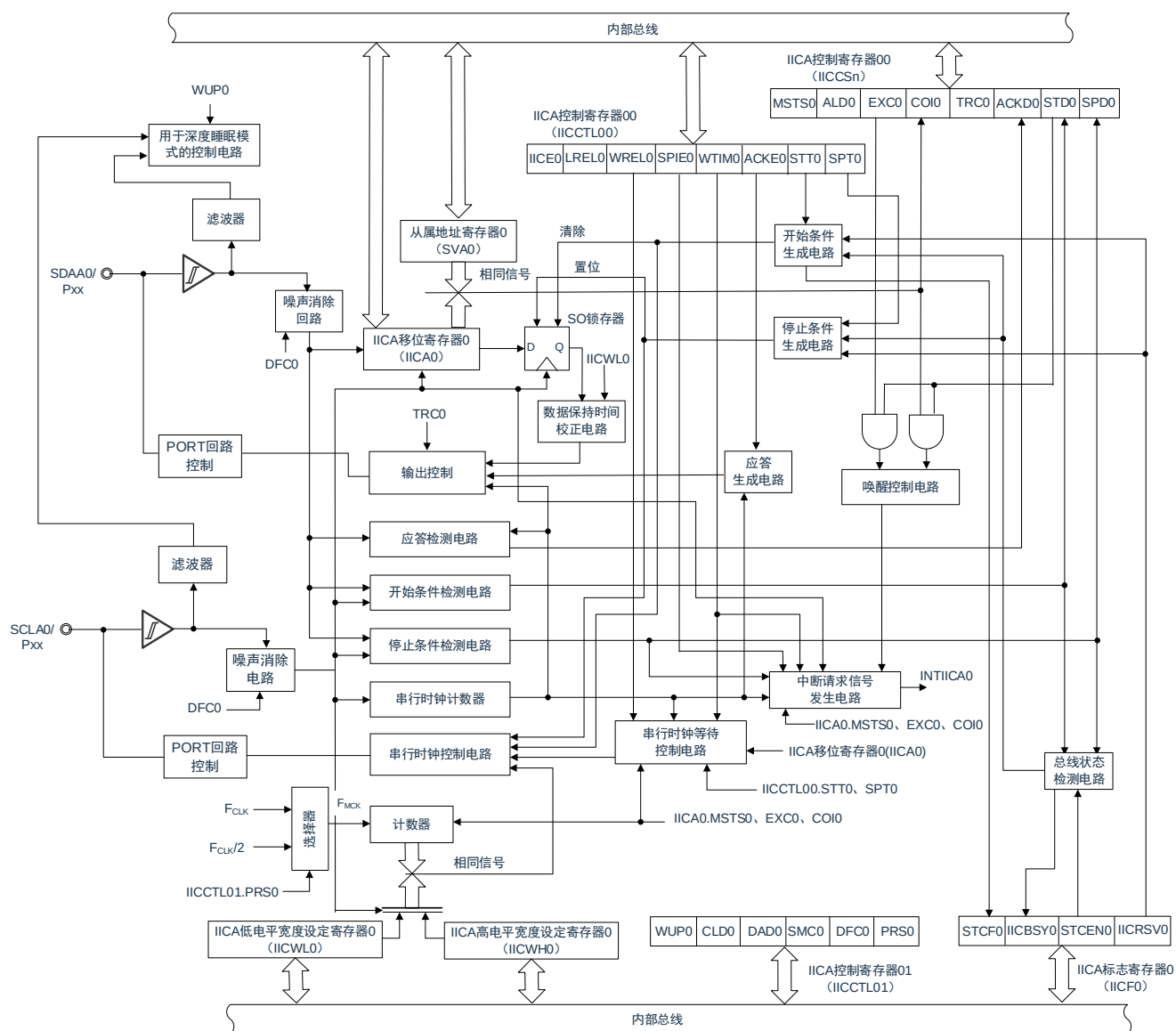
图 18-1: 串行接口 IICA 的框图
