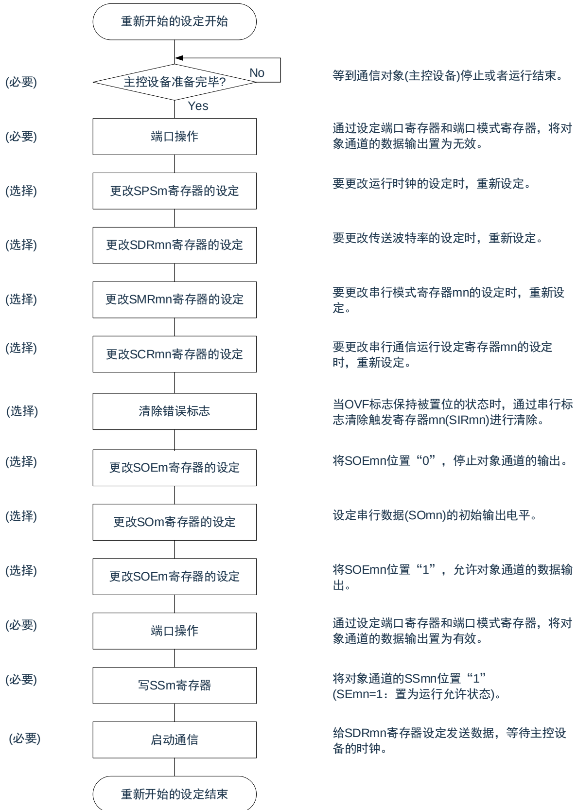
图 16-50：重新开始从属发送的设定步骤
