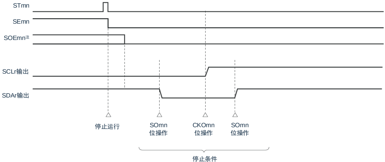
图 16-132：产生停止条件的时序图
