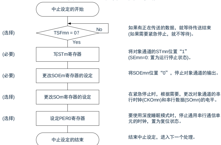
图 16-25：主控发送的中止步骤
