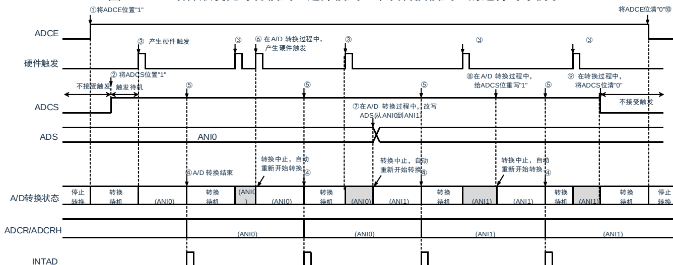
图 11-23：硬件触发无等待模式（选择模式、单次转换模式）的运行时序例子
