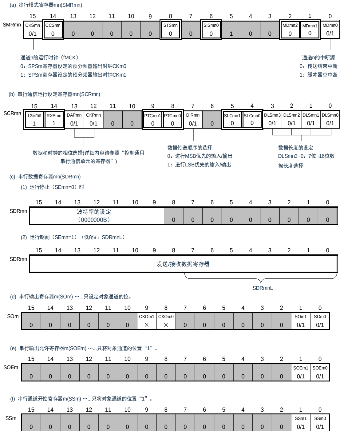
图 16-61: 3 线串行 I/O (SSPI00、SSPI01、SSPI10、SSPI11、SSPI20、SSPI21) 从属发送和接收时的寄存器设定内容例子
