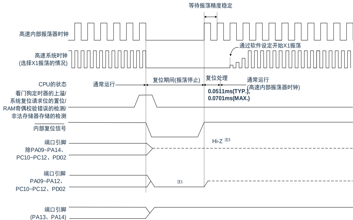
图 26-3: 因看门狗定时器的上溢、系统复位请求位的置位、RAM 奇偶校验错误的检测 或者非法存储器存取检测而产生的复位时序
