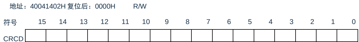
图 29-5: CRC 数据寄存器（CRCD）的格式
