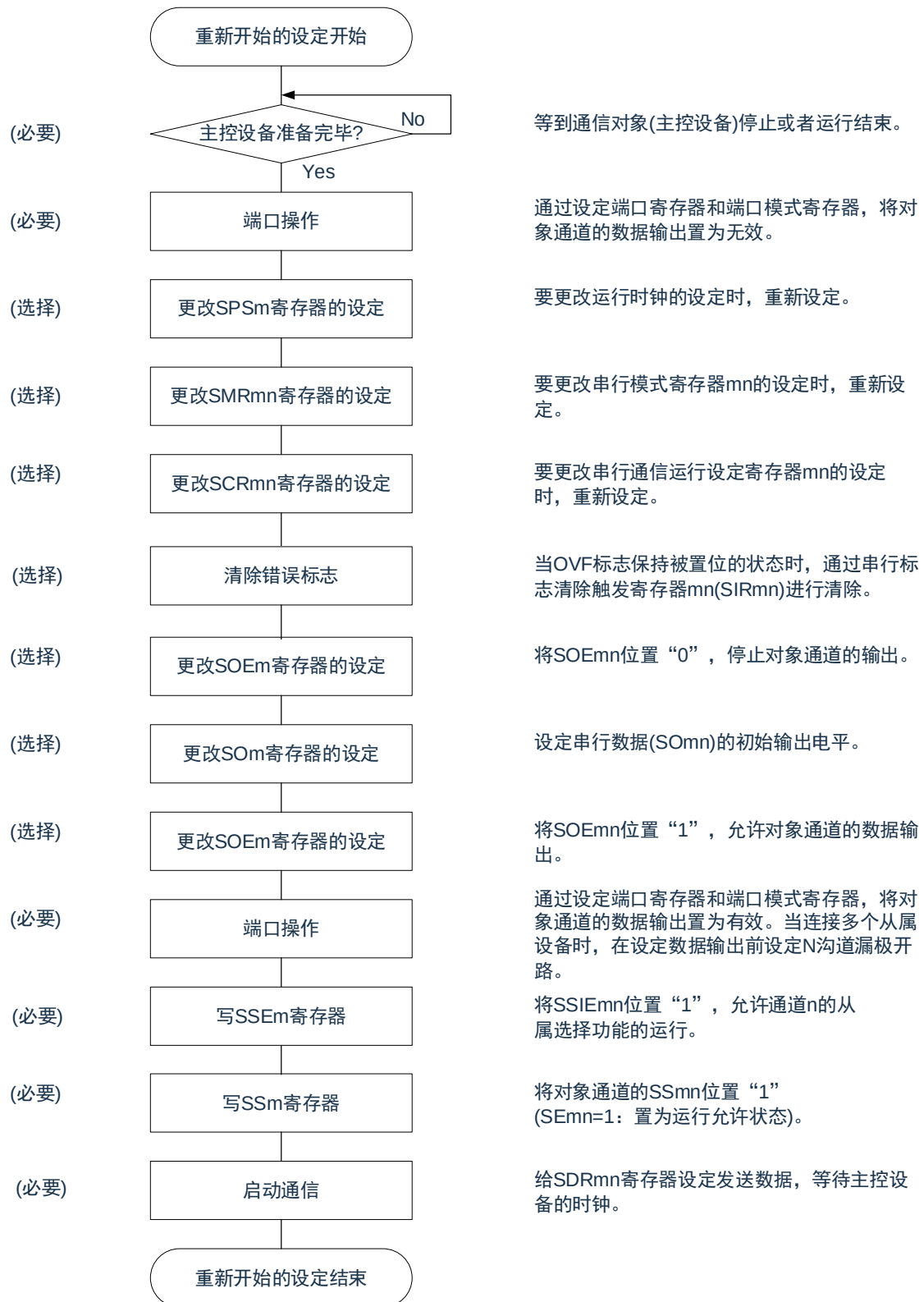
图 16-90：重新开始从属发送和接收的设定步骤
