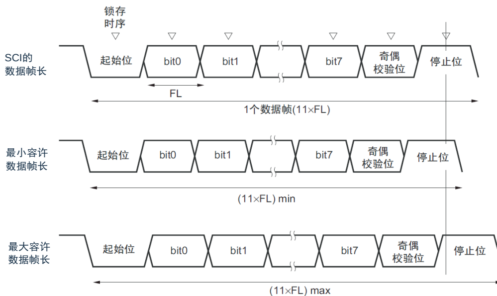
图 16-114: 接收时的波特率容许范围 (1 个数据帧的帧长=11 位的情况)
