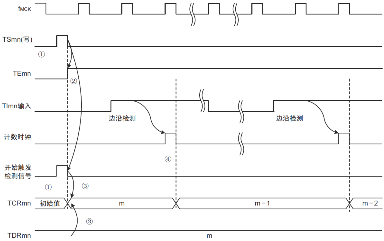
图 5-26: 运行时序 (事件计数器模式)
