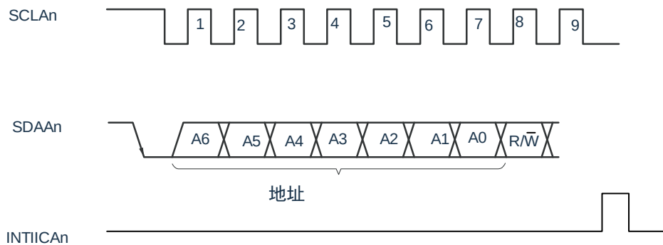
图 18-15：地址
