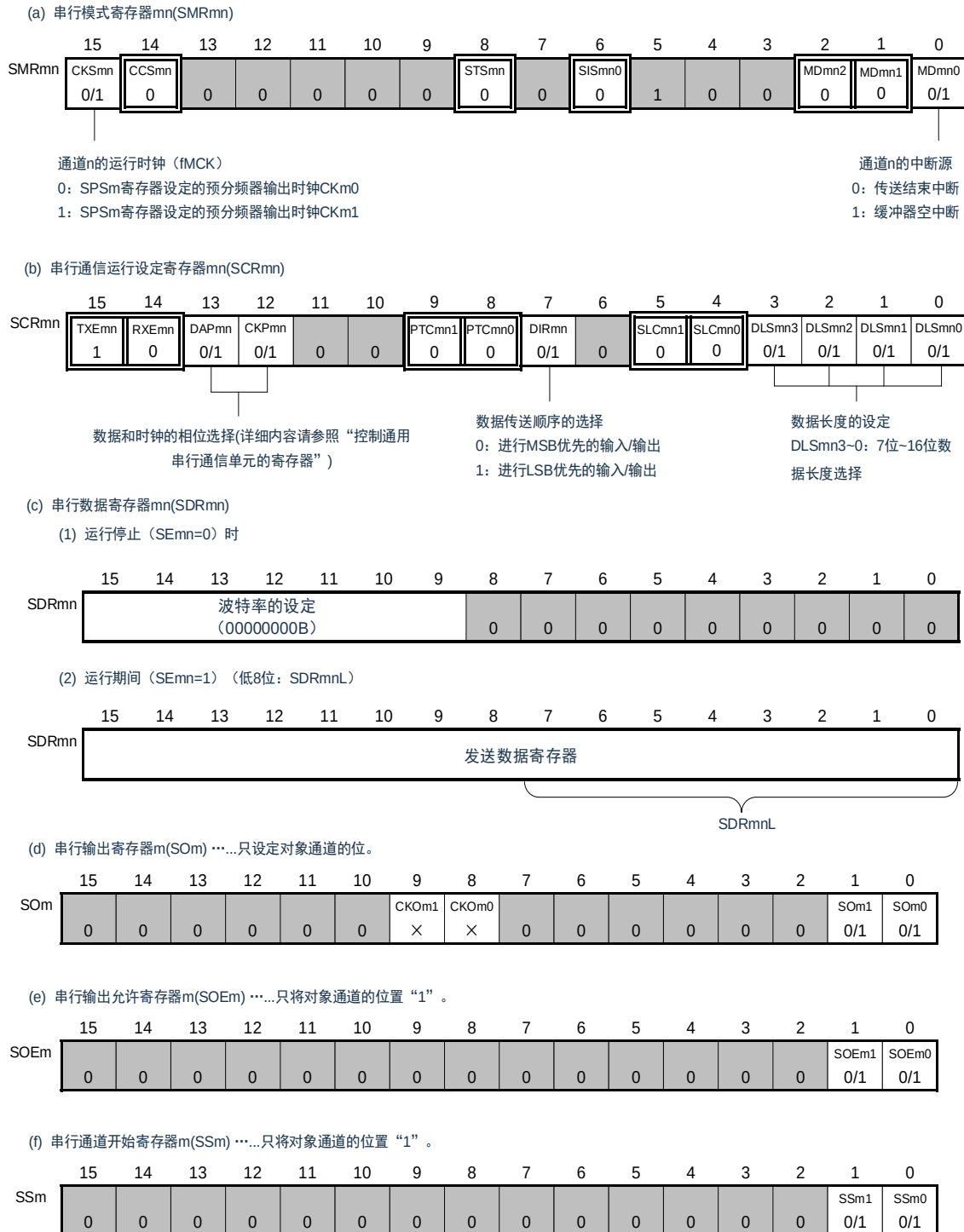
图 16-47：3 线串行 I/O（SSPI00、SSPI01、SSPI10、SSPI11、SSPI20、SSPI21） 从属发送时的寄存器设定内容例子
