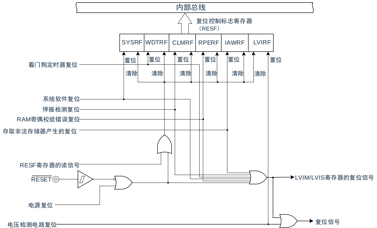
图 26-1: 复位功能的框图
