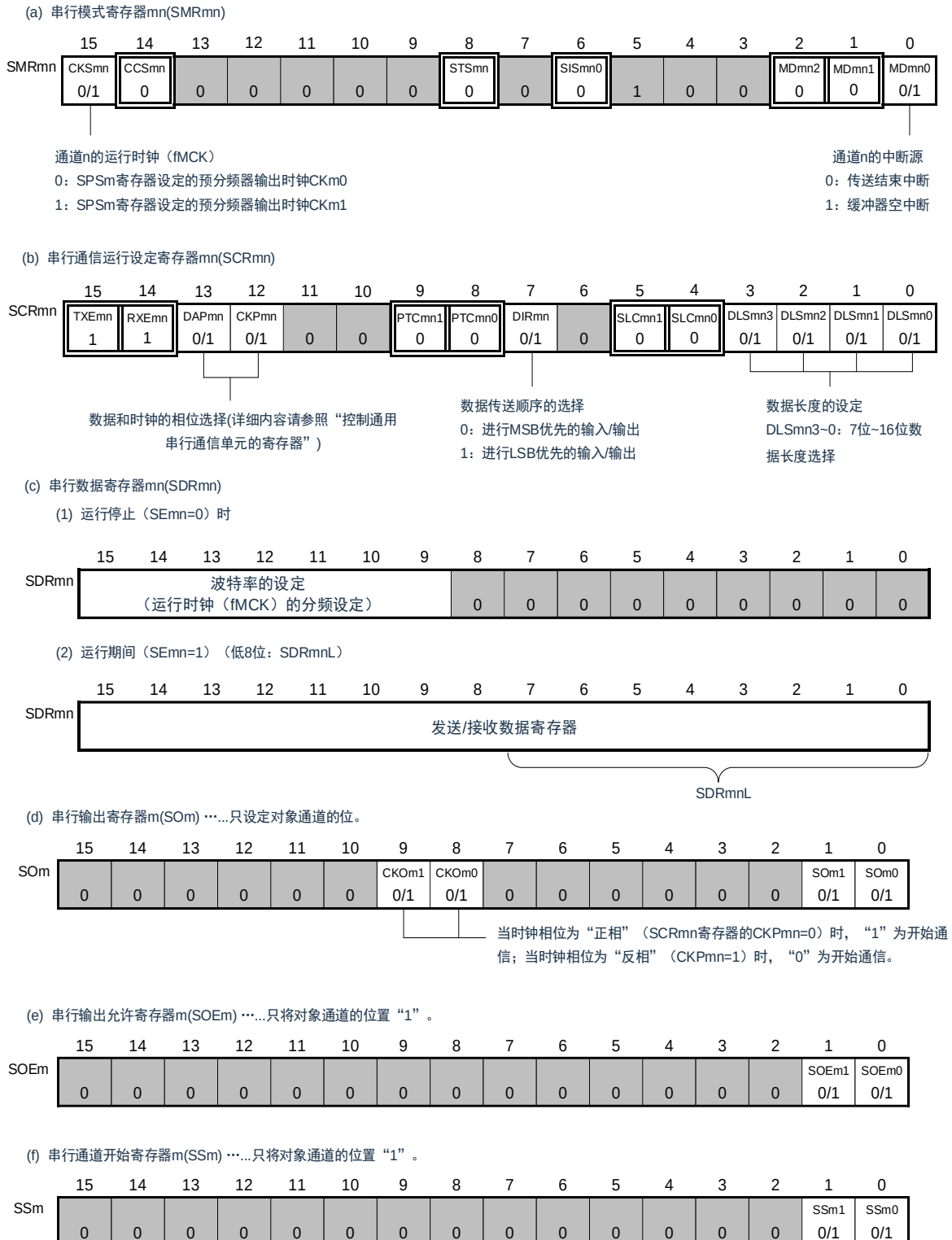
图 16-39: 3 线串行 I/O (SSPI00、SSPI01、SSPI10、SSPI11、SSPI20、SSPI21) 主控发送和接收时的寄存器设定内容例子
