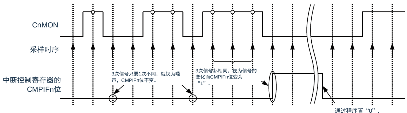
图 14-12: 比较器 n (n=0、1) 的数字滤波器和中断运行例子
