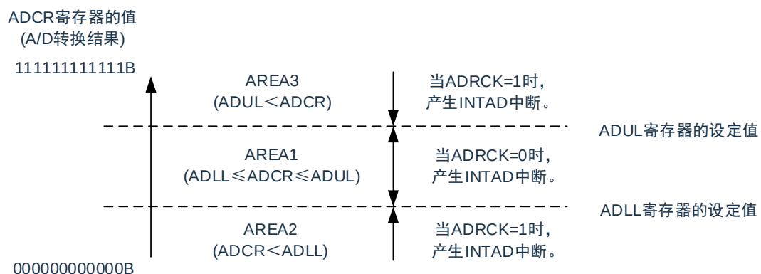
图 11-6: ADRCK 位的中断信号产生范围
