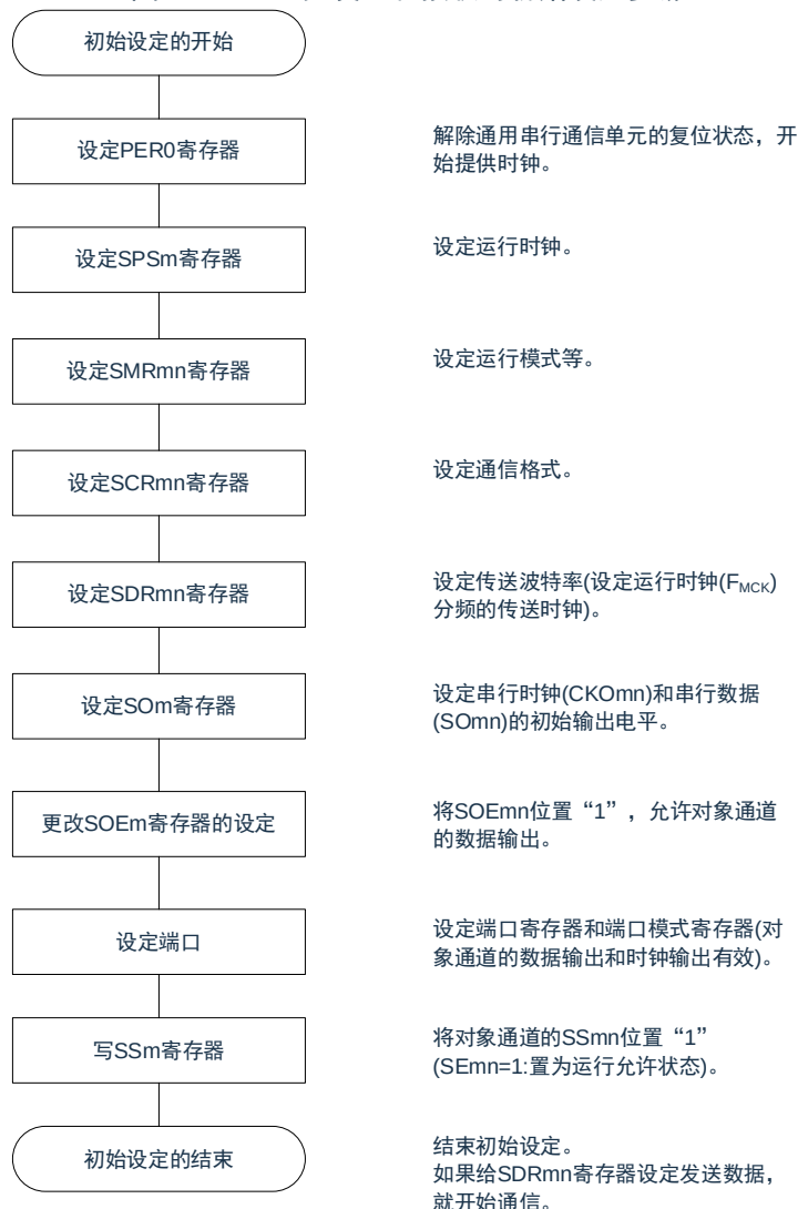
图 16-40：主控发送和接收的初始设定步骤
