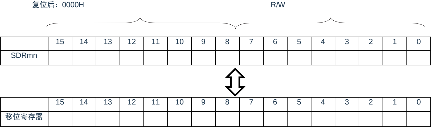
图 16-2：串行数据寄存器 mn（SDRmn）的格式
