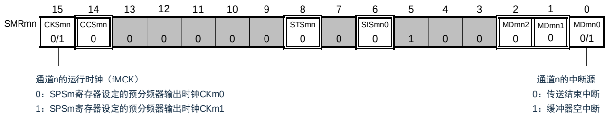
图 16-23: 3 线串行 I/O (SSPI00、SSPI01、SSPI10、SSPI11、SSPI20、SSPI21) 主控发送时的寄存器设定内容例子
