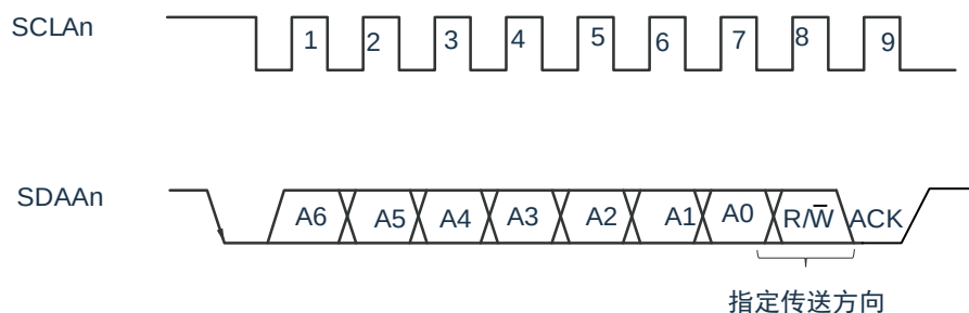
图 18-17: 应答
