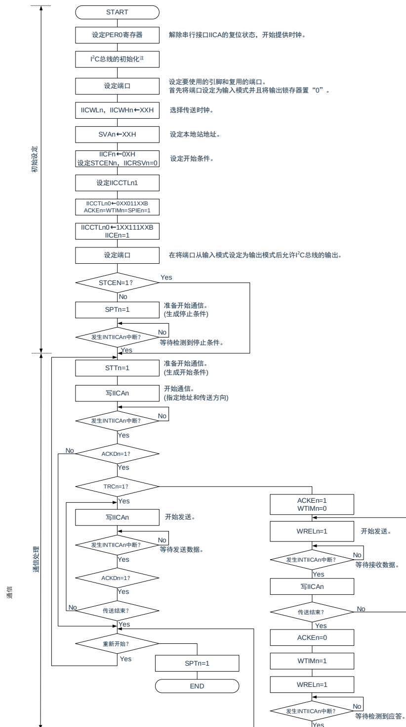
图 18-27：单主控系统的主控运行
