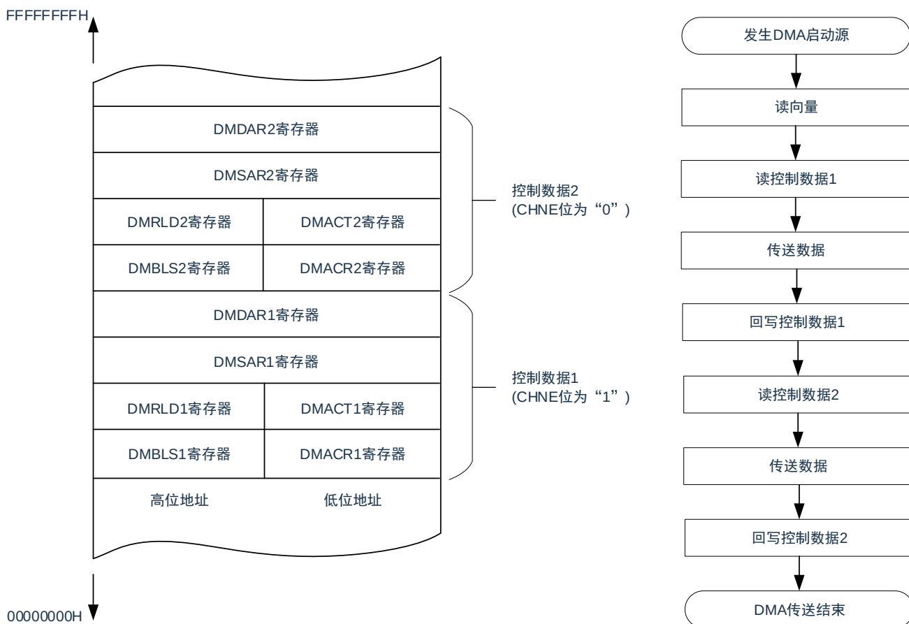
图 21-21：链传送的流程图
