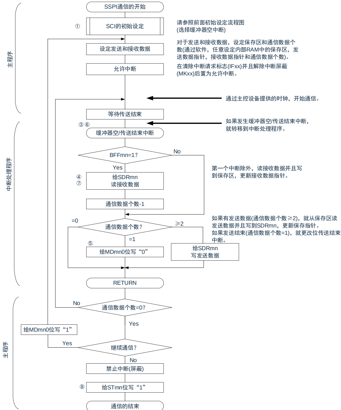
图 16-94: 从属发送和接收（连续发送和接收模式）的流程图
