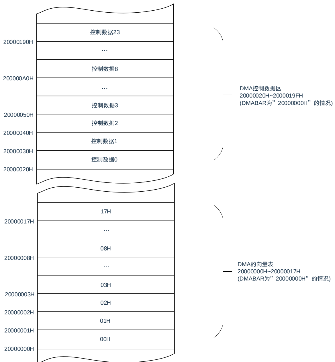
图 21-4：控制数据的起始地址和向量表 DMABAR 寄存器的设置值为“2000_0000H”的情况（例）
