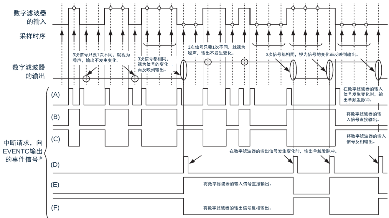
图 14-13: 数字滤波器、中断请求和向 EVENTC 输出事件信号的运行
