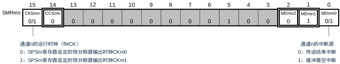
图 16-96: UART (UART0~UART2) 的 UART 发送时的寄存器设定内容例子(1/2)
