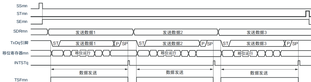
图 16-100: UART 发送（单次发送模式）的时序图
