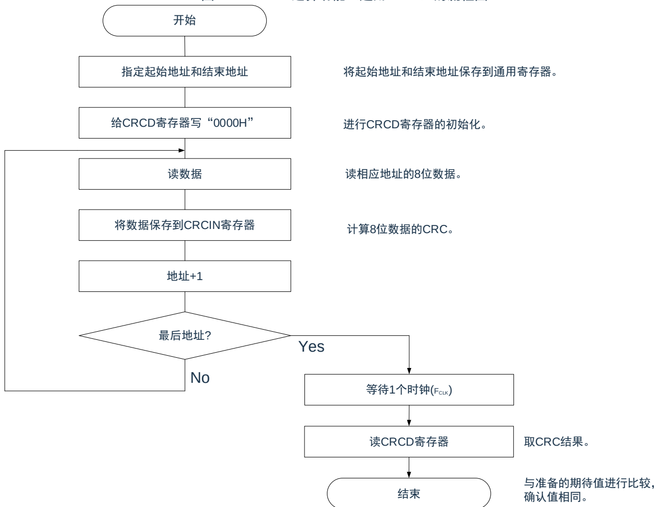
图 29-6: CRC 运算功能（通用 CRC）的流程图
