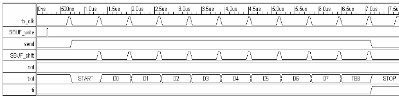
图 16-3：UARTn 通信模式 2 时序图
