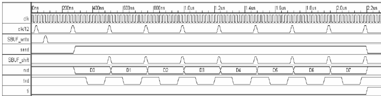
图 16-1：通信模式 0 时序图
