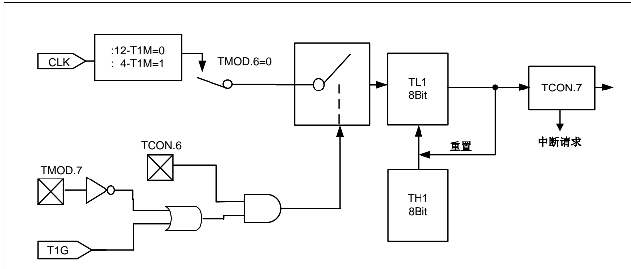
图 8-7: Timer1, 模式 2: 8-位定时/计数器（自动重装）
