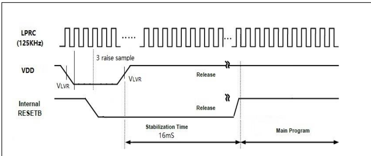
图 4-2: LVR 低压复位时序图
