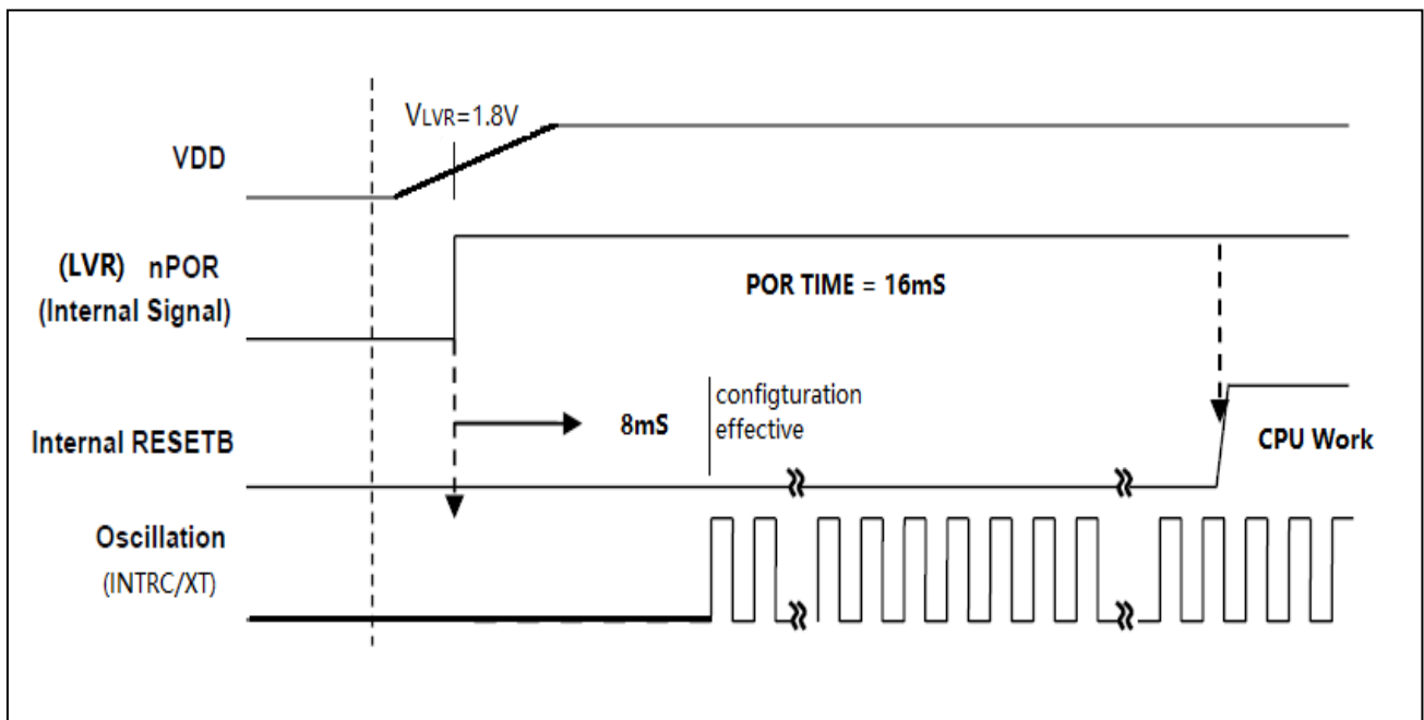
图 4-1：上电复位时序图
