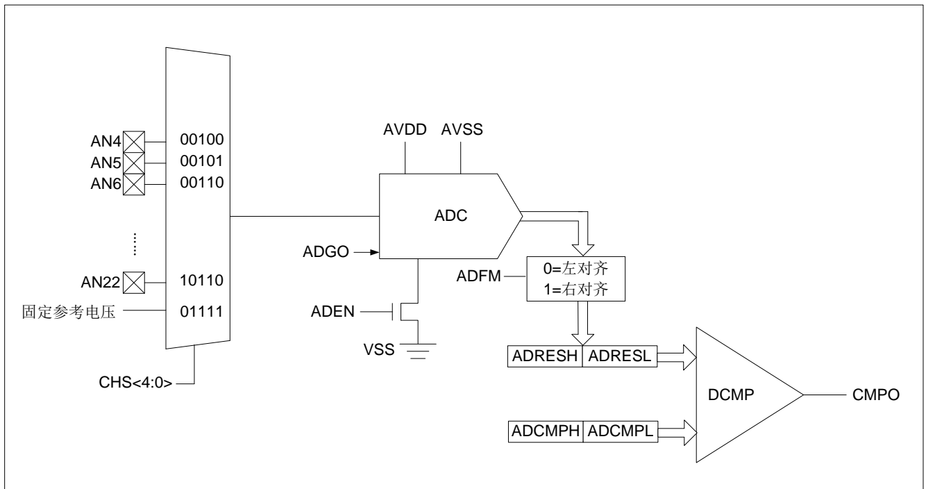
图 12-1: ADC 框图
