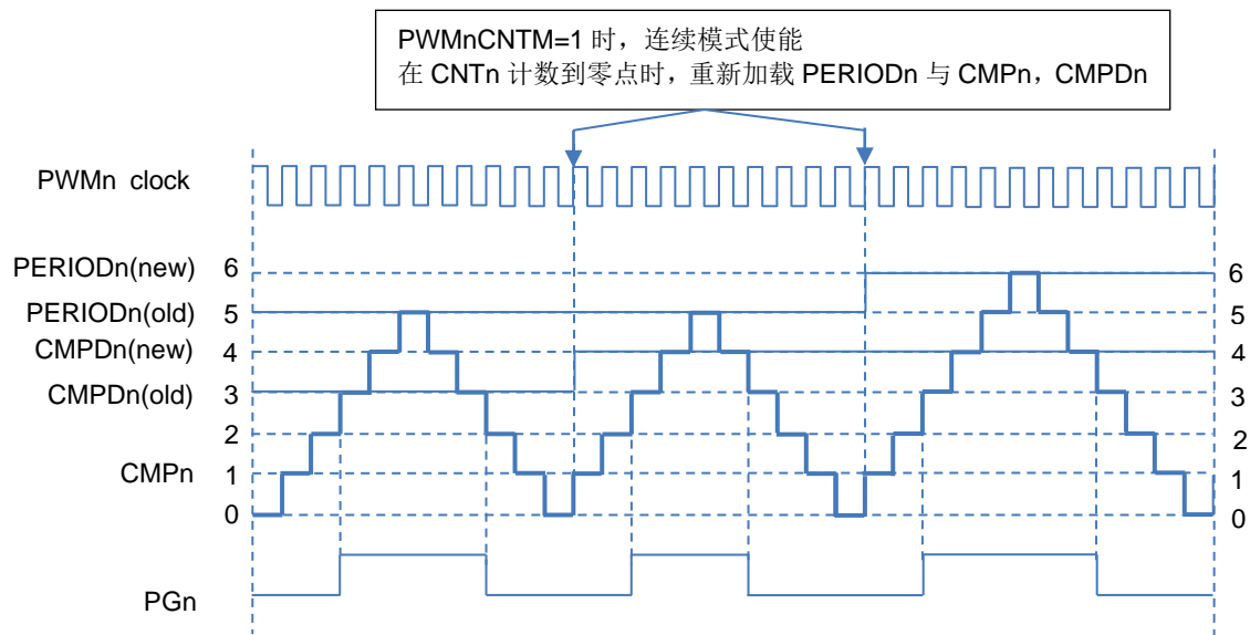
图 13-5：中心对齐时序图（非对称计数）
