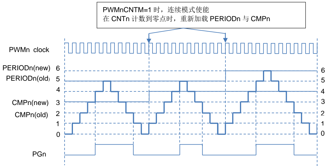
图 13-3: 中心对齐计数器波形（对称计数）
