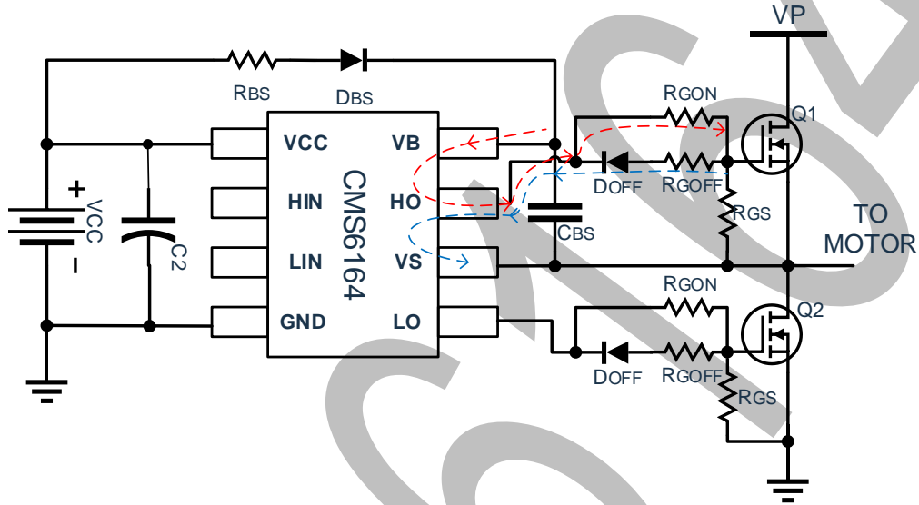
图 8-2：栅极输出驱动电路示意
