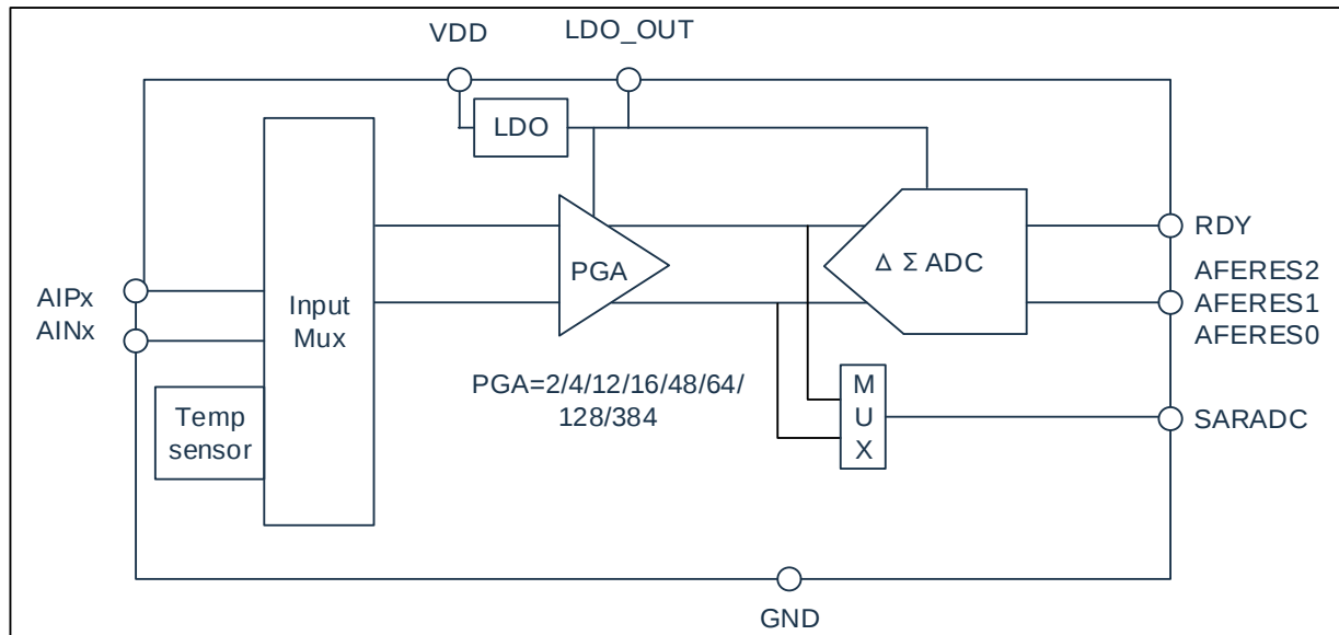
图 11-1: AFE 框图
