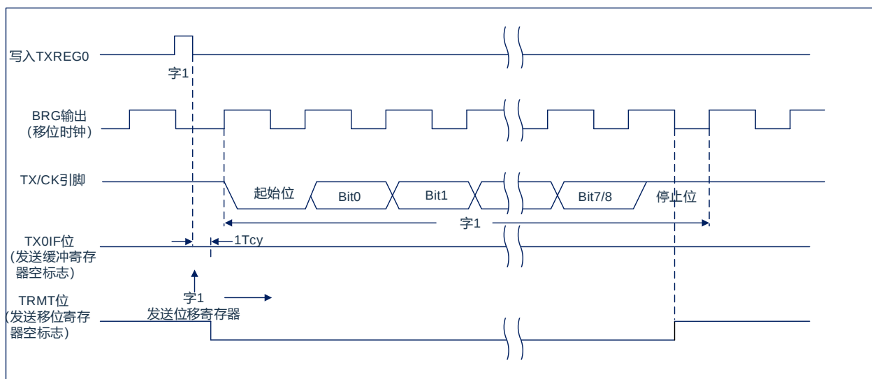
图 13-3: 异步发送
