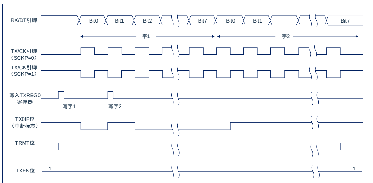
图 13-6: 同步发送
