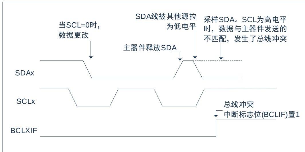
图 15-16: 发送和应答时的总线冲突时序
