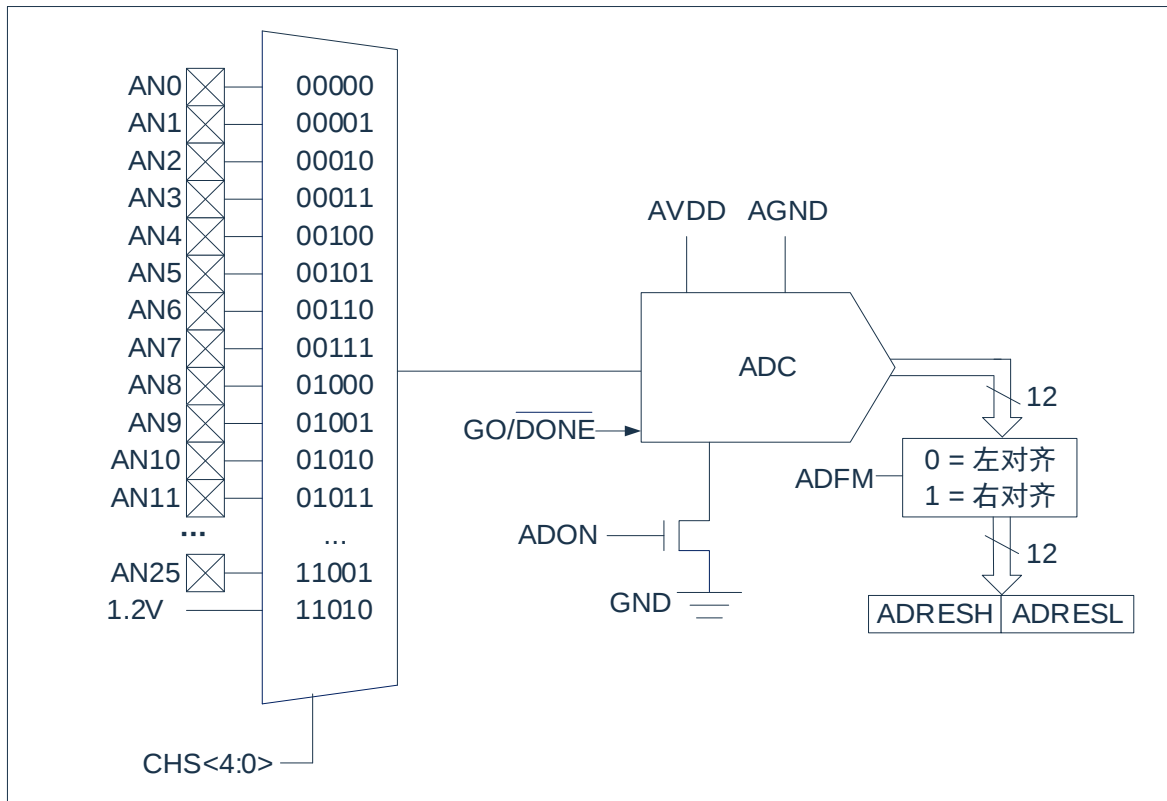
图 11-1：ADC 框图
