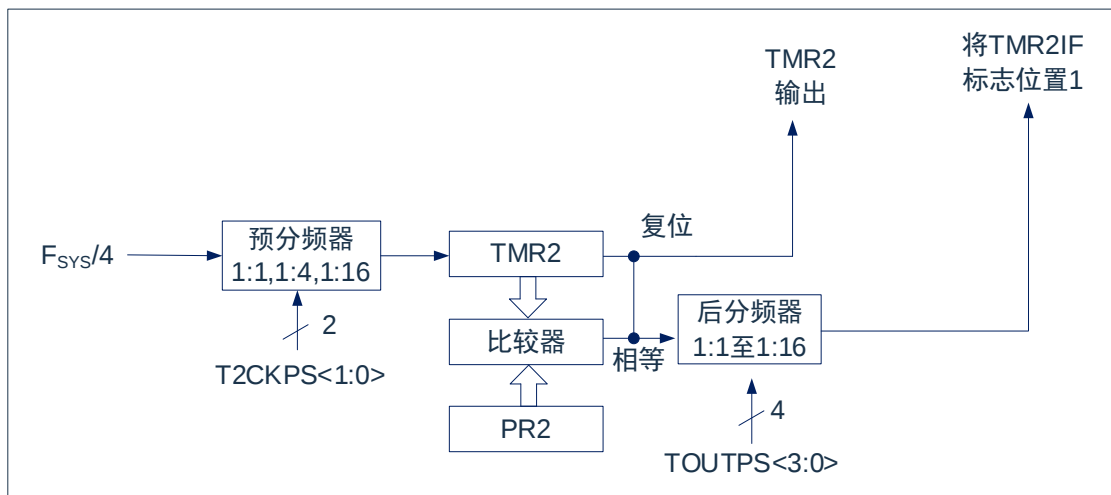
图 10-1: TIMER2 框图
