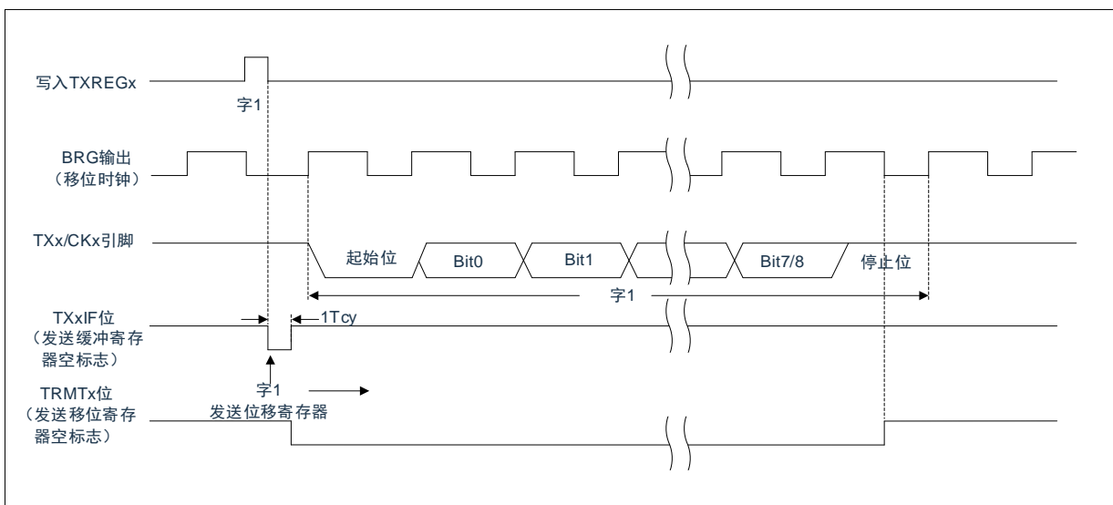
图 14-3: 异步发送
