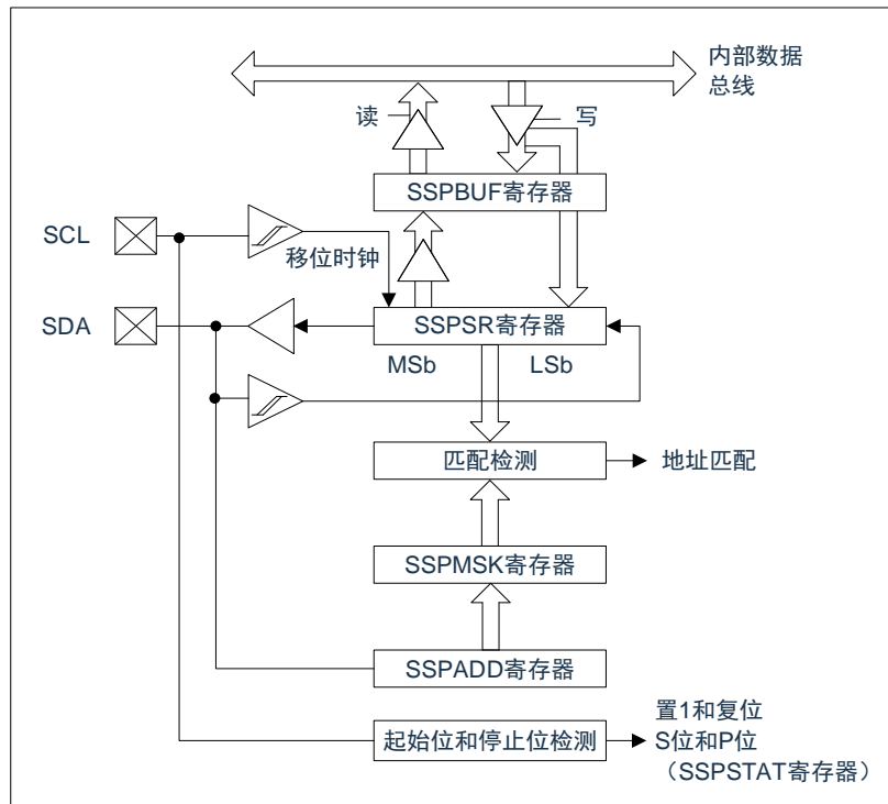
图 15-6: MSSP 框图 (I 2 C 模式)
