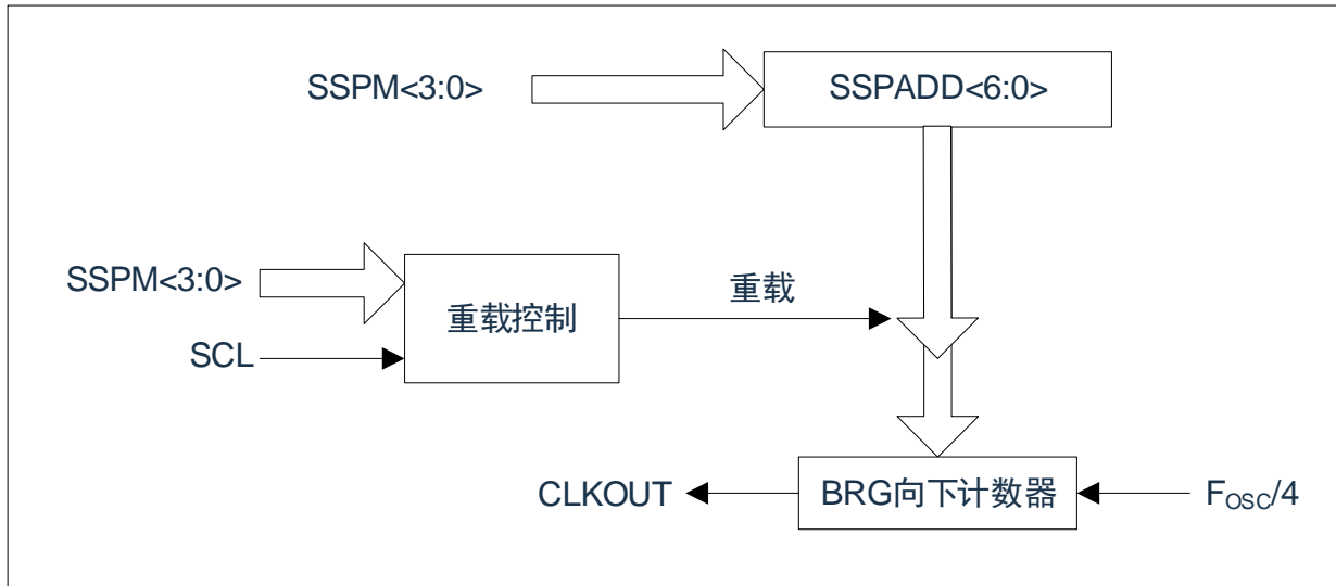
图15-8：波特率发生器框图
