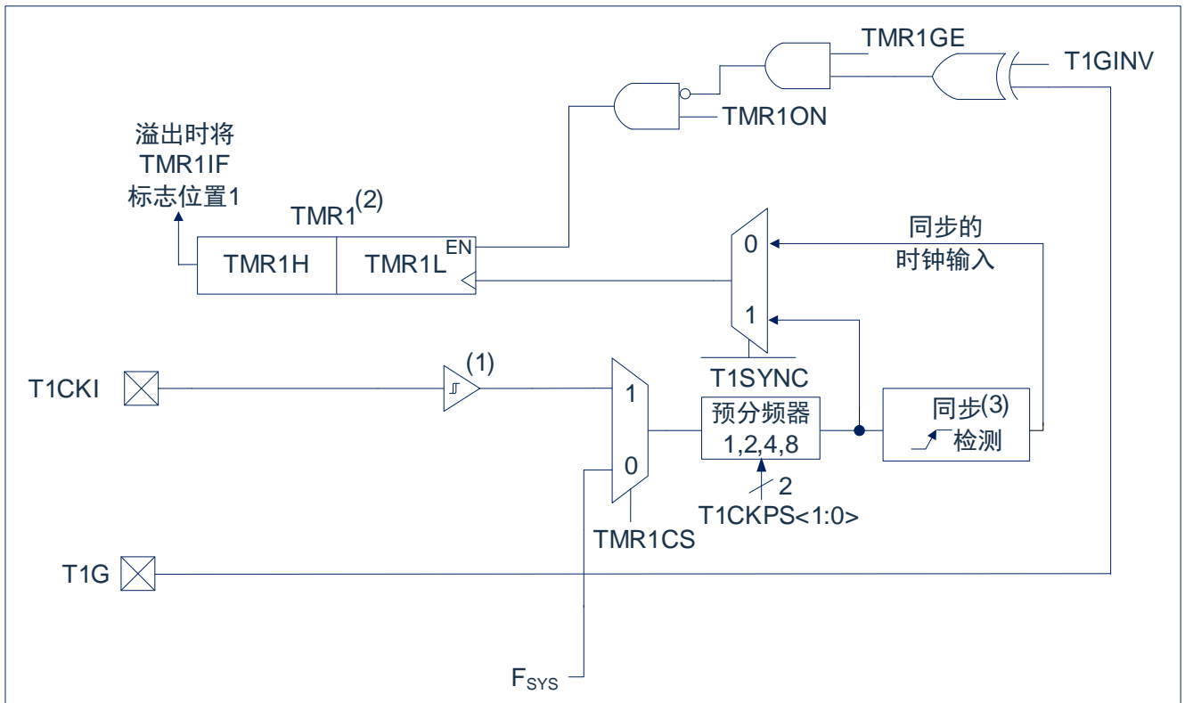
图9-1: TIMER1结构图
