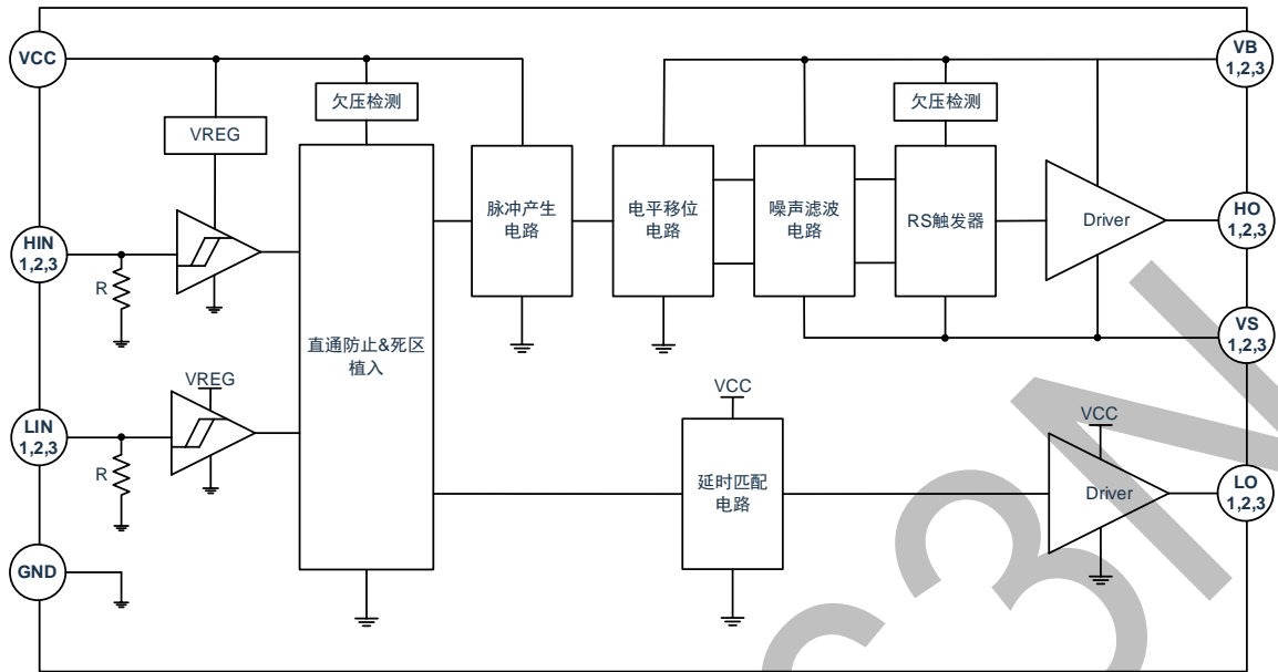
图 3-1 CMS6163N 内部框图
