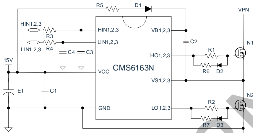
图 7-1 CMS6163N 典型应用电路
