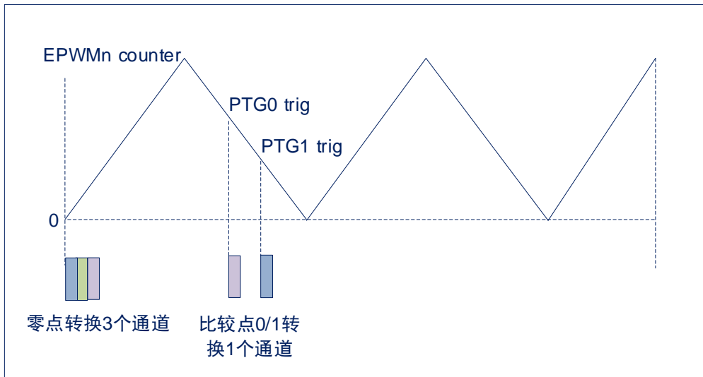
图16-2: EPWM触发启动ADC设置
