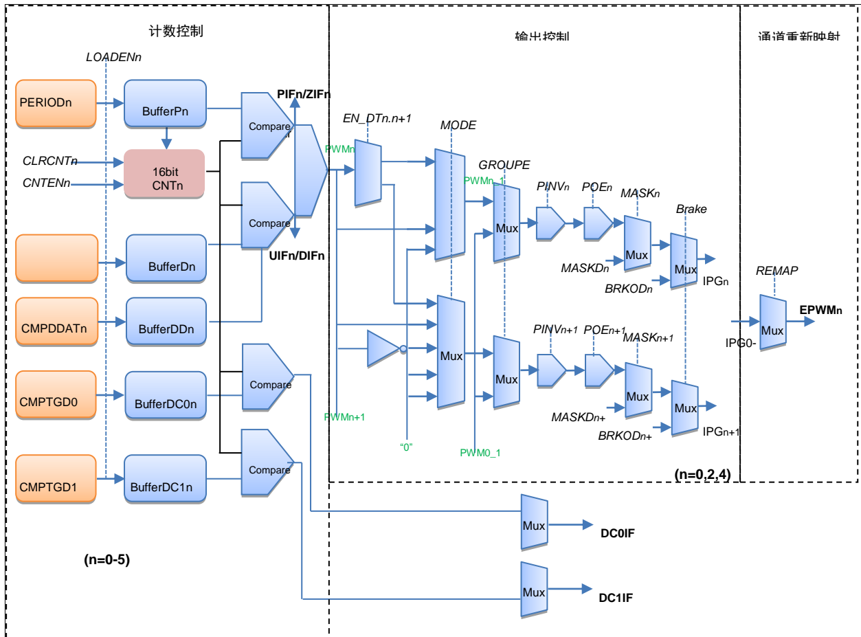
图12-1: IPGn的信号为EPWMn重映射前的信号。
