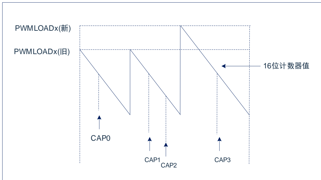
图 11-2: CAP0-CAP3 通道捕捉操作
