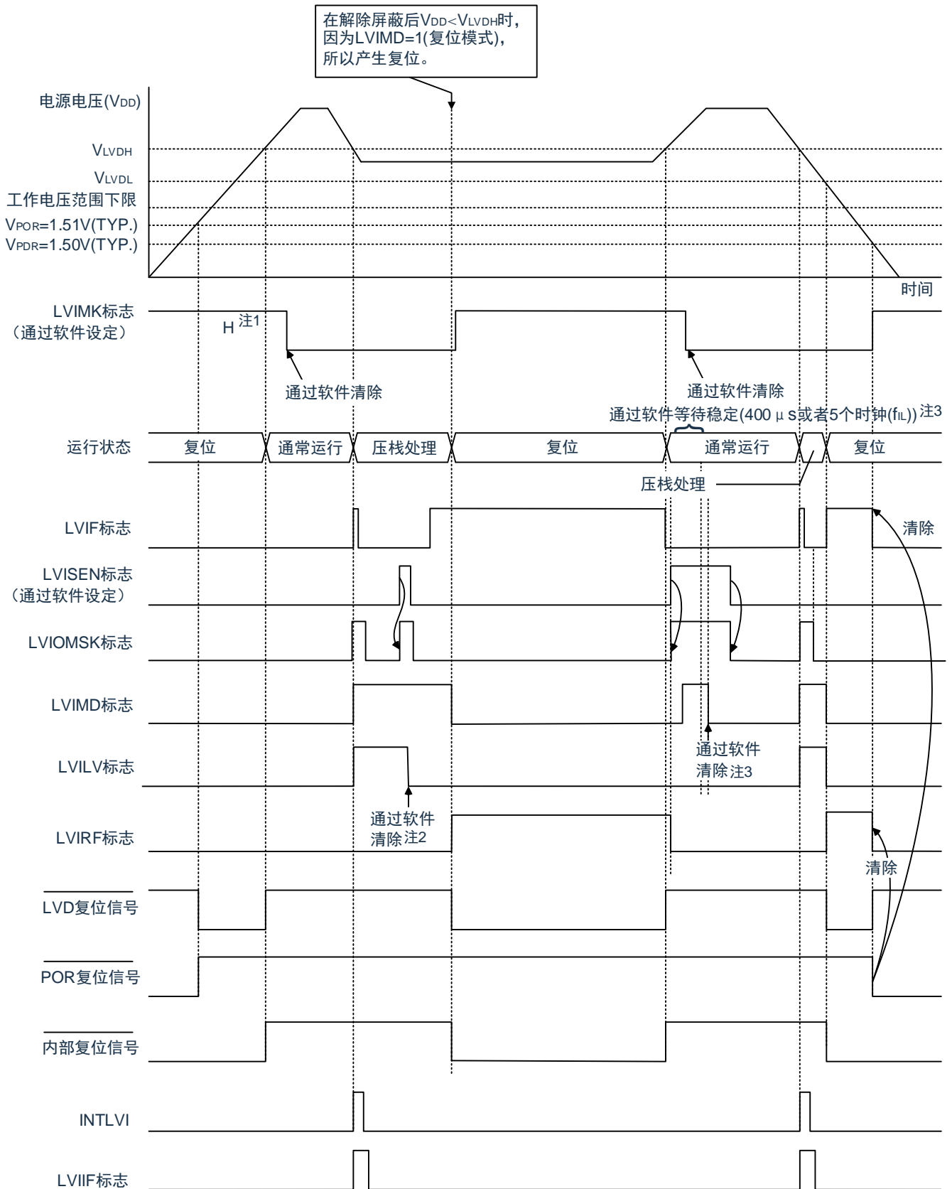
图 24-4: 中断&复位信号的产生时序 (选项字节的 LVIMDS1、LVIMDS0=1、0) (2/2)
