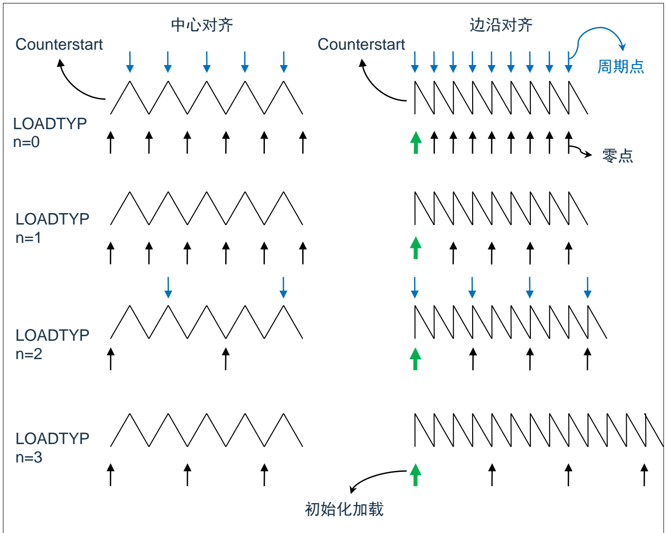
图12-2: PWM周期/占空比加载更新框图
