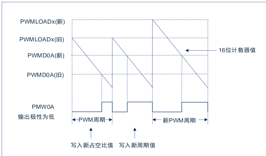
图 11-1: PWM 时序图
