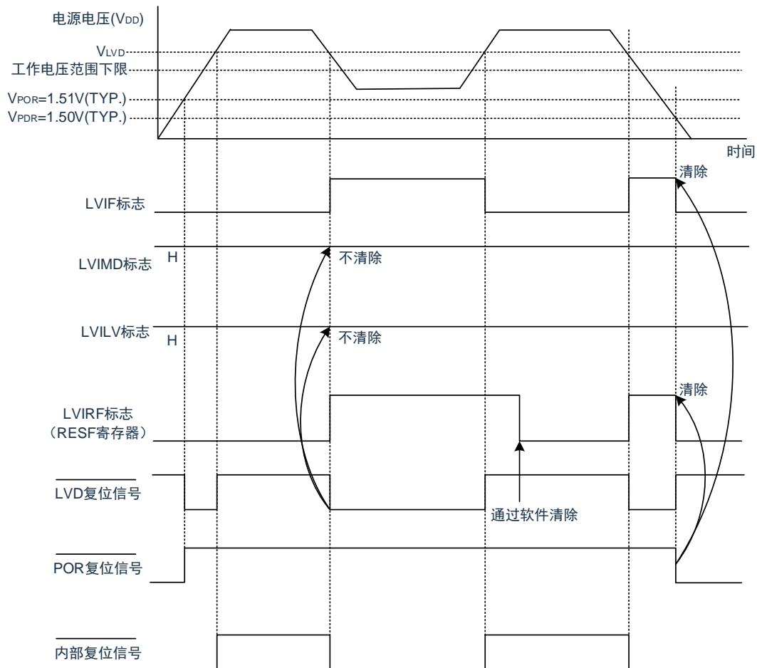
图24-2：内部复位信号的产生时序（选项字节的LVIMDS1、LVIMDS0=1、1）
