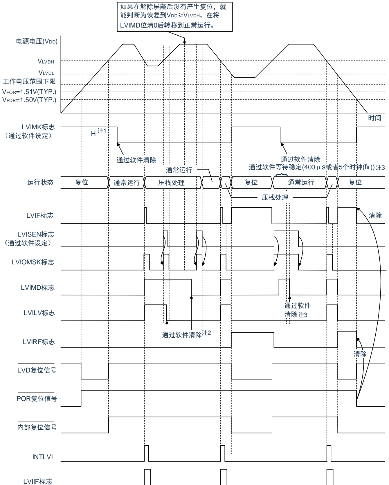
图 24-4: 复位&中断信号的产生时序 (选项字节的 LVIMDS1、LVIMDS0=1、0) (1/2)
