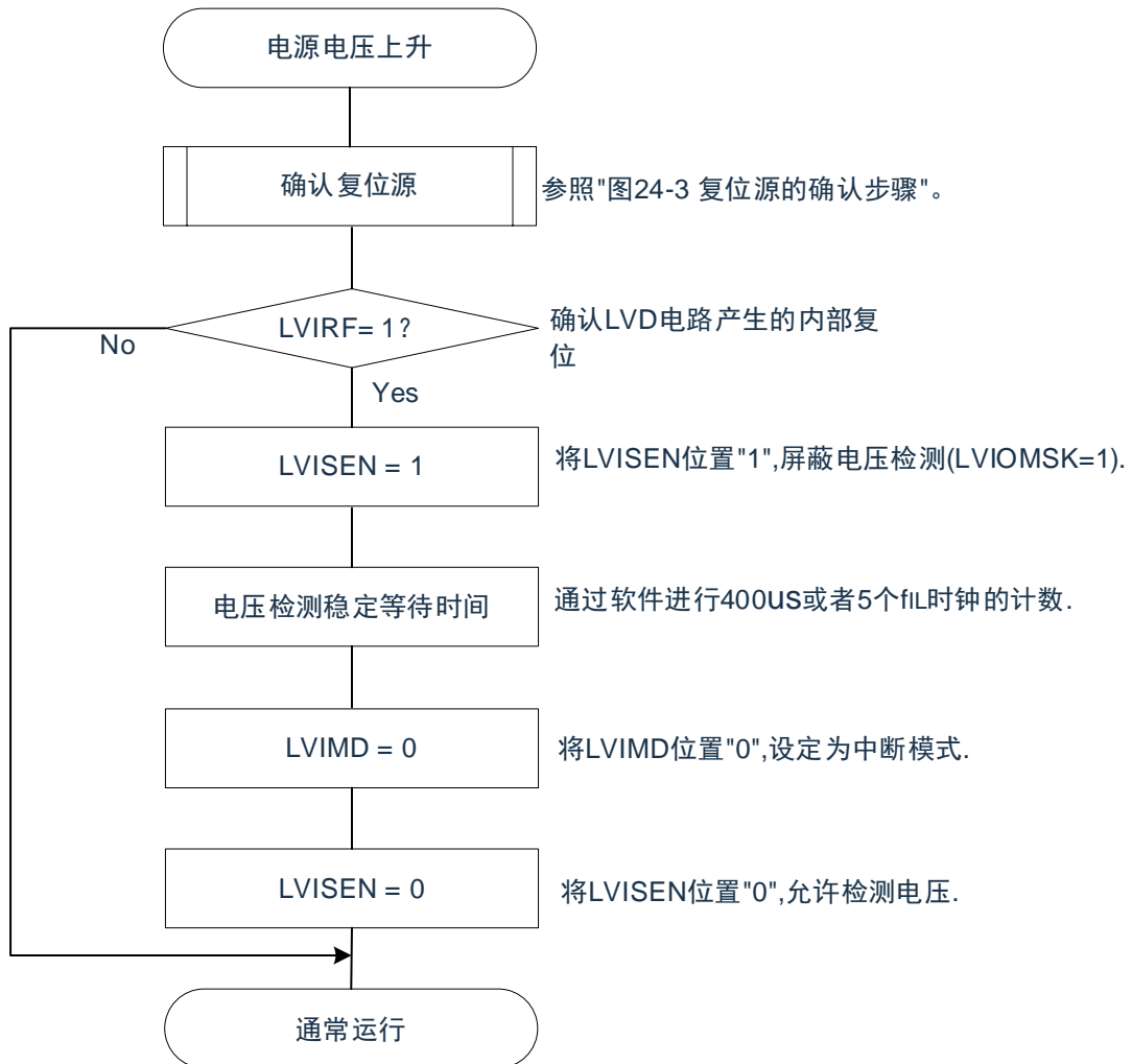
图24-6：中断&复位模式的初始设定步骤
