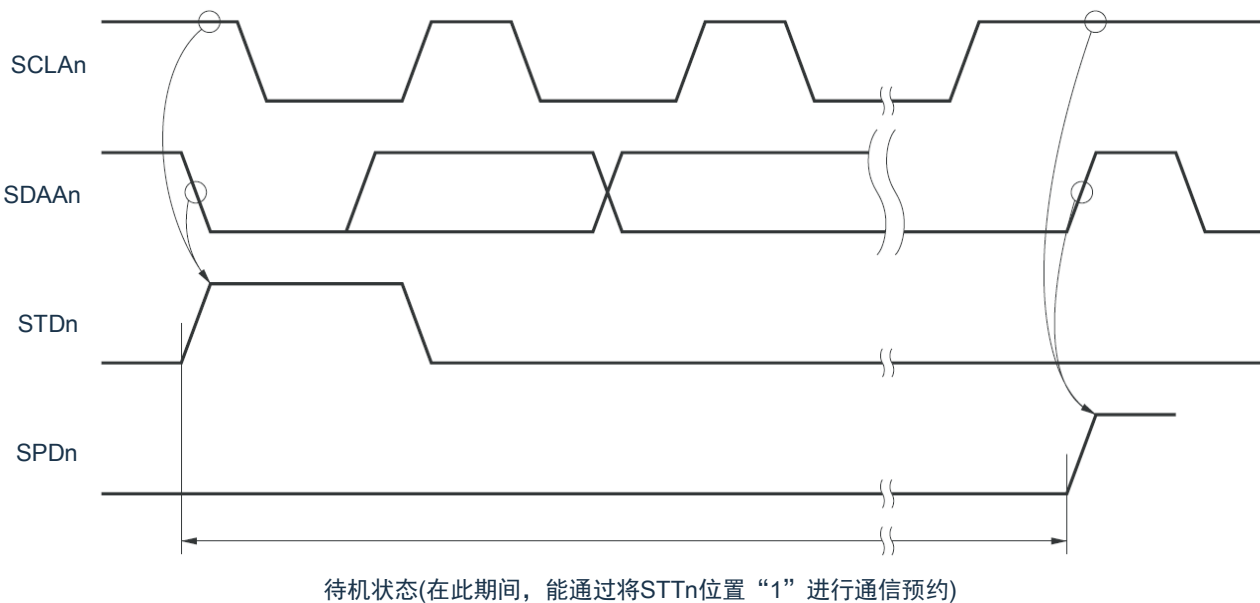
图14-25 通信预约的接受时序
