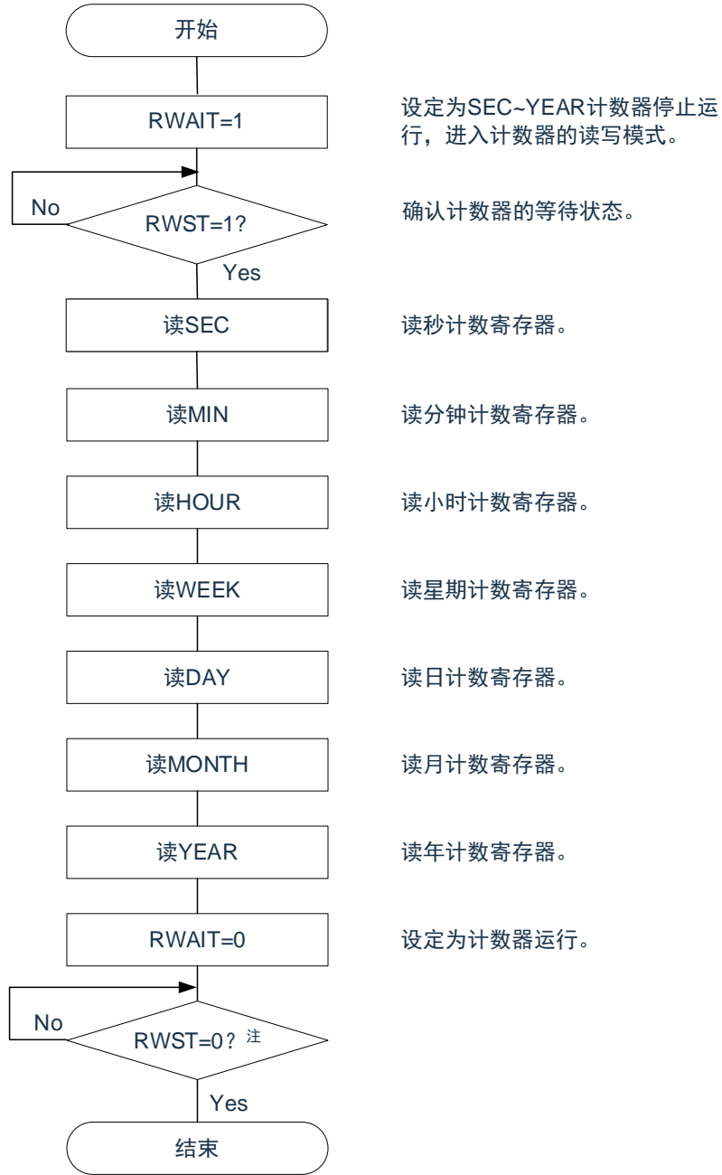
图7-19 实时时钟计数器的读操作步骤
