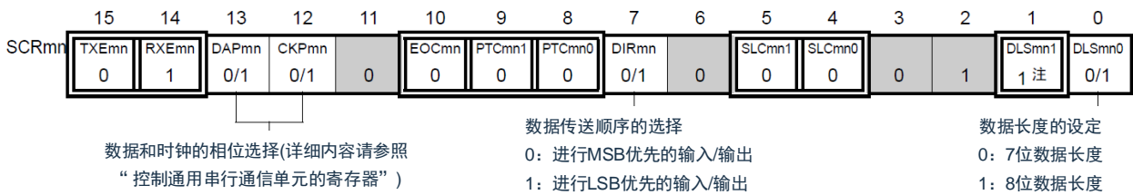
(b) 串行通信运行设定寄存器mn(SCRmn)
