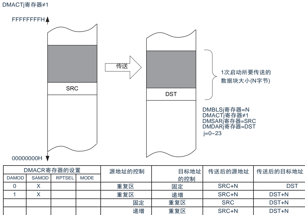
图16-18 重复模式的数据传送
