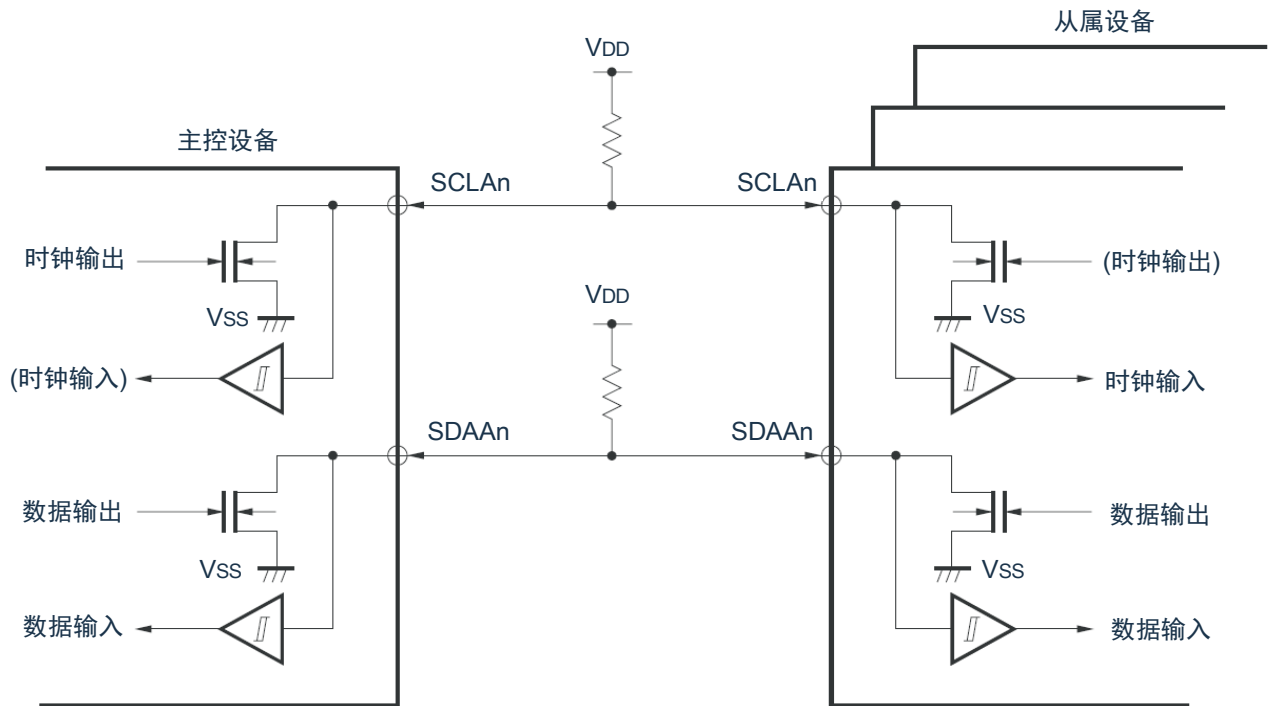
图14-12 引脚结构图
