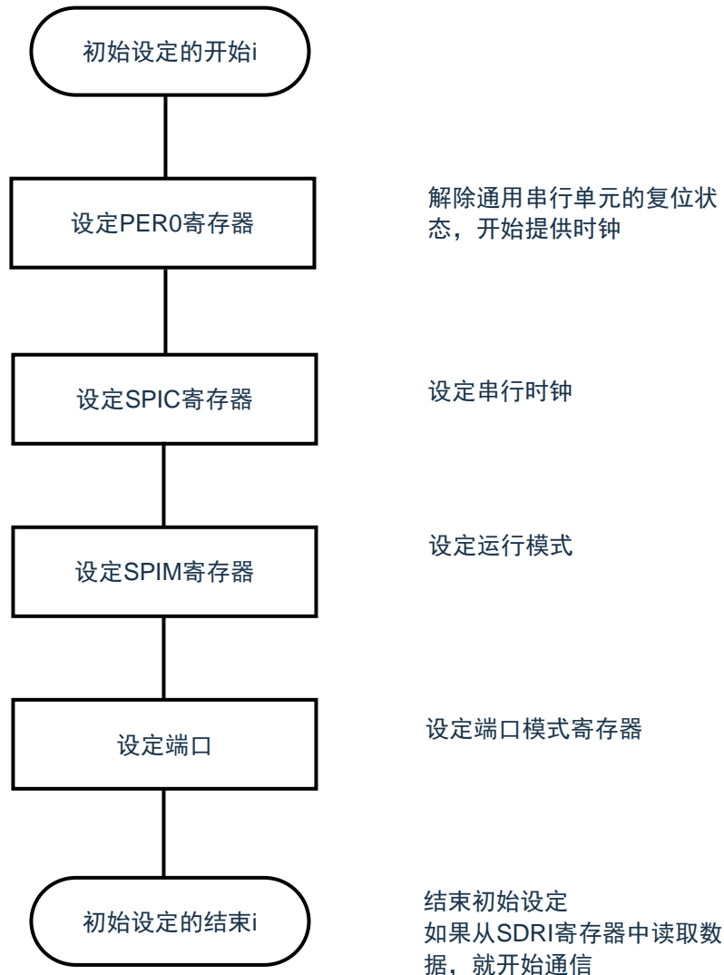
图13-10 主控接收的初始设置步骤
