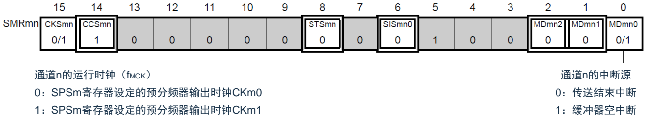
图12-72 从属选择输入功能（SSPI00）从属发送时的寄存器设定内容例子(1/2)
