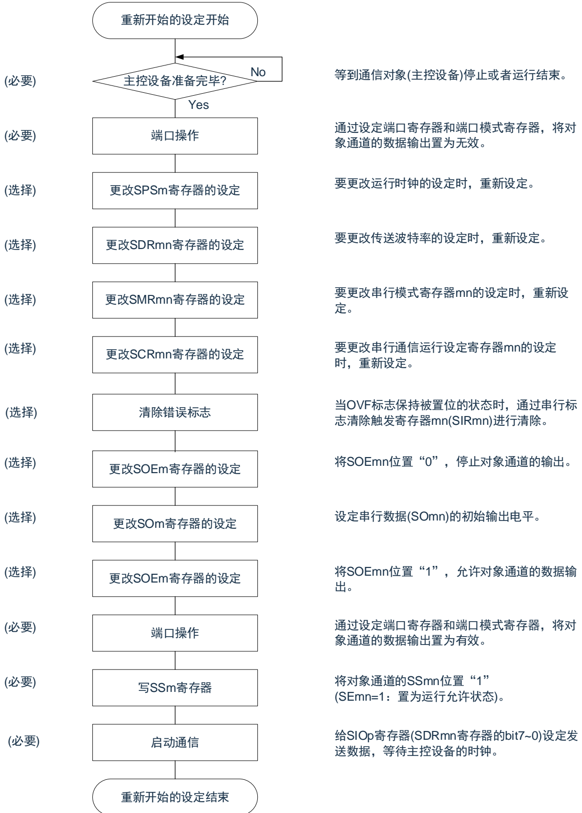
图12-50 重新开始从属发送的设定步骤
