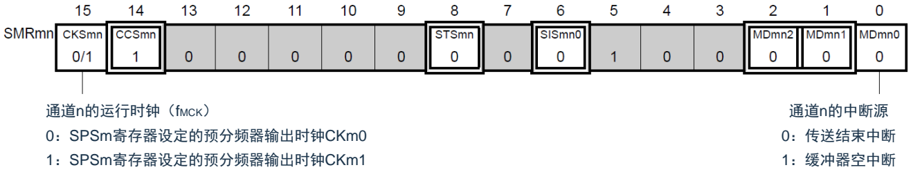
图12-80 从属选择输入功能 (SSPI00) 从属接收时的寄存器设定内容例子(1/2)
