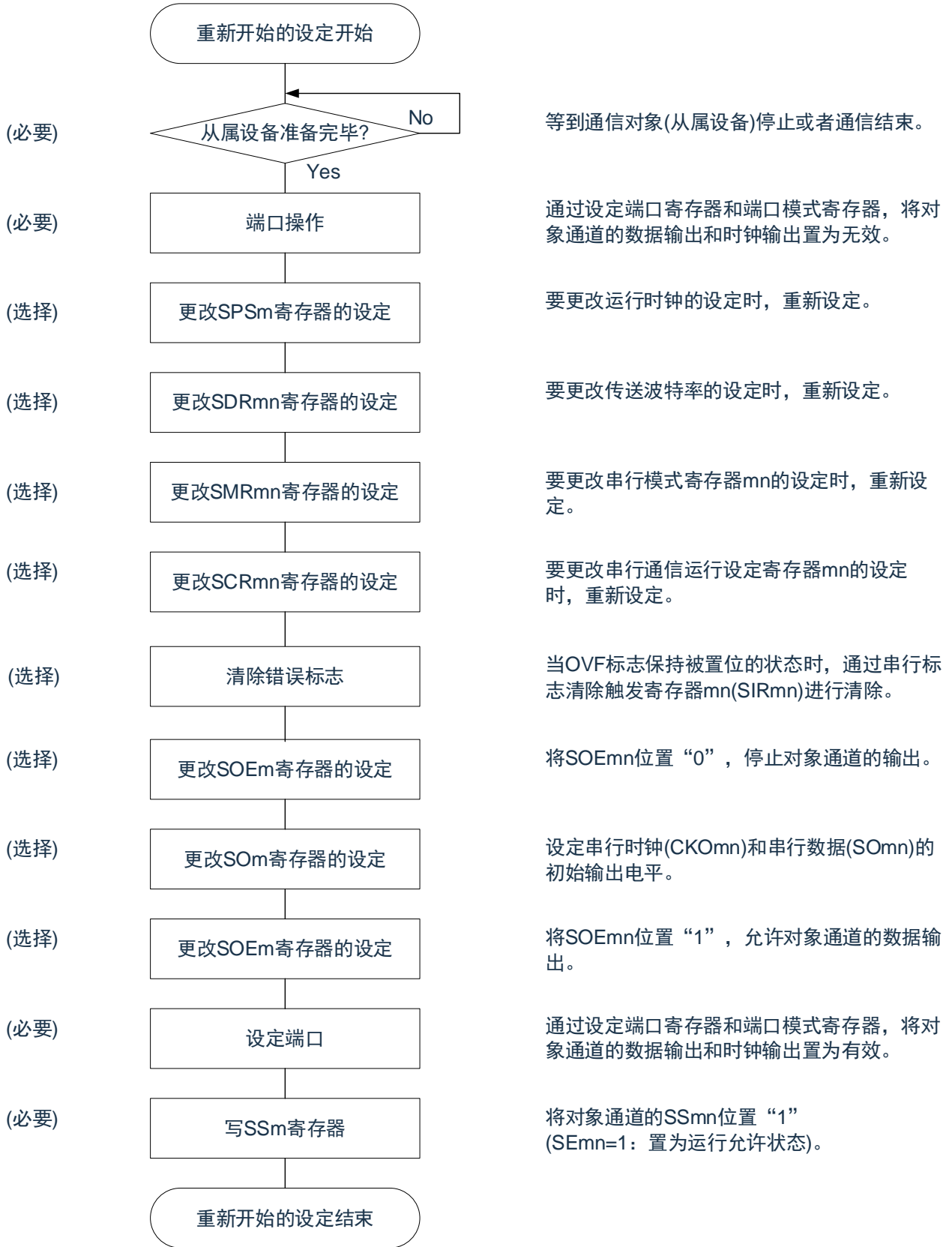
图12-42 重新开始主控发送和接收的设定步骤
