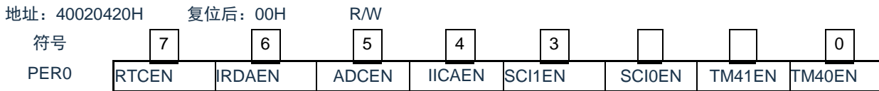
图15-2 外围允许寄存器0 (PER0) 的格式
