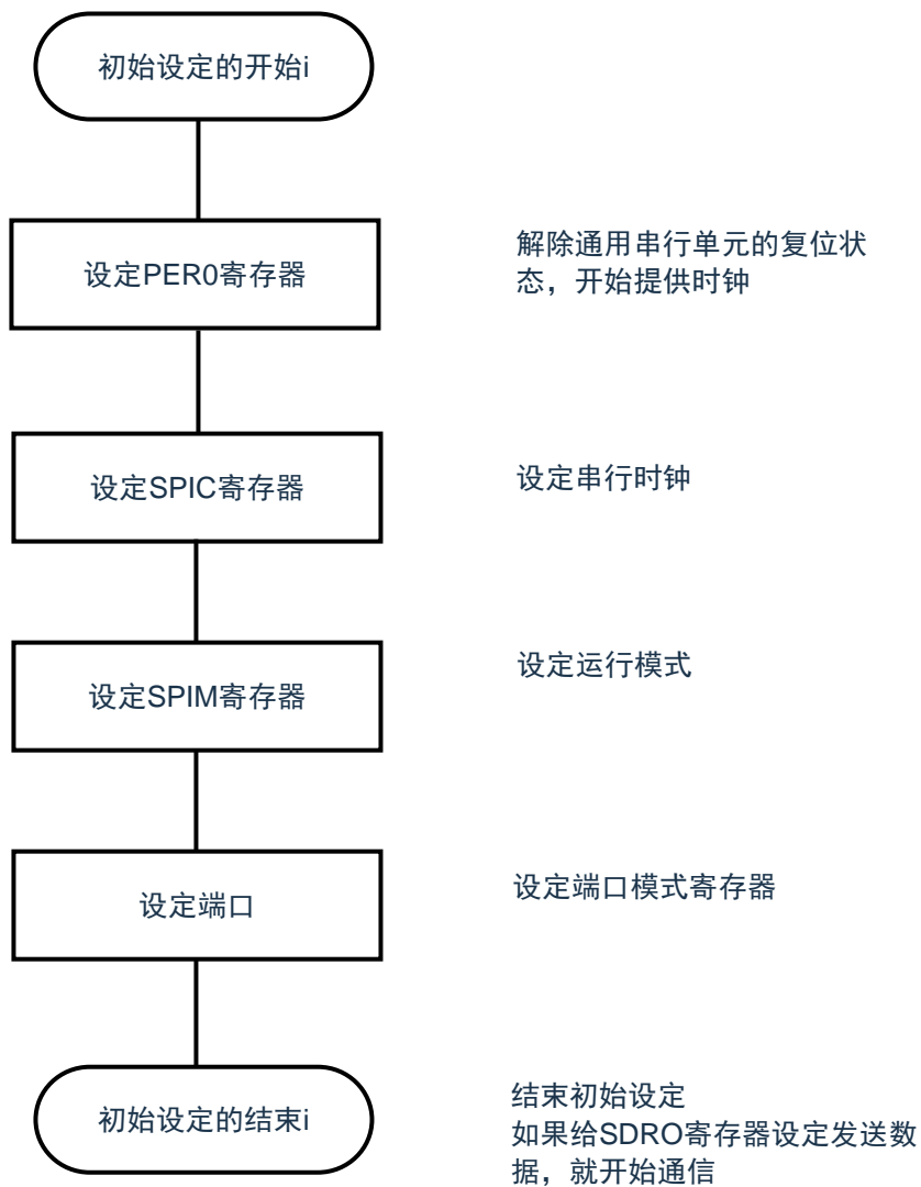
图13-6 主控发送/接收的初始设置步骤
