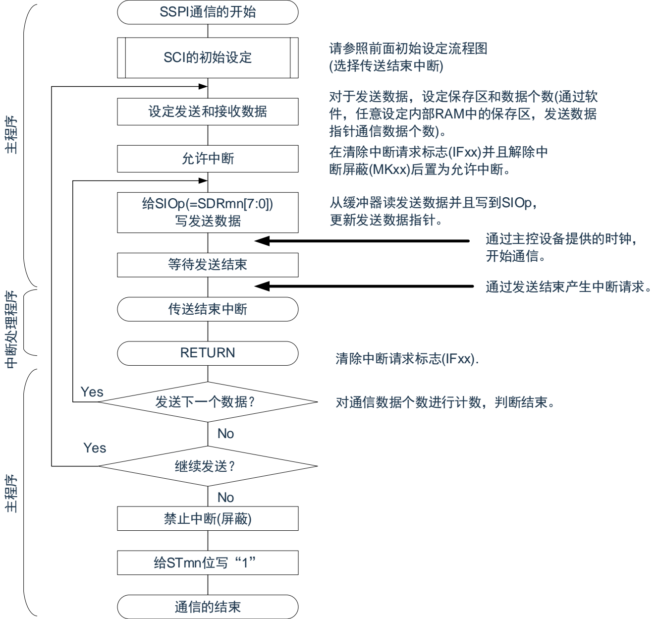
图12-52 从属发送（单次发送模式）的流程图
