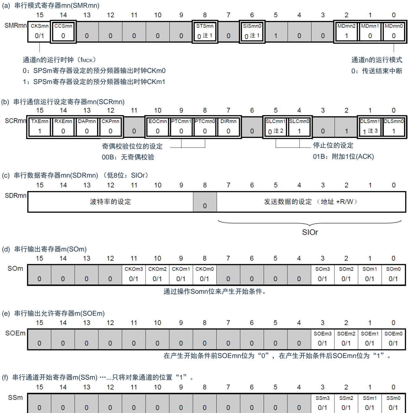
图12-118 简易I 2 C (IIC00、IIC01、IIC10、IIC11、IIC20、IIC21) 地址段发送时的寄存器设定内容例子
