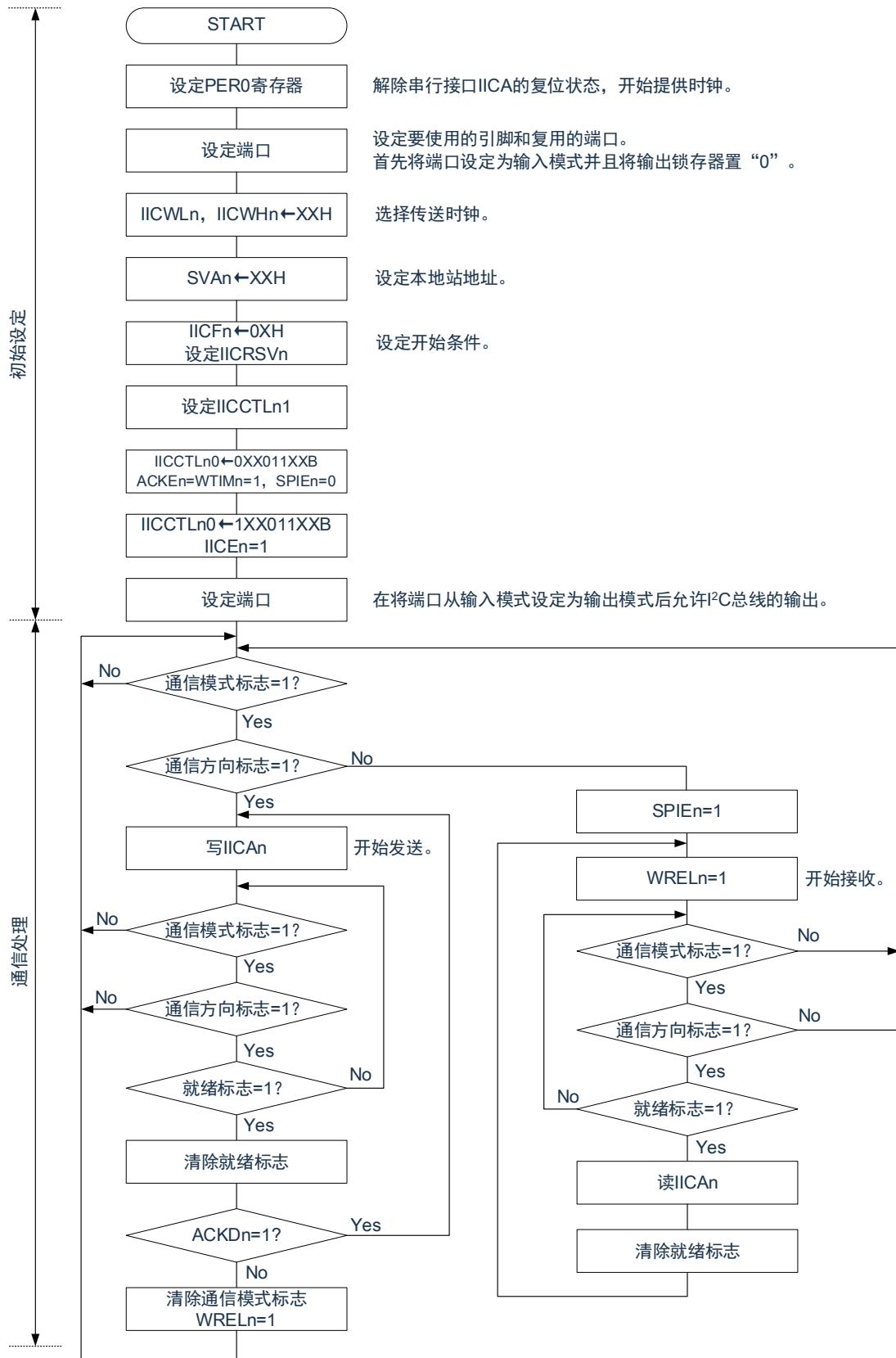
图14-29 从属运行步骤(1)
