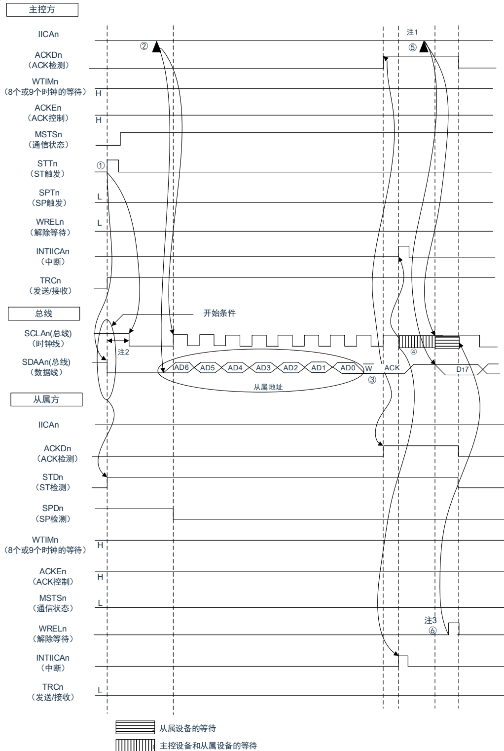
图14-31 主控设备 从属设备的通信例子 (主控设备：选择9个时钟的等待，从属设备：选择9个时钟的等待) (1/4)
