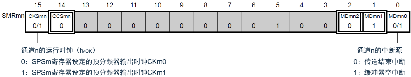
图12-96 UART (UART0~UART2) 的UART发送时的寄存器设定内容例子(1/2)
