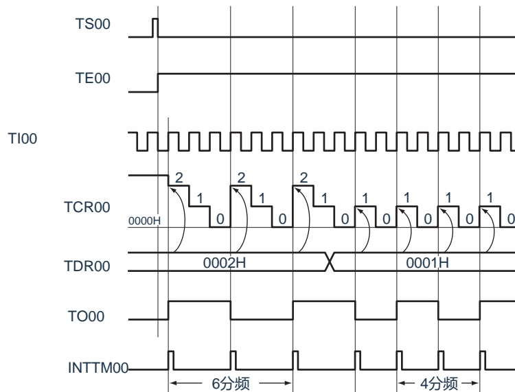
图5-49 作为分频器运行的基本时序例子 (MD000=1)
