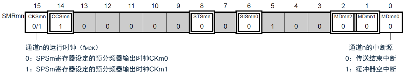
(a) 串行模式寄存器mn(SMRmn)
