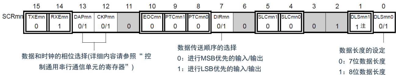
(b) 串行通信运行设定寄存器mn(SCRmn)
