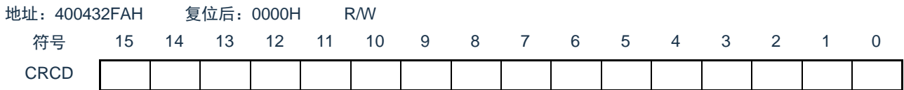
图24-5 CRC数据寄存器 (CRCD) 的格式
