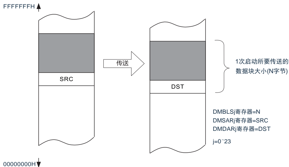
图16-15 正常模式的数据传送
