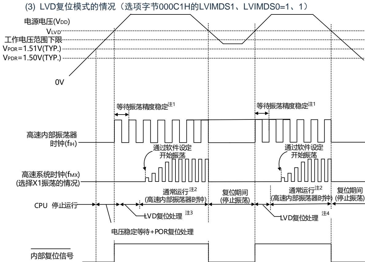
图22-2 上电复位电路和电压检测电路的内部复位信号的产生时序(3/3)
