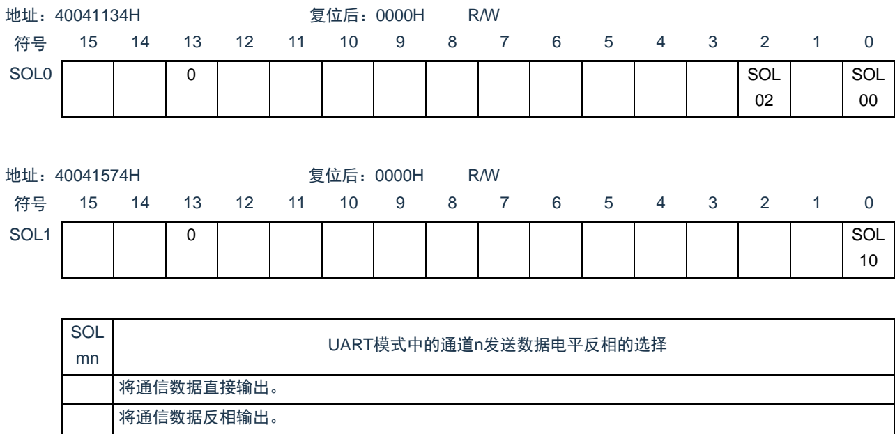
图12-17 串行输出电平寄存器m (SOLm) 的格式
