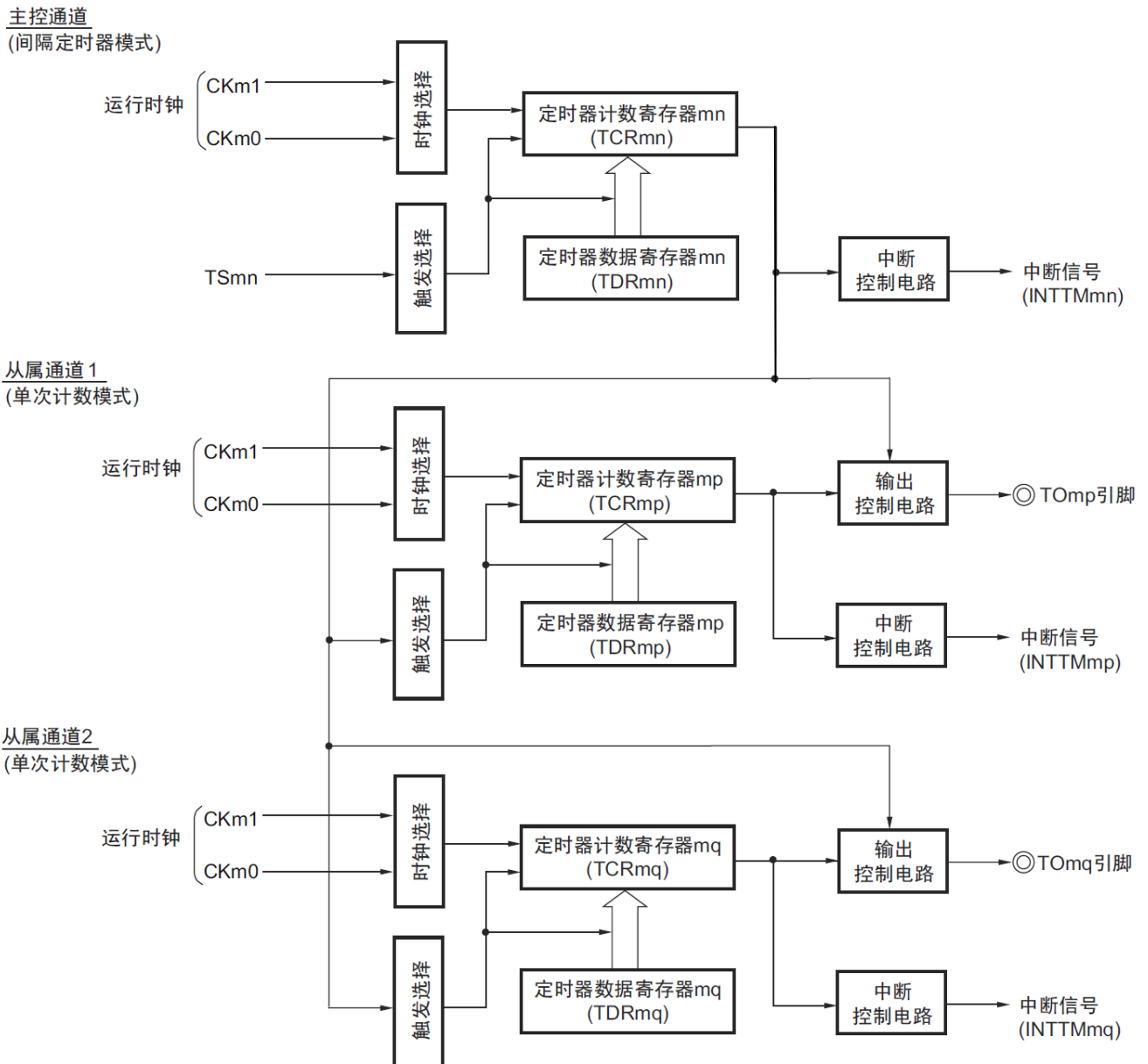
图5-73 作为多重PWM 输出功能运行的框图（输出2 种PWM 的情况）
