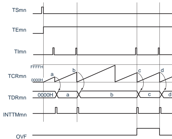
图5-52 作为输入脉冲间隔测量的运行基本时序例子 (MDmn0=0)
