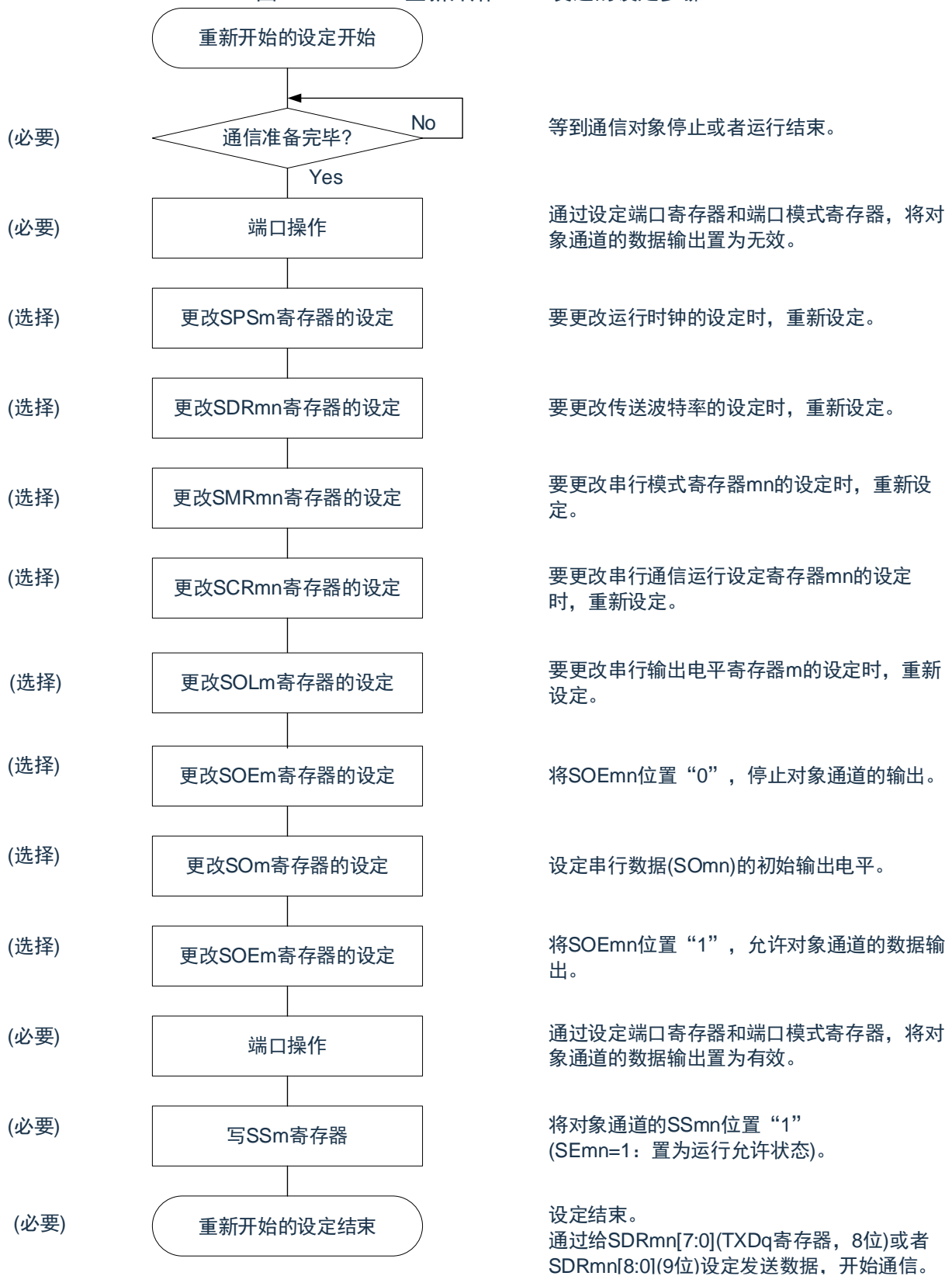
图12-99 重新开始UART发送的设定步骤
