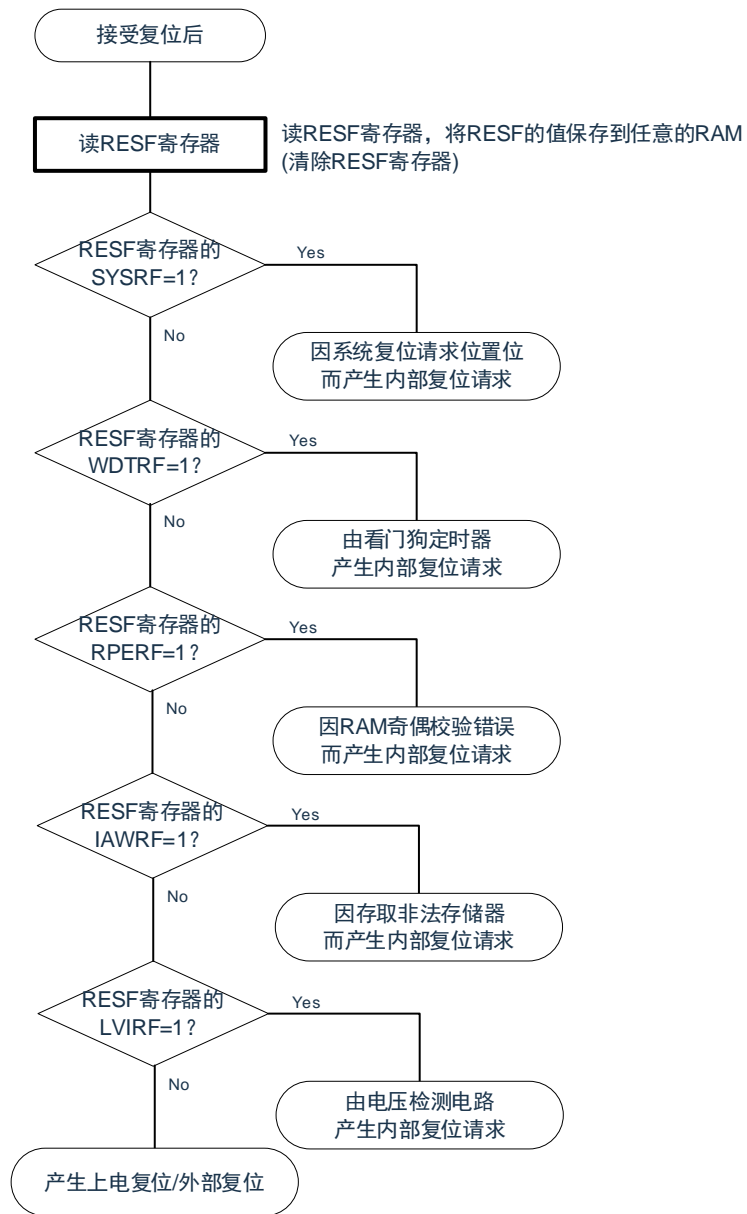
图21-5 复位源的确认步骤
