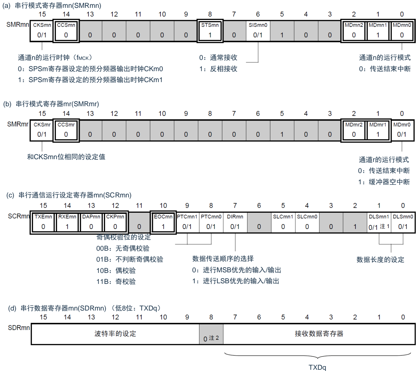
图12-104 UART (UART0~UART2) 的UART接收时的寄存器设定内容例子(1/2)
