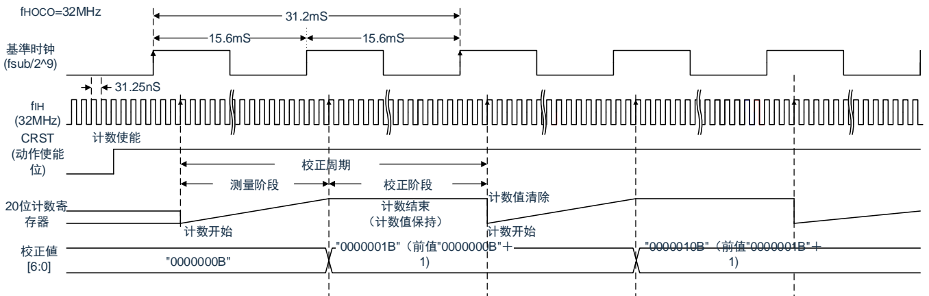
图4-20 高速内振频率校正动作时序图（详细）
