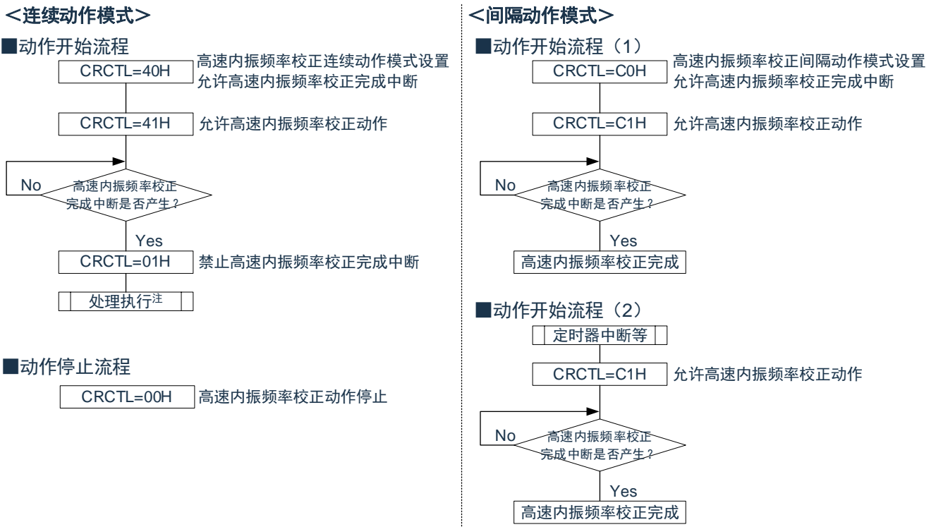
图4-23 动作模式设定流程（例）
