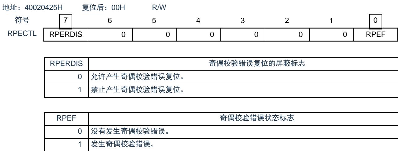
图24-7 RAM奇偶校验错误控制寄存器（RPECTL）的格式
