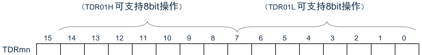
图5-5 定时器数据寄存器mn (TDRmn) (n=1、3) 的表格
