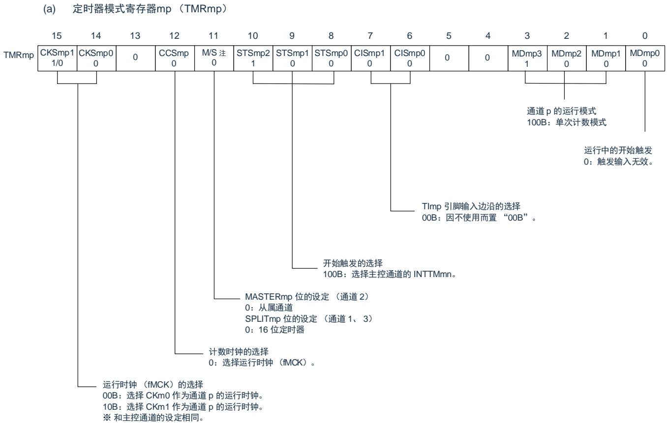
图5-64 单触发脉冲输出功能时（从属通道）的寄存器设定内容例子
