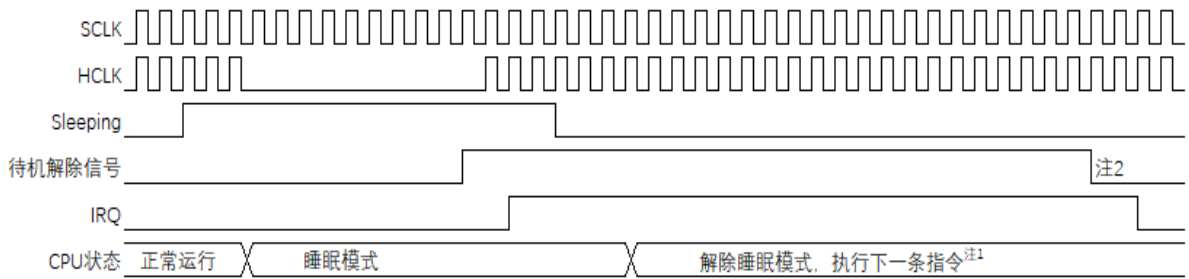
图20-1 通过中断请求解除睡眠模式
