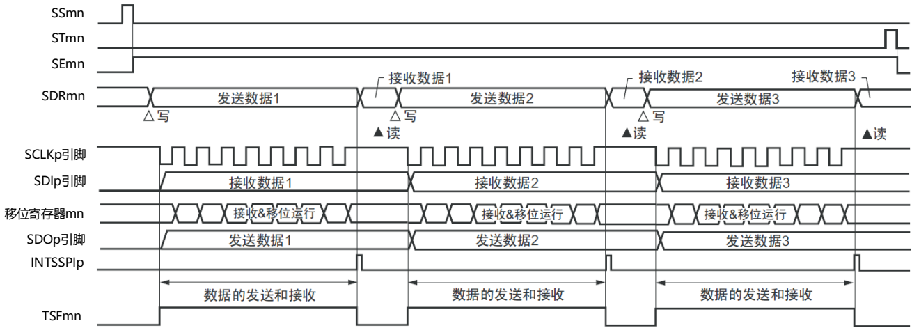
图12-43 主控发送和接收（单次发送和接收模式）的时序图（类型1：DAPmn=0、CKPmn=0）
