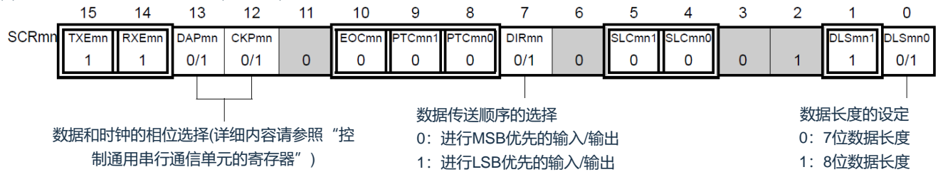
(b) 串行通信运行设定寄存器mn(SCRmn)
