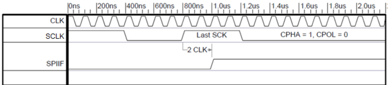
图 18-13: 中断产生
