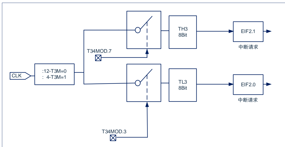
图 11-4: Timer3, 模式 3: 两个 8-位定时器
