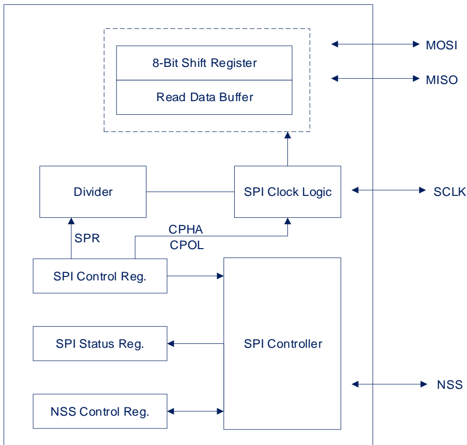
图 18-2: SPI 框图
