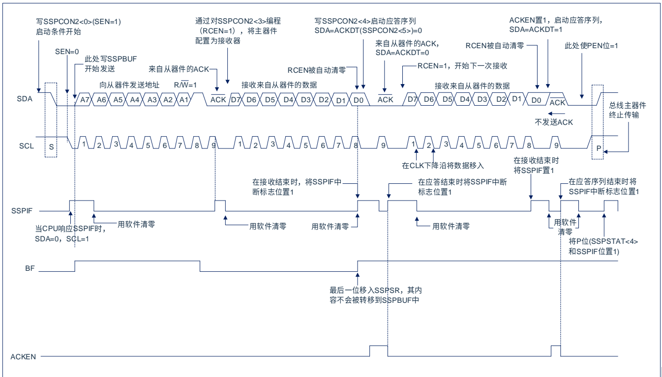
15-11: I 2 C™主控模式接收时序 (7位地址)
