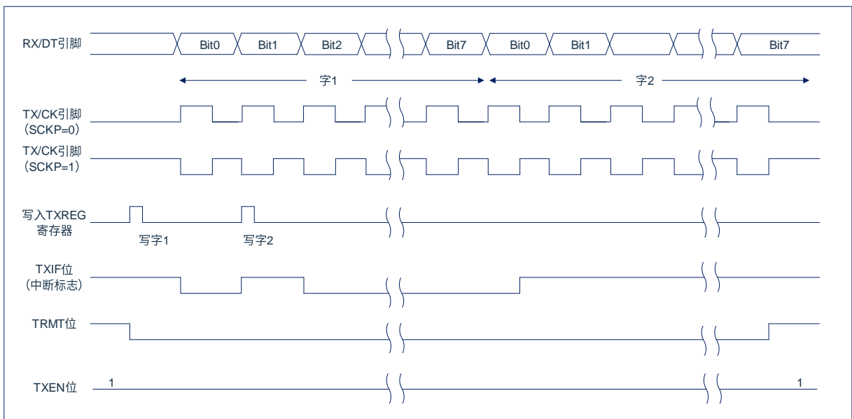
图 14-6: 同步发送
