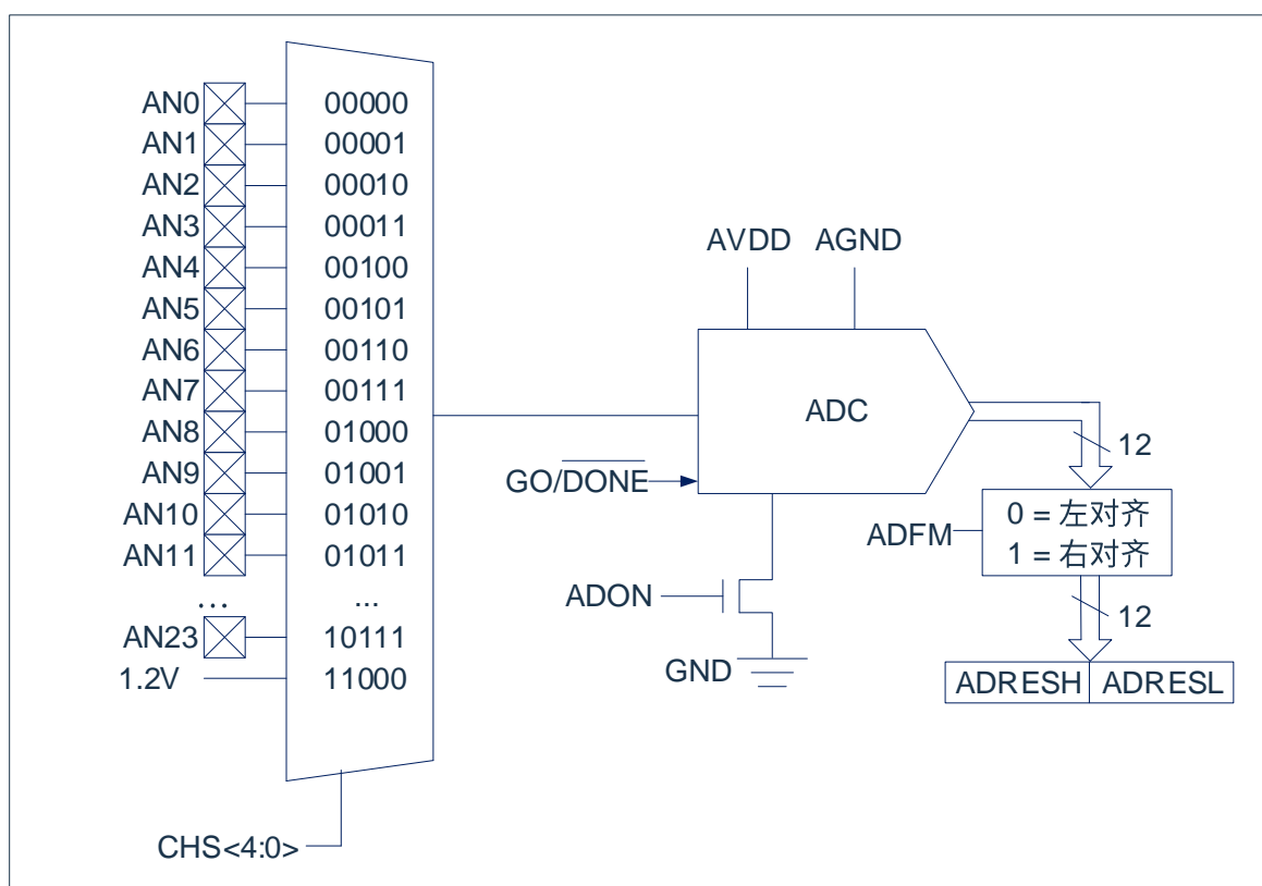
图 11-1: ADC 框图
