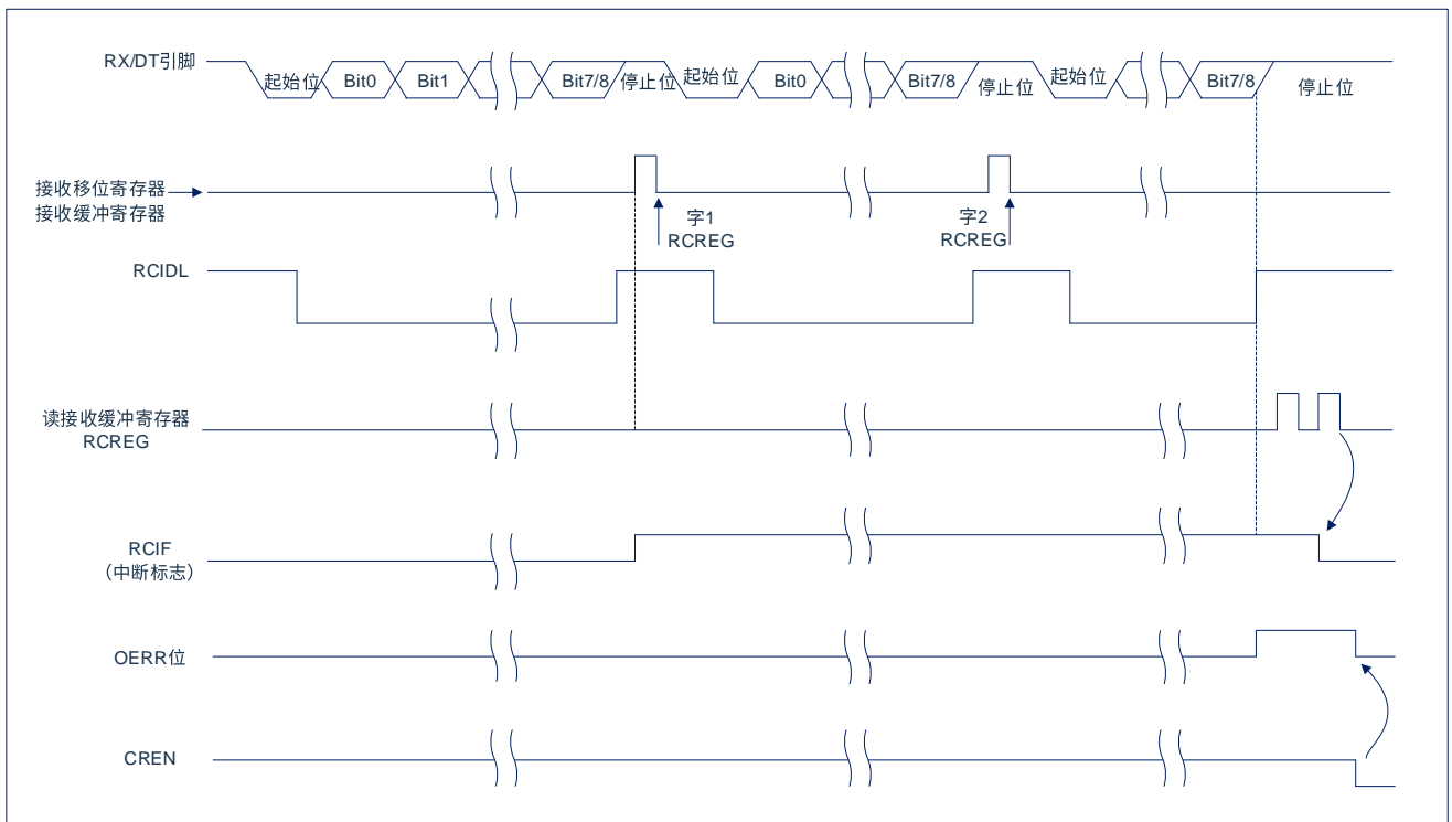
图 14-5: 异步接收
